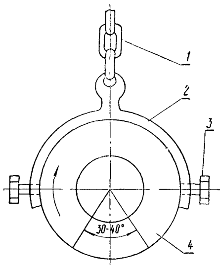
Рис. 2. Закрепление выглаживающей трубы:
