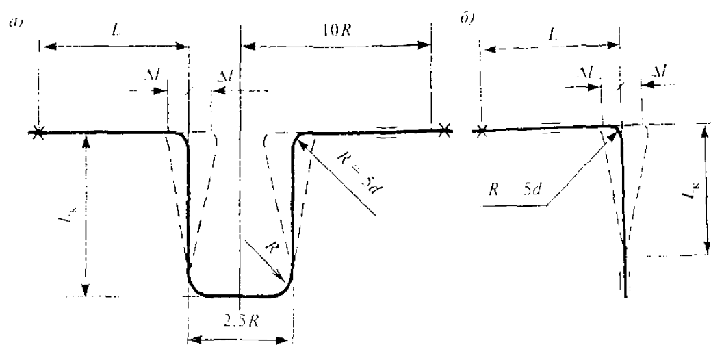
Рисунок 1 – Устройство П-образного (а) и Г-образного (б) компенсаторов
