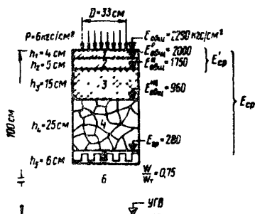
Рис. 1. Схема конструкции к примеру 1:
