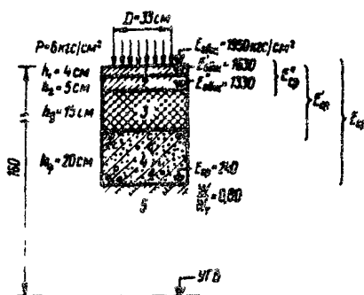
Рис.2. Схема конструкции и пример 2:
