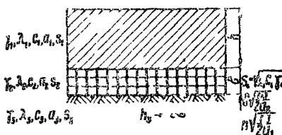
Рис. 7. Модель дорожной конструкции с теплоизолирующим слоем
