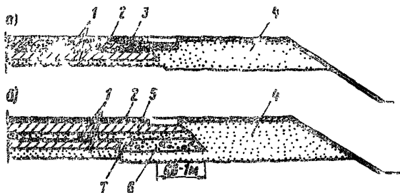
Рис. 6. Теплоизоляция, устраиваемая при усилении дорожной одежды (а) и при реконструкции дорог с утратившим и усилением дорожной одежды (б): 1-старая дорожная одежда; 2-новое покрытие; 3-легкий бетон; 4-новый дренажный слой; 5-основание; 6-укрепление основания под утратившим; 7-теплоизоляция
