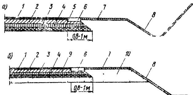
Рис.1. Конструкции с теплоизолирующим слоем из пенопласта, предотвращающим промерзание земляного полотна (а) и уменьшающим глубину промерзания земляного полотна (б):
