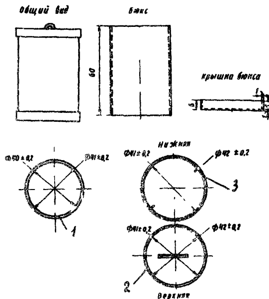
Рис.1. Бюкс для грунта: 1-бюкс; 2-верхняя крышка с дужкой; 3-нижняя крышка
