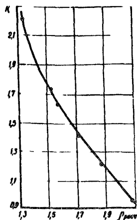
Рис.10. Градуировочный график гамма-плотвмера ПГП-2 с приставкой
