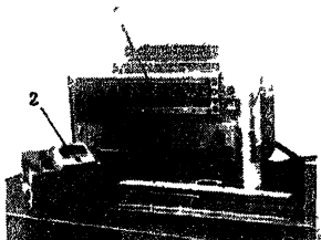
Рис.2. Комплект аппаратуры для измерений объемной массы грунта : 1-ШГП; 2-радиомер СРП-68-01; 3-сцинтилляционный детектор; 4-электронно-счетный частотомер ЧЗ-12
