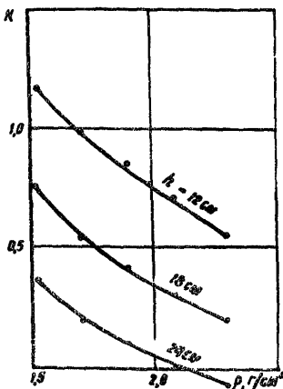
Рис.3. Градуировочные кривые гамма-плотномера со сцинтилляционным детектором для глубины зондирования 24, 18, 12 см
