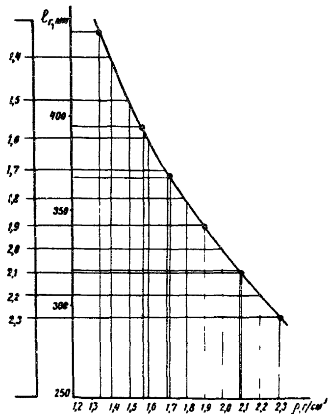
Рис.8. Построение шкалы плотностей по переменной базе для N_{гр} = 0,5 \text{ N/kg}
