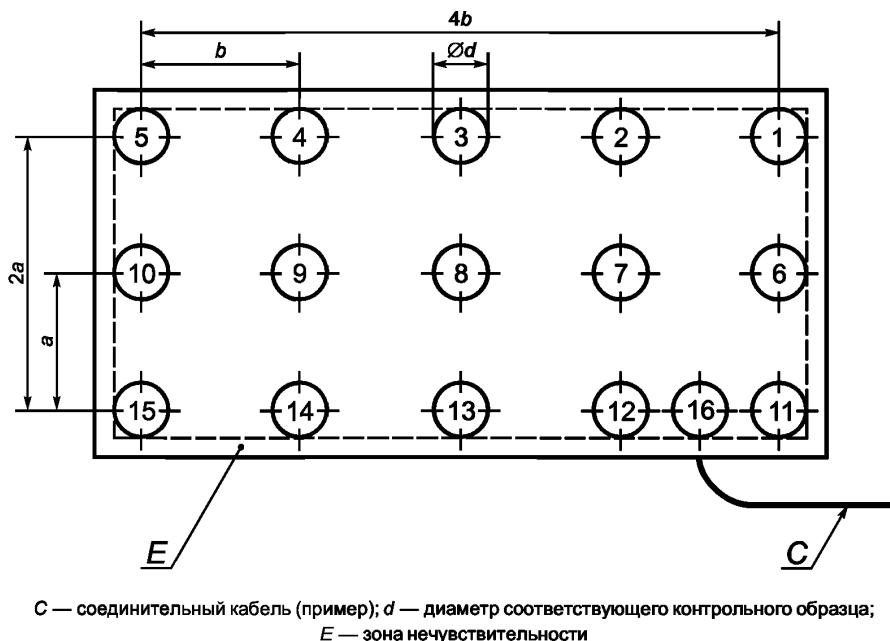
Рисунок 3 — Места испытаний эффективной чувствительности области одиночного датчика
