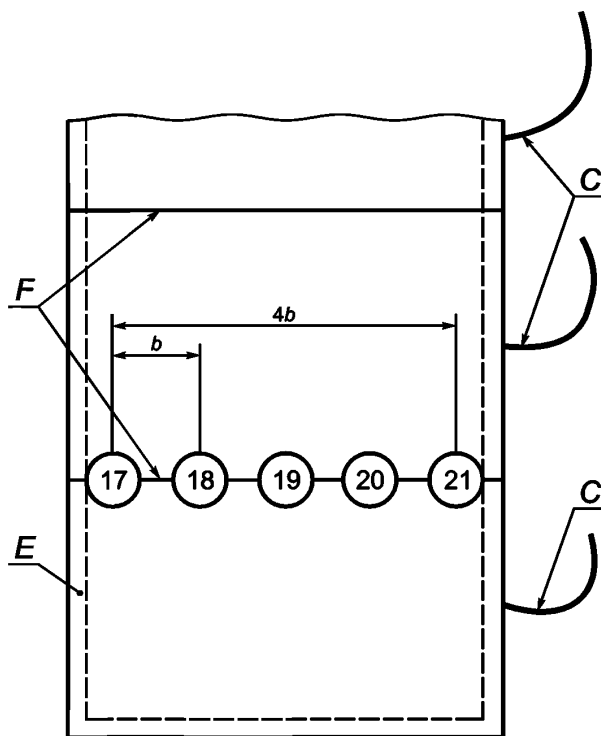
Рисунок 4 — Места испытаний на сочленениях между датчиками
