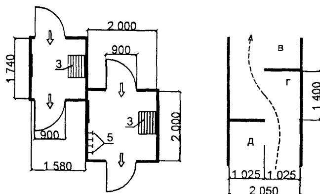
Спортивные индивидуальные кабины для переодевания
