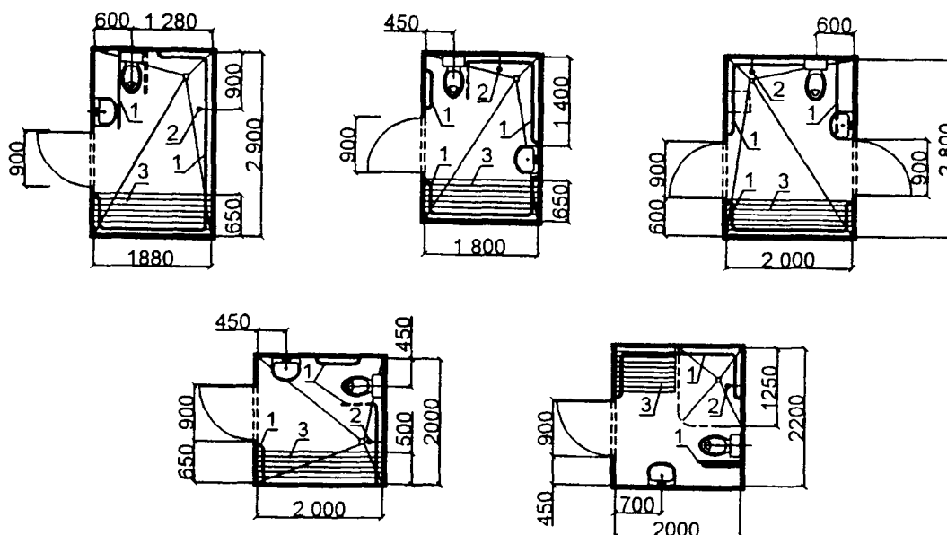
Индивидуальные душевые кабины
