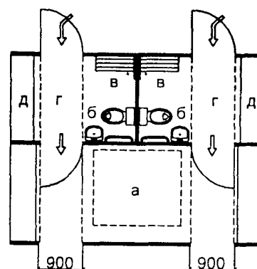
Блок проходных душевых
