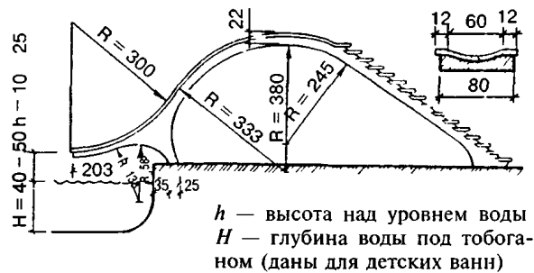
Тобоган железобетонный Разрез по желобу
