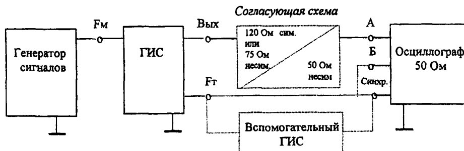
Рисунок 6 Схема проверки вводимого фазового дрожания
