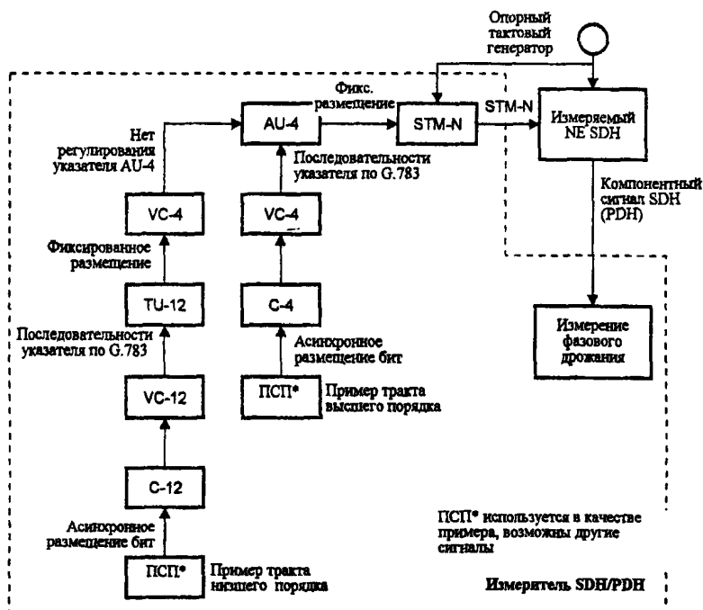
Рисунок Б.1 - Функциональная структурная схема генерирования испытательных последовательностей указателя
