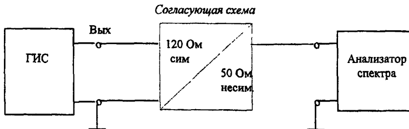
Рисунок 5 Схема проверки собственного фазового дрожания
