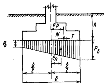
Рис. 1. Эпюра предельного давления под подошвой фундамента
