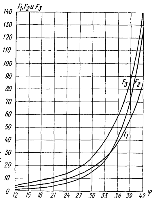
Рис. 2. Графики для коэффициентов в формулах (4) и (5)
