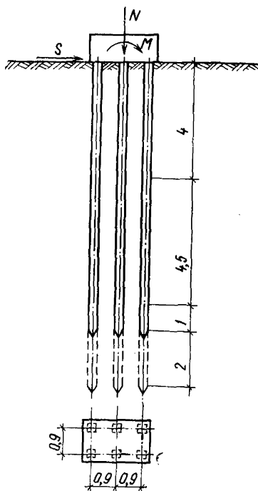
Рис. 8. Расчетная схема свайного фундамента
