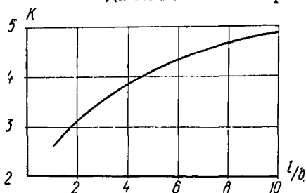
Рис. 7. Зависимость коэффициента K от отношения длины фундамента к его ширине
