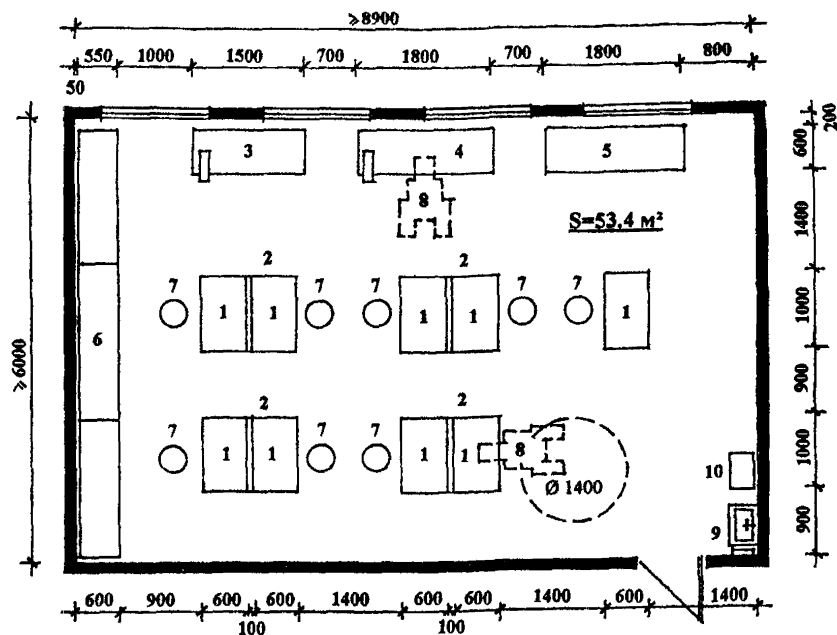
Экспликация оборудования
