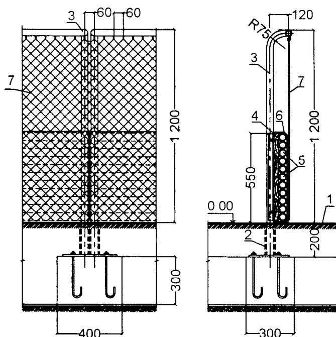
ОГРАЖДЕНИЕ СЕКТОРА ДЛЯ ПРИЗЕМЛЕНИЯ ЯДРА (ПРИМЕРНЫЙ ВАРИАНТ)
