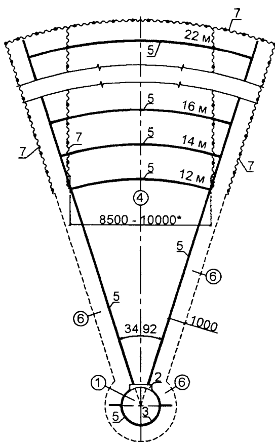
ПЛОЩАДКА ДЛЯ ВЫПОЛНЕНИЯ ТОЛЧКА
