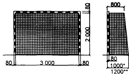
СХЕМА ВОРОТ
