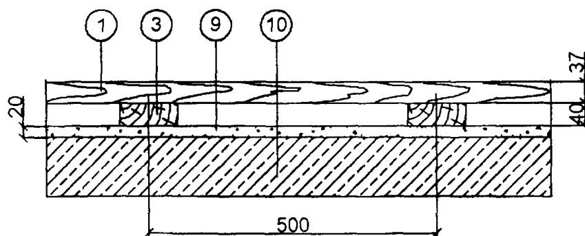
Схема 2. Дощатый пол по лагам на перекрытии
