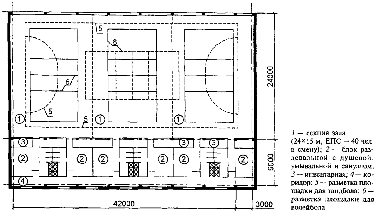
ПРИМЕР ПЛАНИРОВКИ СЕКЦИОННОГО ЗАЛА 45×24 м
