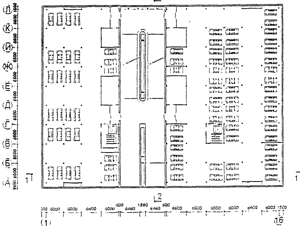
ПЛАН ЭТАЖА на отм. 0.00
