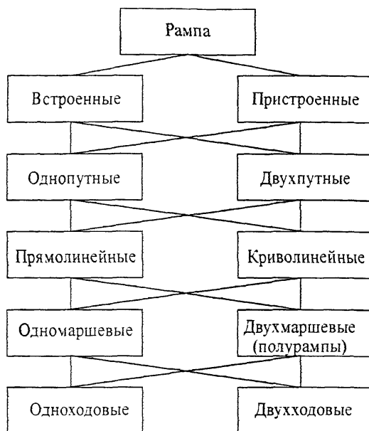
Рис 6. Классификация рамп.
