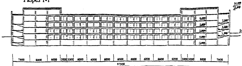
Разрез 1-1
