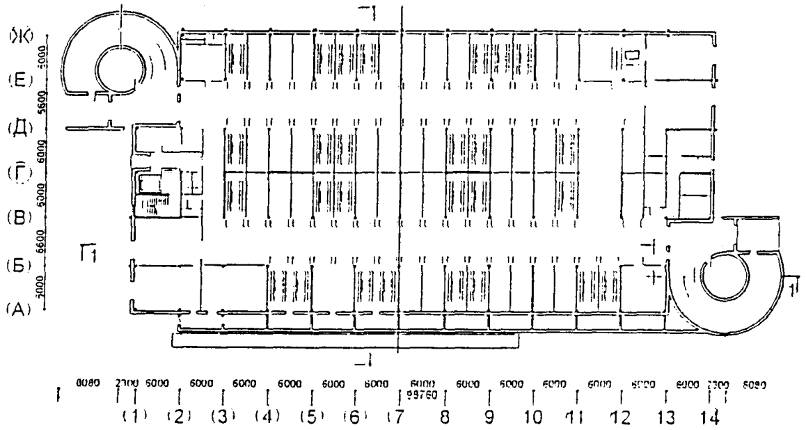
ПЛАН ПЕРВОГО ЭТАЖА
