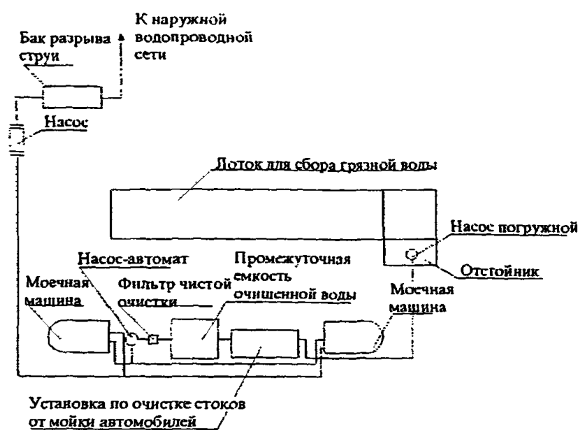
Рис. 13. Технологическая схема ручной мойки.
