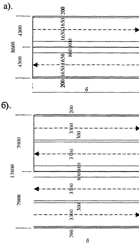
Рис. 10. Минимальная горизонтальная проекция прямолинейной полурампы (аппарели) Уклон 10%.
