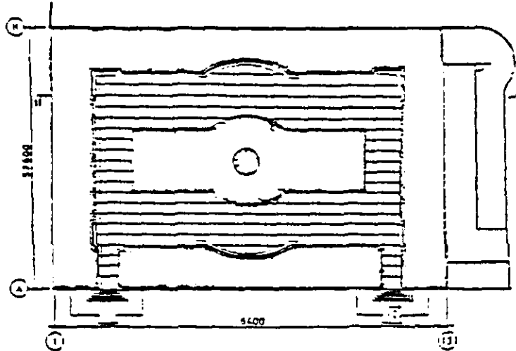
ПЛАН НА ОТМ. -2.30
