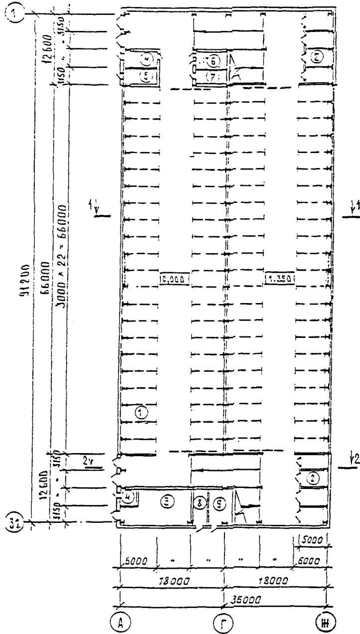
План 1 этажа
