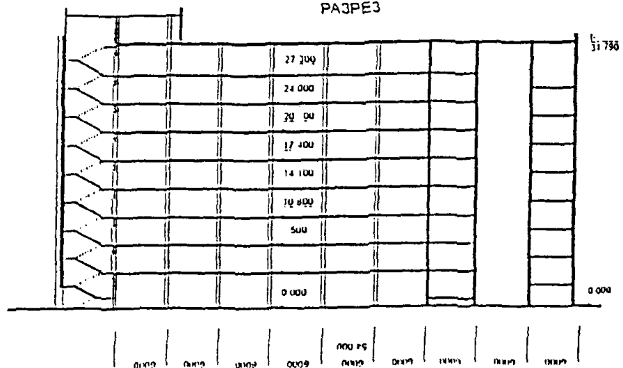
РАЗРЕЗ
