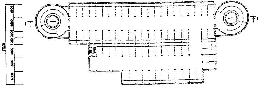
План первого этажа
