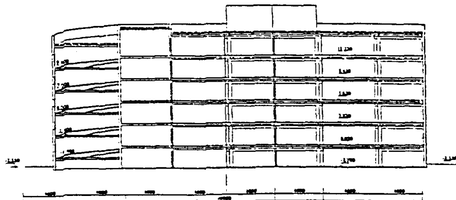
Разрез 1-1
