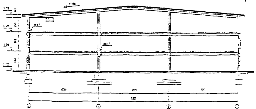
Разрез 1-1
