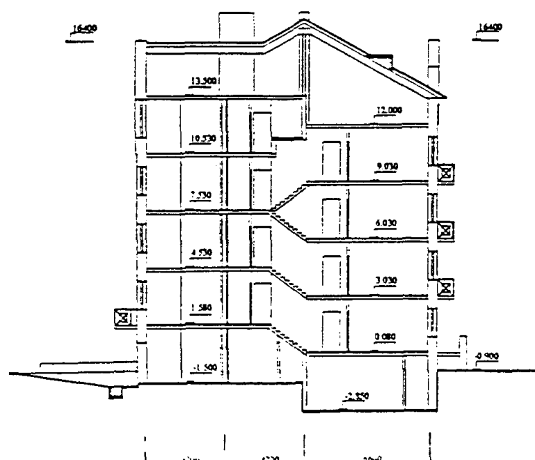
Разрез 1-1
