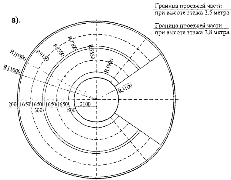
Рис. 9. Минимальная горизонтальная проекция двухпутной криволинейной ramпы.
