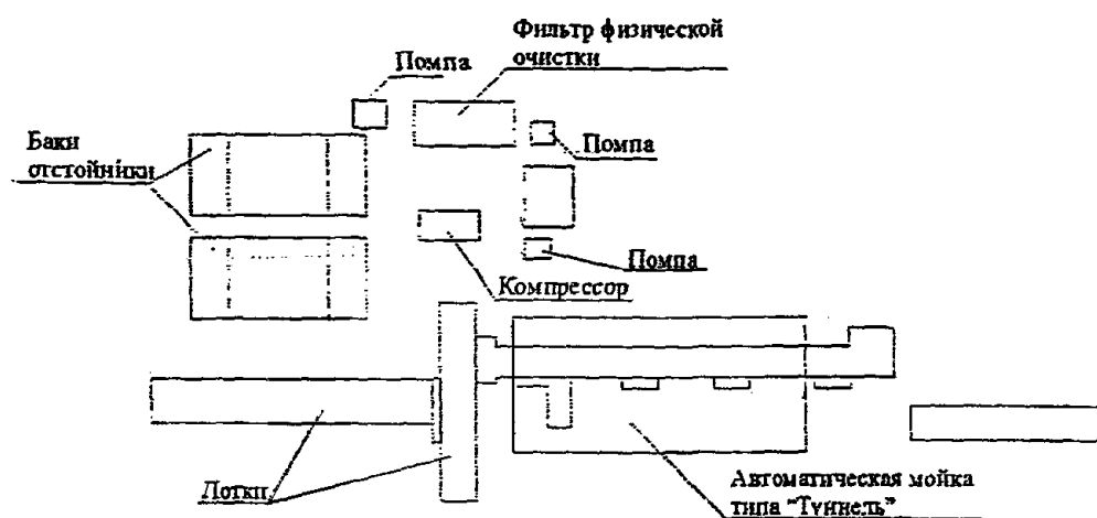
Рис. 14. Технологическая схема механизированной мойки типа "Туннель".
