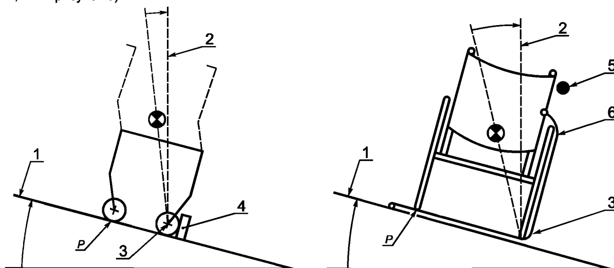
а) Незаблокированные передние колеса, вид спереди
