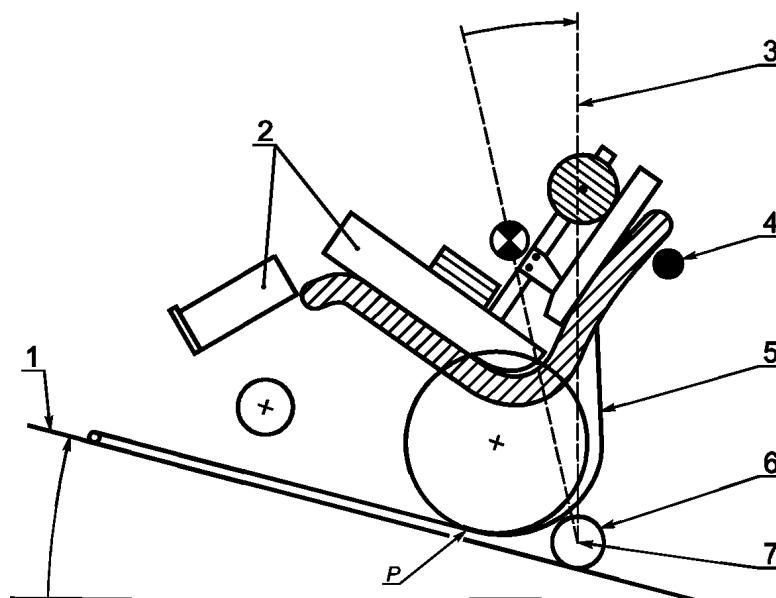
1 — испытательная плоскость; 2 — испытательный манекен; 3 — вертикаль; 4 — ограничитель дальнейшего опрокидывания; 5 — гибкая система удерживания; 6 — устройство против опрокидывания назад; 7 — ось опрокидывания; P — точка отрыва от испытательной плоскости
