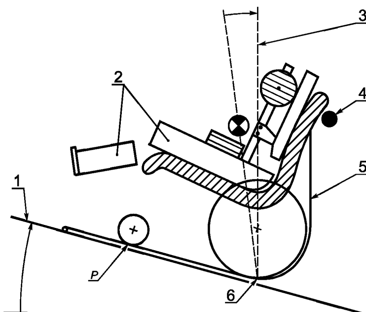
1 — испытательная плоскость; 2 — испытательный манекен; 3 — вертикаль; 4 — ограничитель дальнейшего опрокидывания; 5 — гибкая система удерживания; 6 — ось опрокидывания; P — точка отрыва от испытательной плоскости
