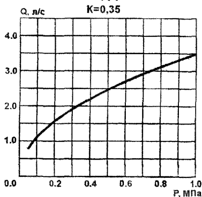
СВВ-12, ДВВ-12
