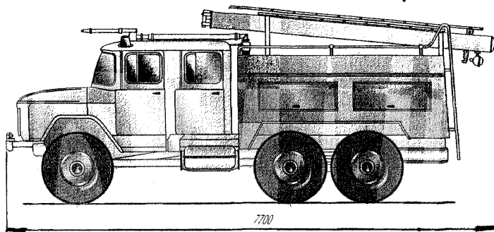
Рис.1 АЦ-25-40(ЗИП-131)-6BP
