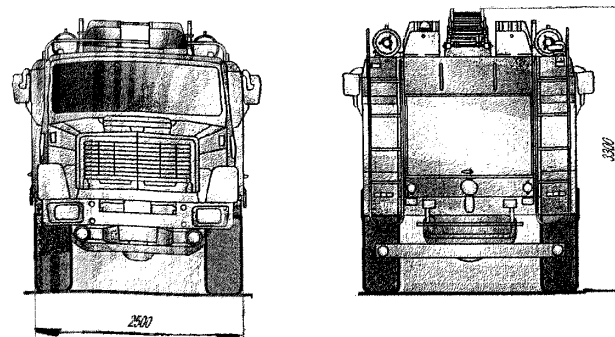
Рис.3 АЦ-3,0-40(ЗИП-4334)-3BP
