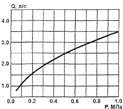
СВН-12, ДВН-12 K=0,47
