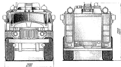
Рис. 7 АЦ-6,0-40(Урал-5557)-12БР
