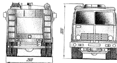
Рис. 8 АЦ-7,0-40(КамАЗ-532150)-21БР
