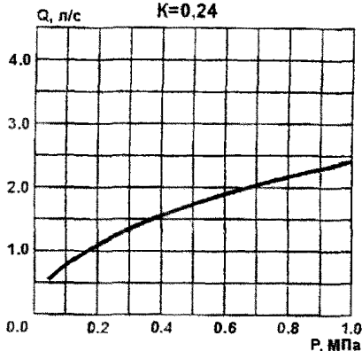
СВВ-10, ДВВ-10
