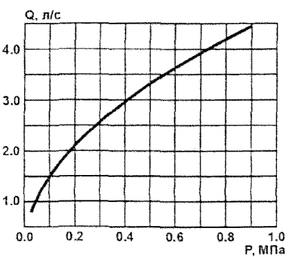
СВН-15, ДВН-15 K=0,77
