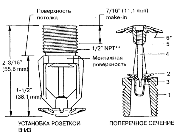
1/2" Сопло, 1/2" NPT резьба
