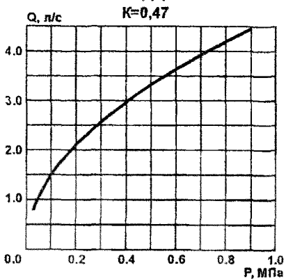
СВВ-15, ДВВ-15
