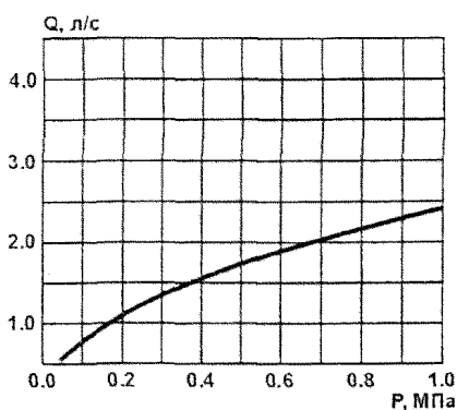
СВН-10, ДВН-10 K=0,35
