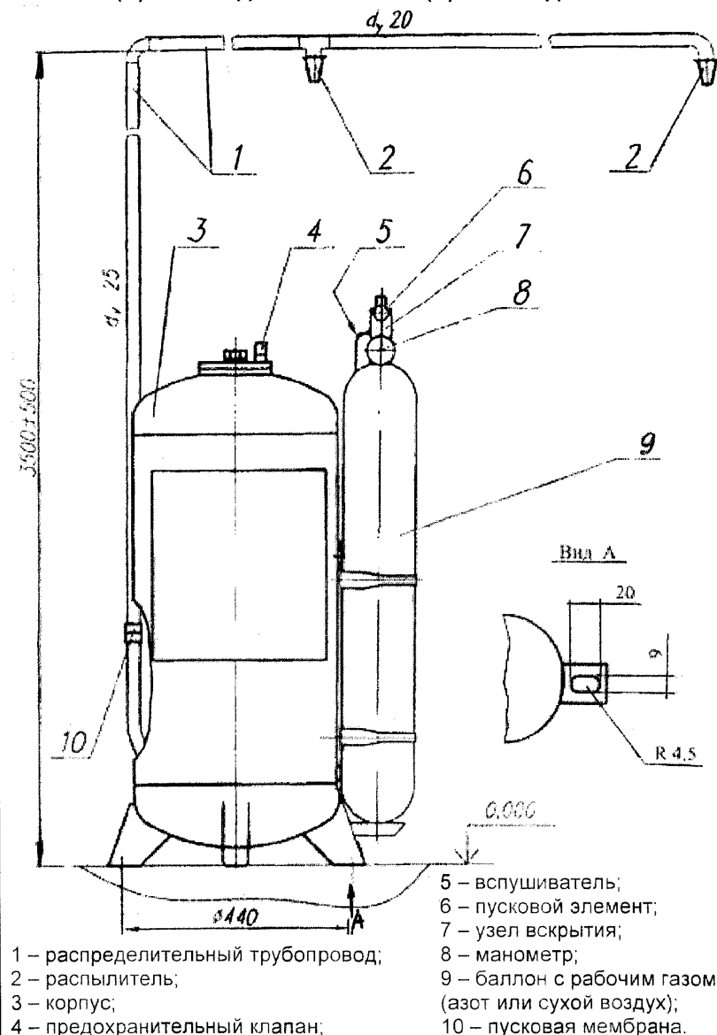
Общий вид модуля «Лавина» МПП(Н)-100-07-КД-2-БСГ-У2 и МПП(Н)-100-08-КД-2-БСГ-У2
