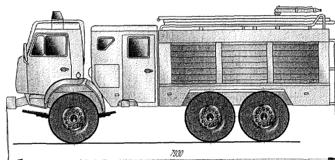
Рис.4 АЦ-4,0-40(Упан-5557)-9Б
