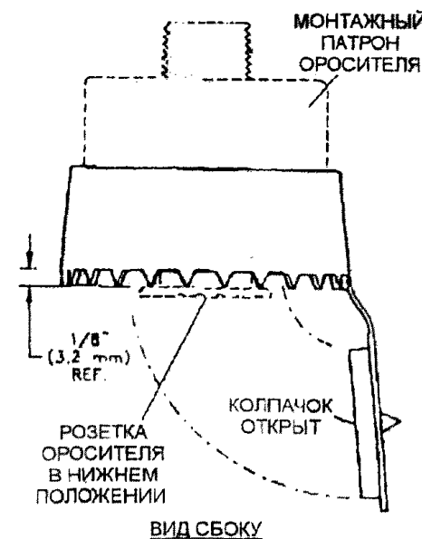
Рис.4 Защитный колпак
