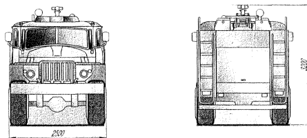
Рис. 9 АЦ-8,0-40(Урал-4320)-25БР
