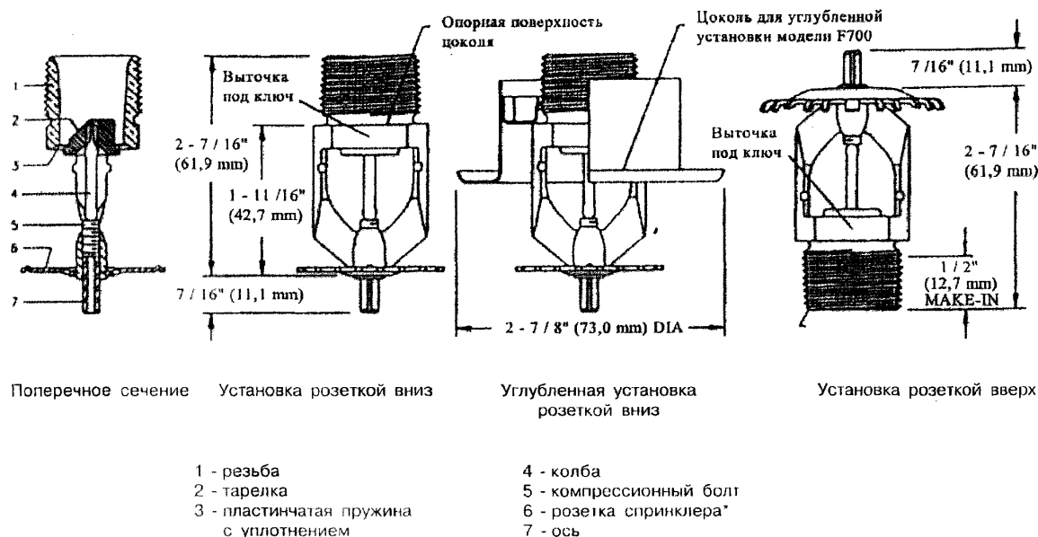
Рис.А: 5/8" и 3/4" sprinkлеры модели F895 розеткой вверх, вниз обычной и углубленной установки с увеличенной площадью орошения
