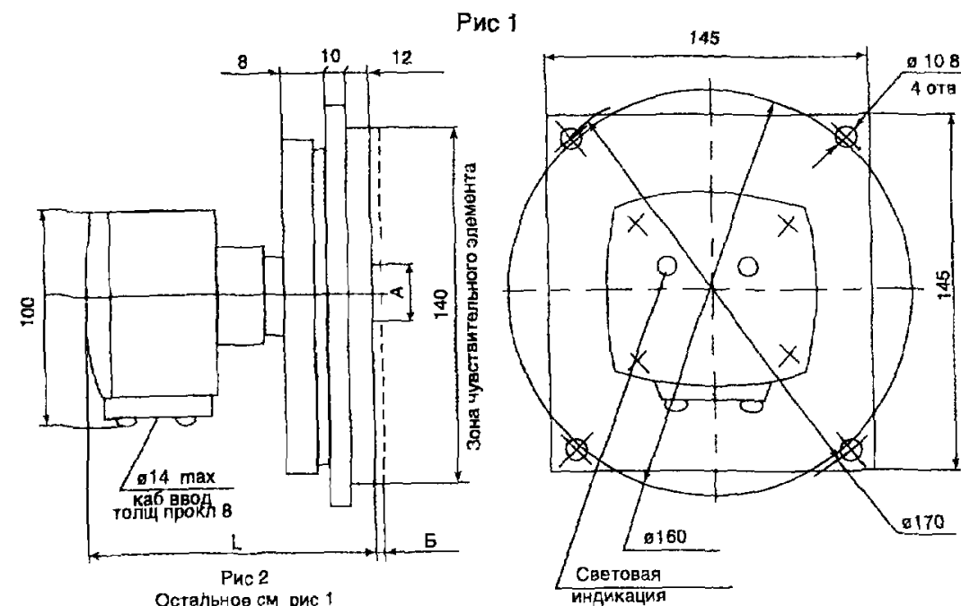
Датчики-реле РОС 171
