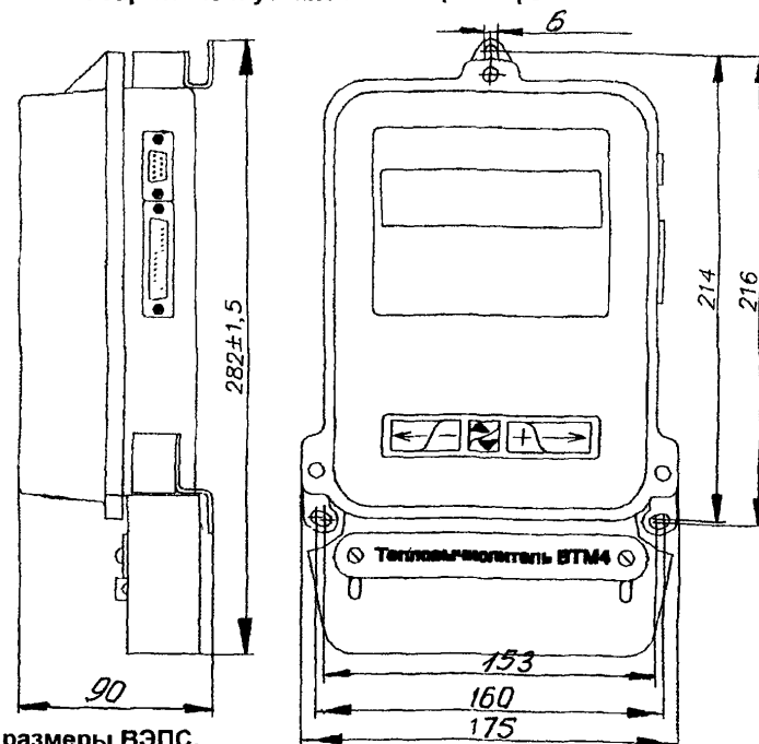
Габаритные и установочные размеры ВЭПС.
