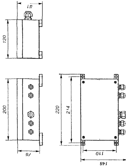
Преобразователь ДРК-ЗЭПХ
