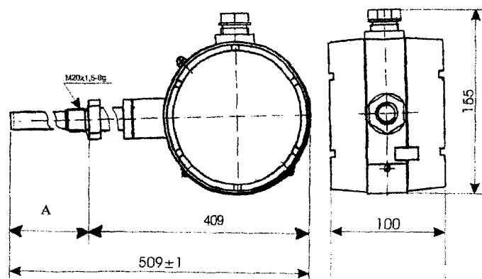
Габаритные размеры УСУ-1
