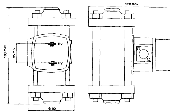
Первичный преобразователь
