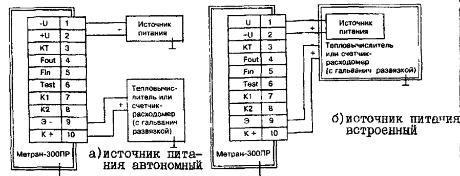
Рис. 2. Блок-схемы подключения Метран-300ПР с выходным сигналом "замкнуто/разомкнуто" (ОП).
