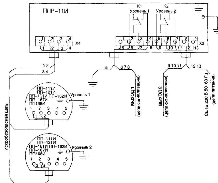
Схема электрических внешних соединений РОС 102-И
