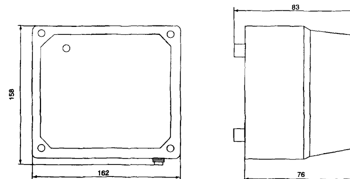
Передающий преобразователь
