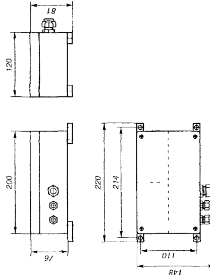
Преобразователь ДРК-ЗОП
