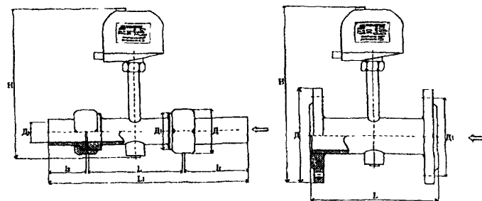
Габаритные и установочные размеры ВЭПС.
