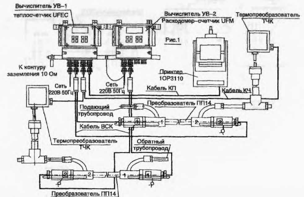
Рис. 1 – схема установки теплосчетчиков моделей UFEC 005-1C
