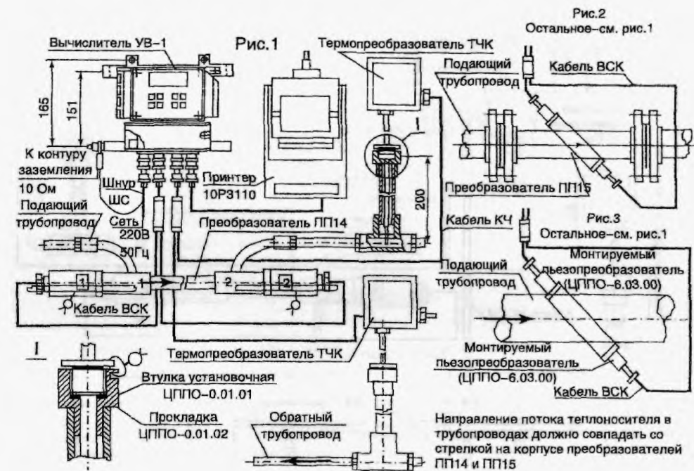
Рис. 1 – схема установки теплосчетчиков моделей UFEC 005-1C
