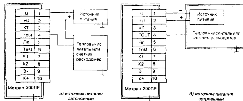
Рис. 1. Блок-схемы подключений Метран-300ПР с токоимпульсным (ТИ) выходным сигналом.
