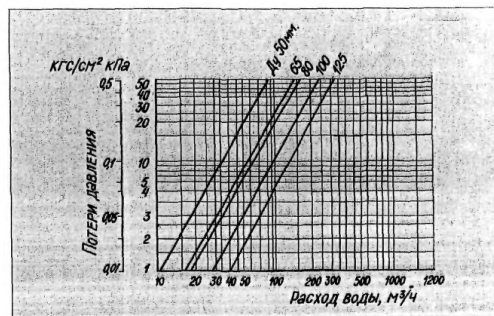
Гидравлические характеристики турбинных счетчиков Ду 50-250 мм
