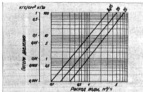
Гидравлические характеристики крыльчатых счетчиков Ду 15-40 мм
