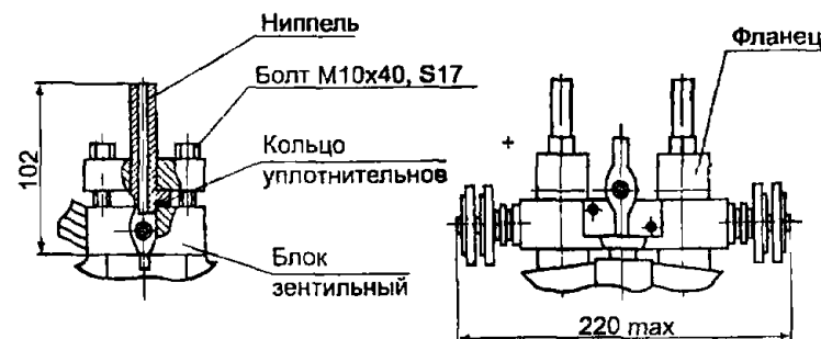
Рис.10. Преобразователь с установленными вентильным блоком и ниппелями под закладные гайки M20x1.5, остальное см. рис.6
