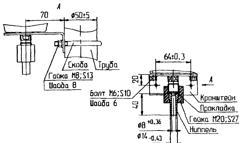
Рис 13. Присоединительные размеры для 141 Остальное см рис 11 и 12
