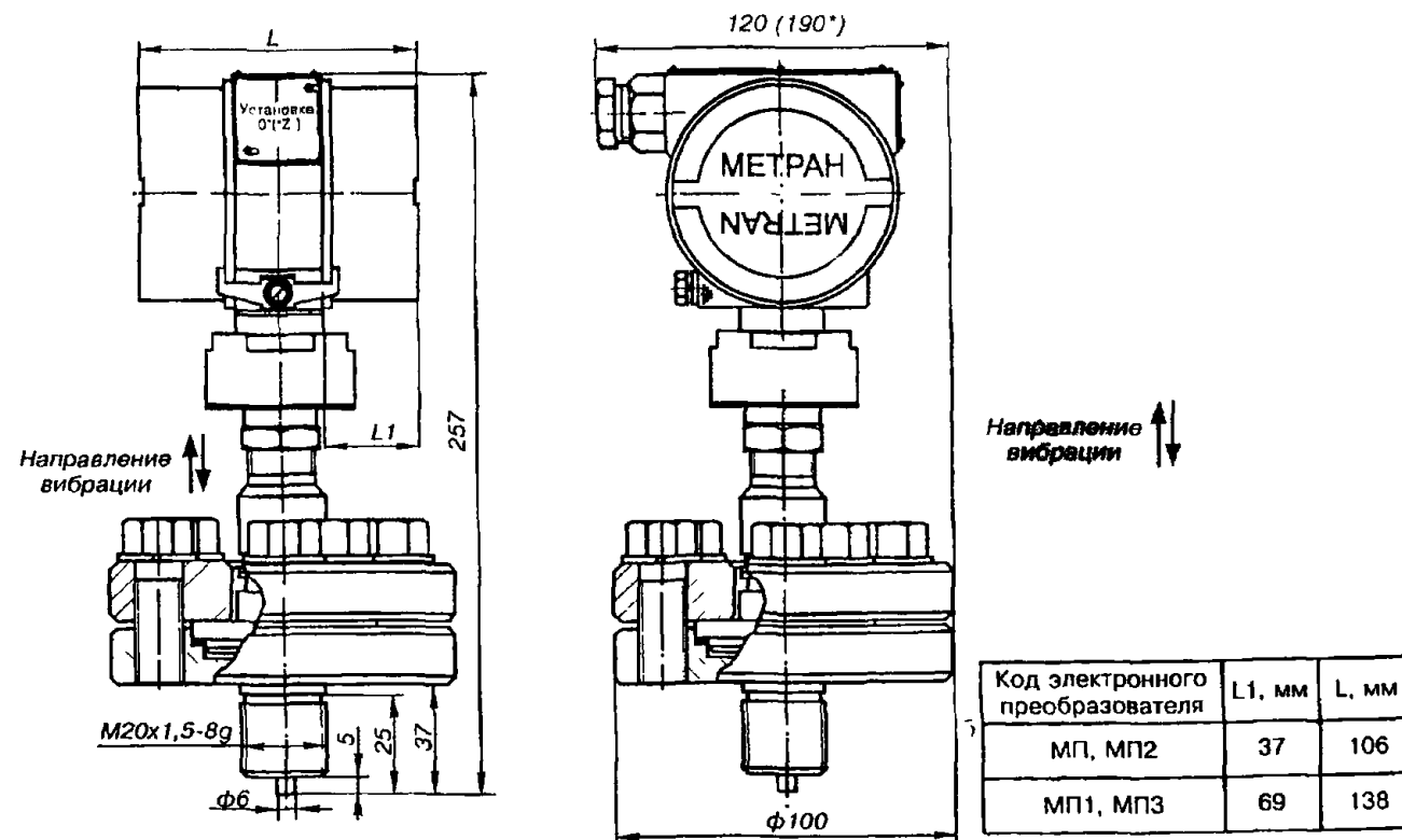
ФАБРИТНЫЕ И ПРИСОЕДИНИТЕЛЬНЫЕ РАЗМЕРЫ ДАТЧИКОВ МЕТРАН-49
