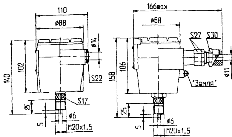
Рис 12. Модели 11229 11239 Исполнение Вн ("взрывонепроницаемая оболочка")
