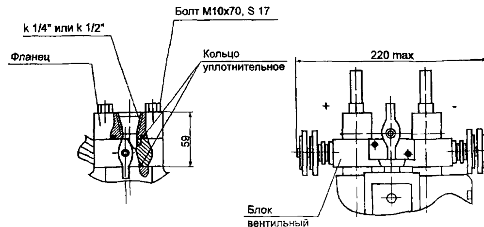
Рис.11. Преобразователь с установленными вентильным блоком и фланцами, остальное см. рис.6
