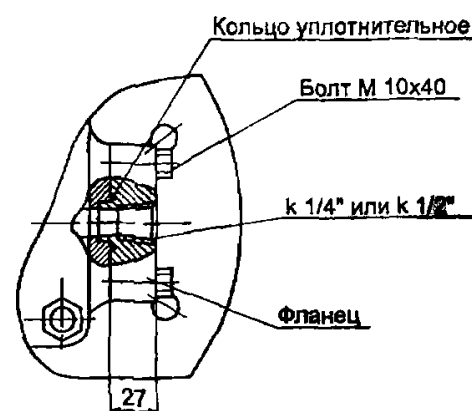
Рис.14. Преобразователь с установленными фланцами, остальное см. рис.12
