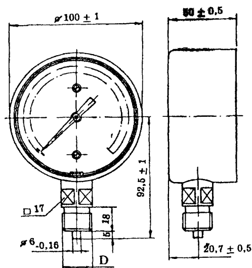
Габаритные и присоединительные размеры манометра без борта
