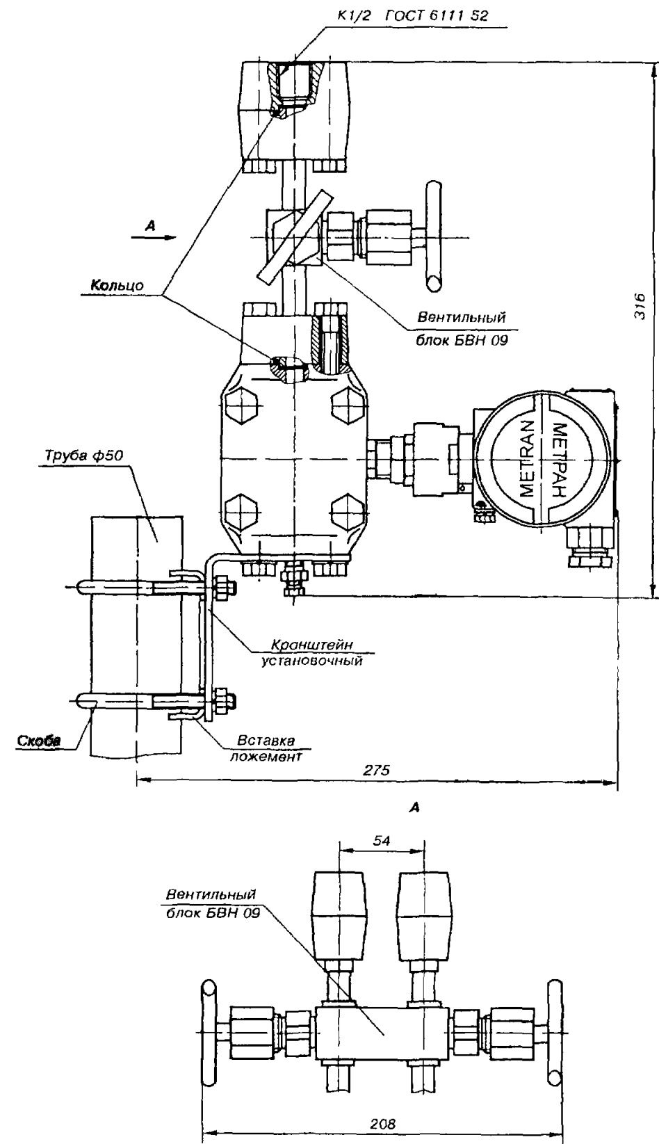
Рис.7. Метран-49-ДД мод.9420, 9430, 9440 с вентильным блоком БВН 09.
