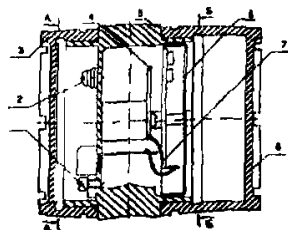
Рис.15. Устройство электронного блока
