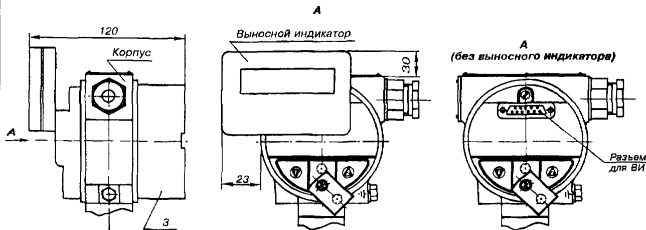
Вид электронного преобразователя датчиков МП
