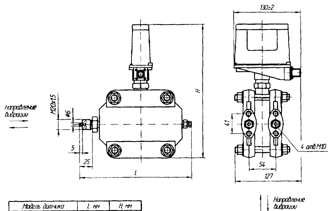
Рисунок 4 Габаритные и присоединительные размеры датчиков моделей 2410, 2420, 2434, 2444, 2450, 2464
