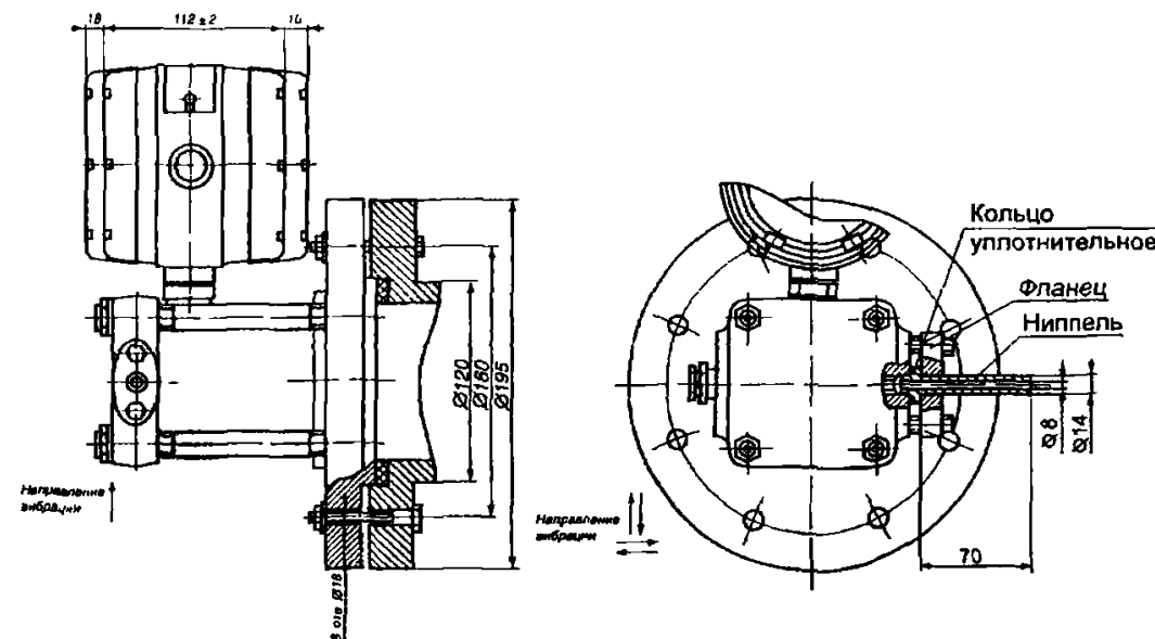
Рис.13. Преобразователь с установленными ниппелями под накидные гайки М20х1,5, остальное см. рис.12
