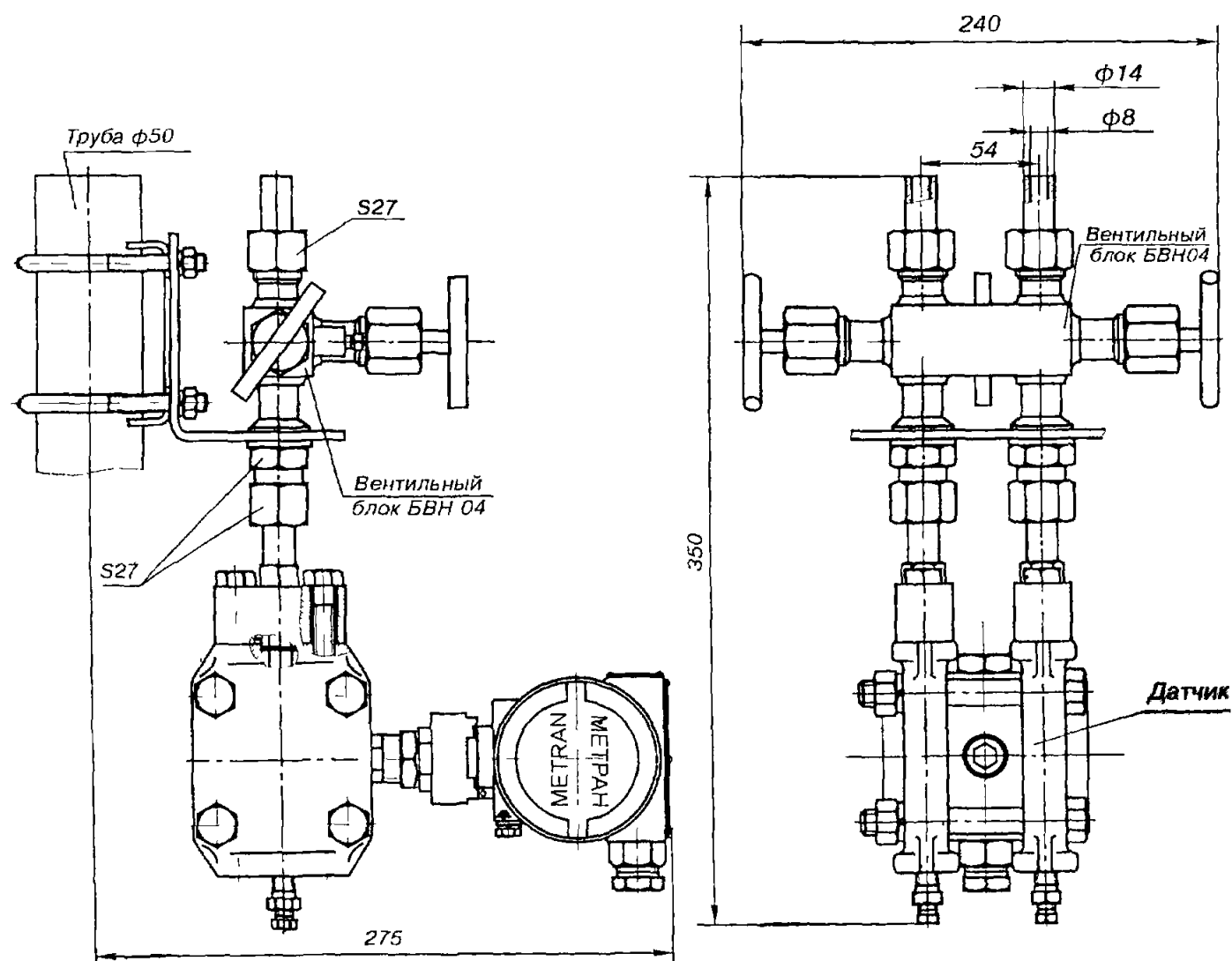
Рис.6. Метран-49-ДД мод.9420, 9430, 9440 с вентильным блоком БВН 04.
