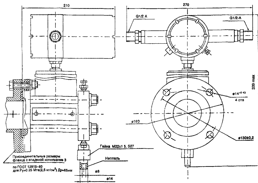
Рис.1. Габаритные, установочные и присоединительные размеры преобразователя Сапфир-22К-ДГ-Вн
