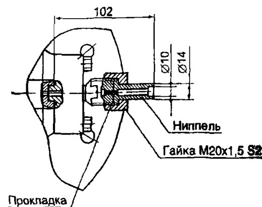
Рис.13. Преобразователь с установленными ниппелями под накидные гайки М20х1,5, остальное см. рис.12
