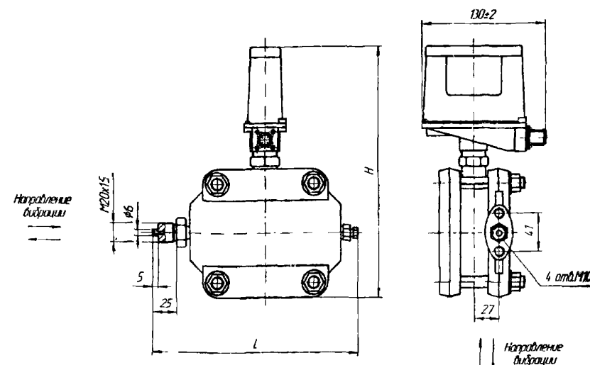
Рисунок 2. Габаритные и присоединительные размеры датчиков моделей 2020, 2030, 2040, 2110, 2120, 2130, 2140, 2210, 2220, 2230, 2240, 2310, 2320, 2330, 2340
