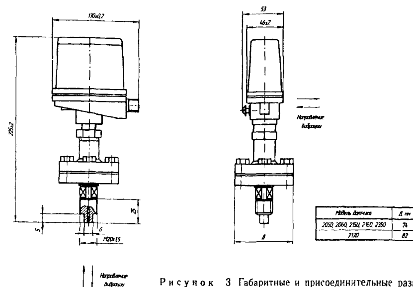
Рисунок 3. Габаритные и присоединительные размеры датчиков моделей 2050, 2060, 2150, 2160, 2170, 2350
