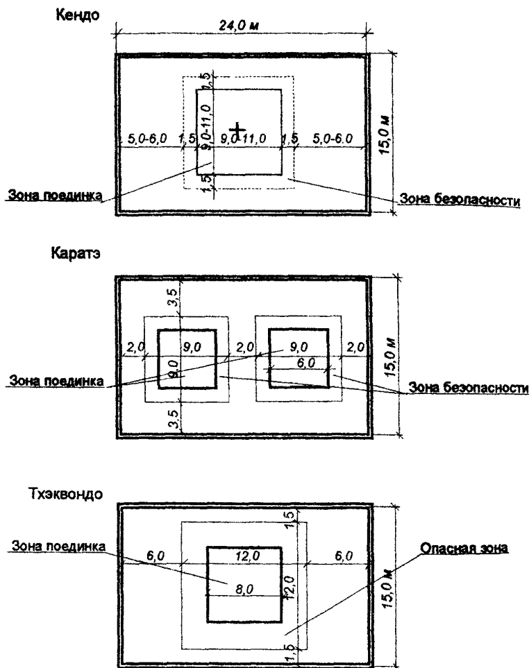
Рис.5. Схемы размещения площадок для учебно-тренировочных занятий кендо, карате, тхэквондо в зале 24 х 15 м.
