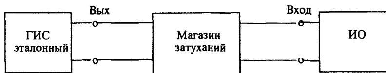
Рисунок 11 - Схема проверки измерения ошибок ИО
