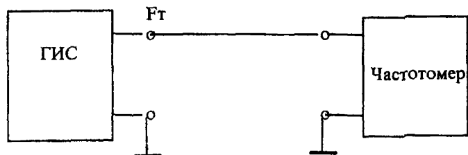
Рисунок 6 - Схема для измерения частоты сигнала
