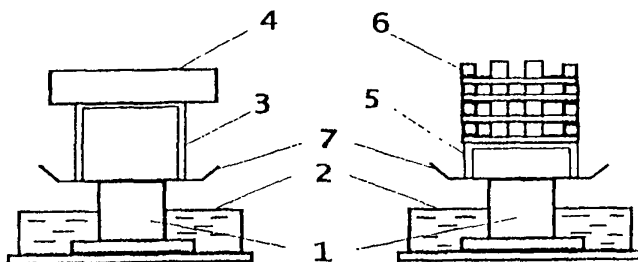
Рис. 2. Модельные очаги для различных видов горючих материалов:
