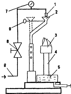
Рис. 1. Схема испытательного стенда:
