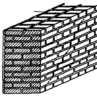
510 Цепная кладка с нормальными швами
