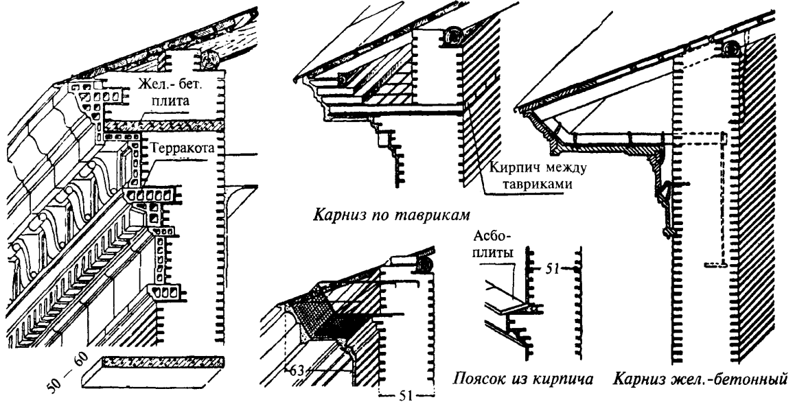
Карниз терракотовый
