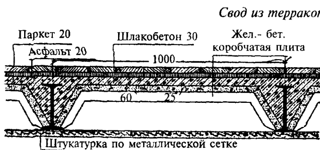
Заполнение из коробчатых жел.-бет. элементов
