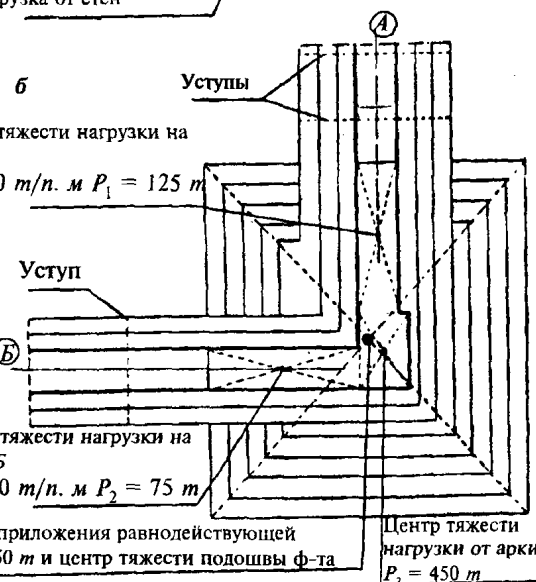
План фундамента и расположение нагрузок
