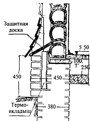
Цоколь с термо-вкладышем
