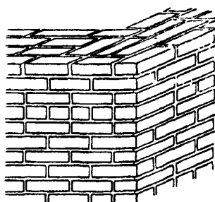
Кладка угла без трехчетвертных кирпичей
