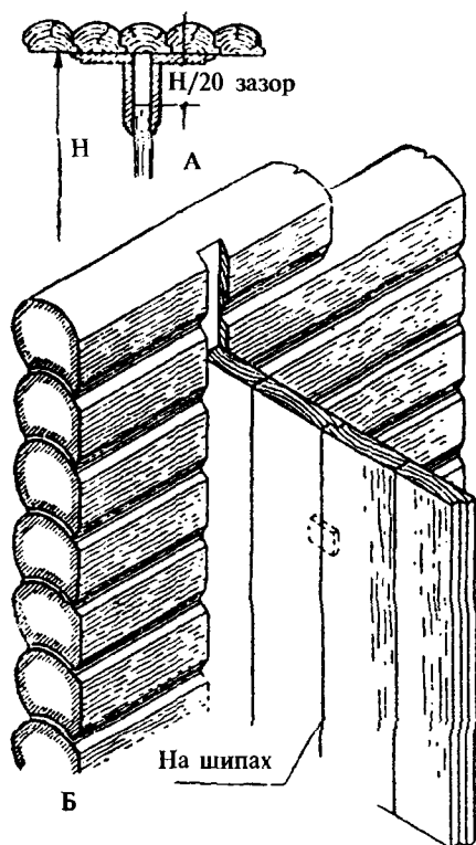
Присоединение перегородки к потолку (А) и к стене (Б)
