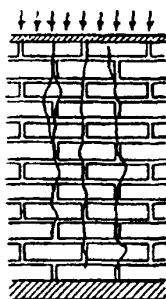
Работа кирпича в кладке
