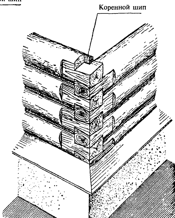
Общий вид сруба без остатка
