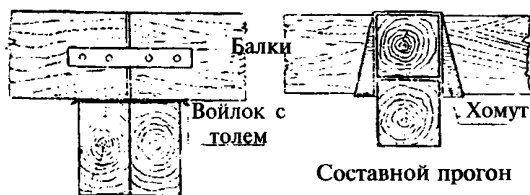
Парный прогон
