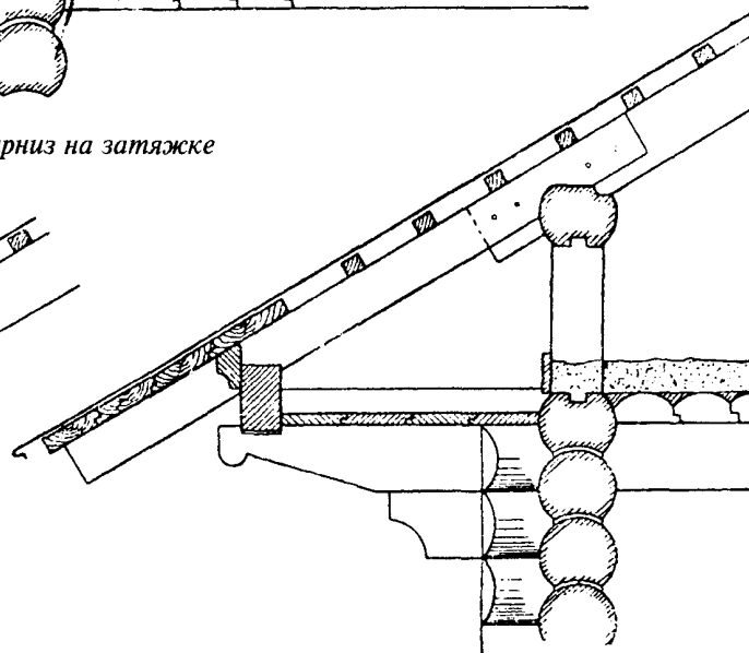
Карниз на консолях
