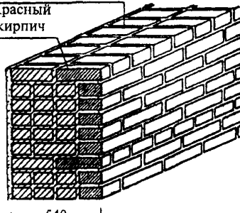
540 Кладка из силикатного кирпича с облицовкой красным
