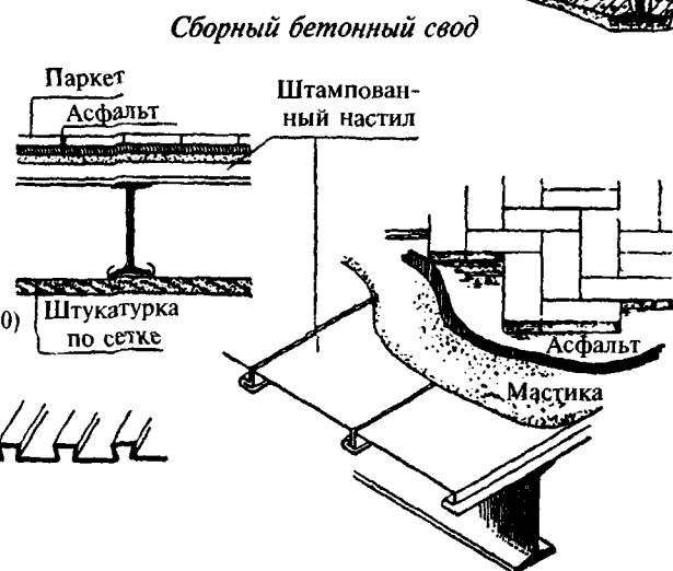
Перекрытия с штампованным настилом
