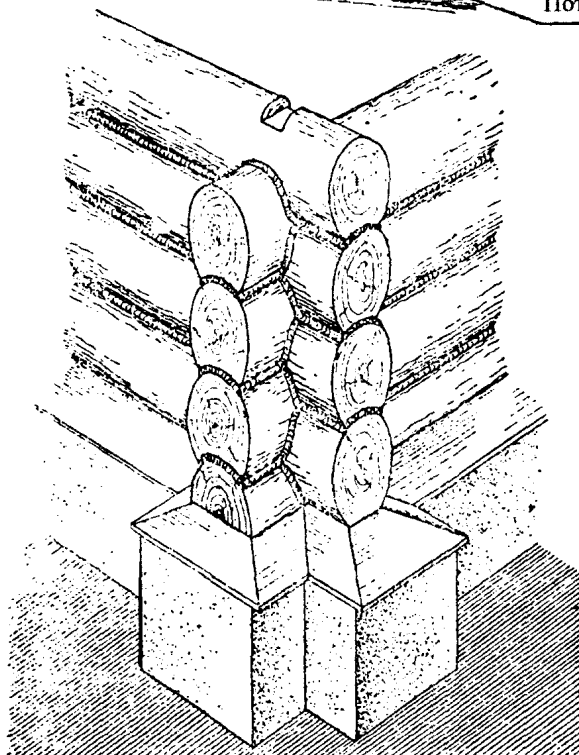
Общий вид сруба с остатком
