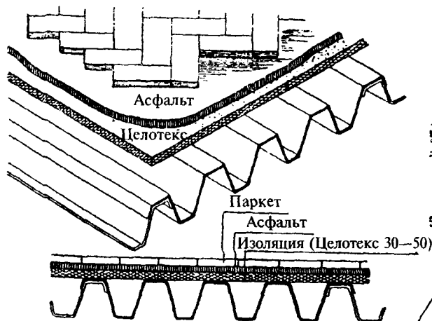
Перекрытия из штампованных профилей (американский тип)
