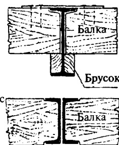
Опираие балок на стальные прогоны
