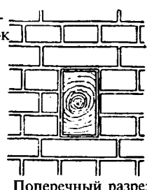
Глухая заделка балок в наружную стену
