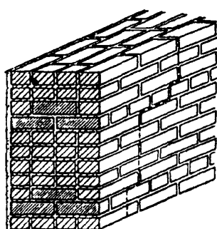
510 Американская кладка с нормальными швами
