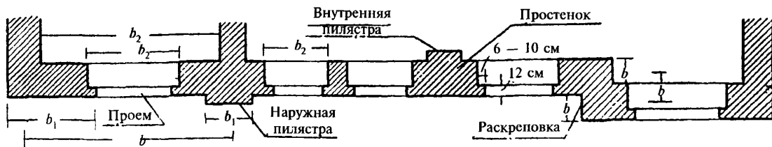
Система перевязки кирпичной кладки
