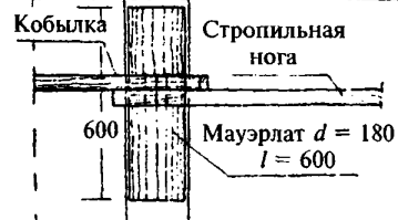
Опираие дощатой стропильной ноги на мауэрлат
