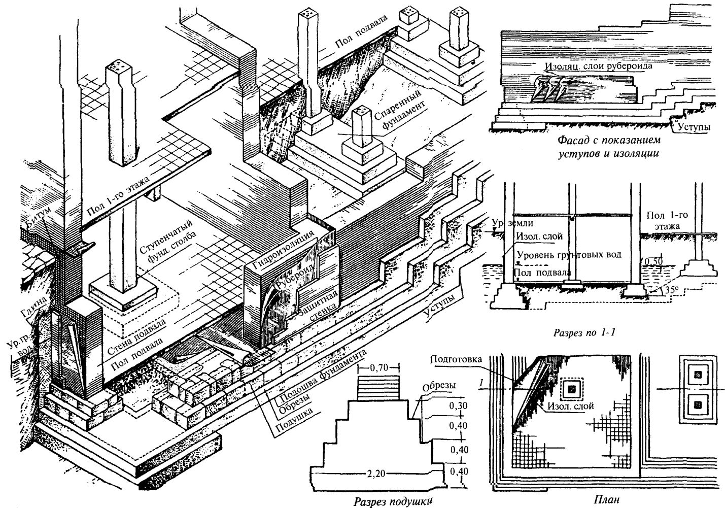
Общий вид фундаментов
