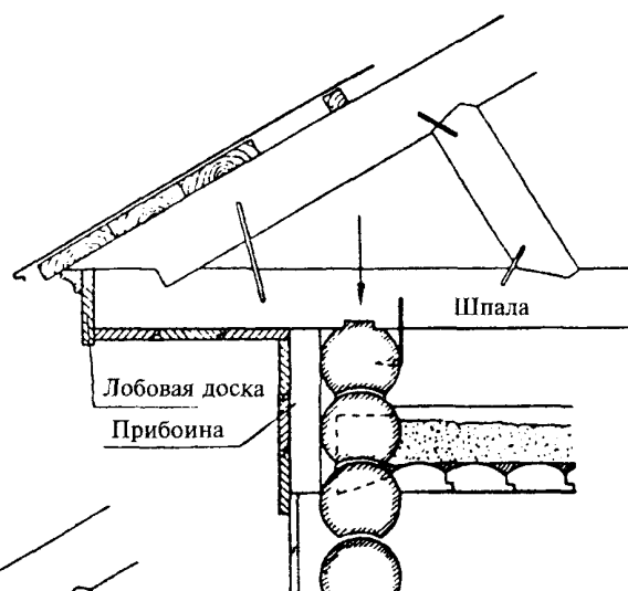
Карниз на шпалах
