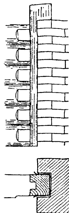
Присоединение рубленых стен к каменным
