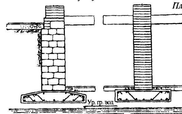
Расположение уступов в подвале
