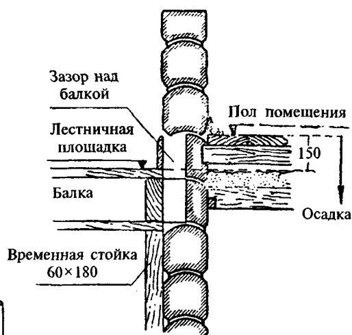
Присоединение лестничной площадки в 2-этажном здании
