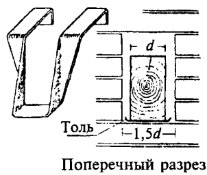
Заделка балки во внутреннюю стену 51 см
