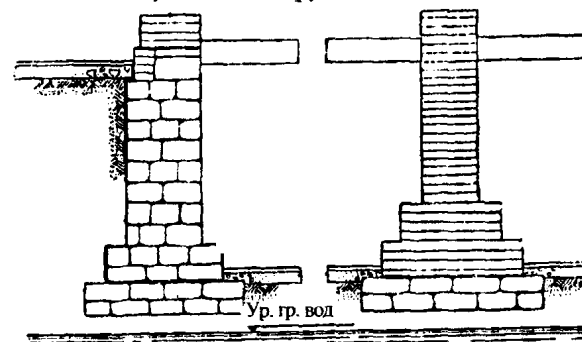
Расположение уступов в подвале
