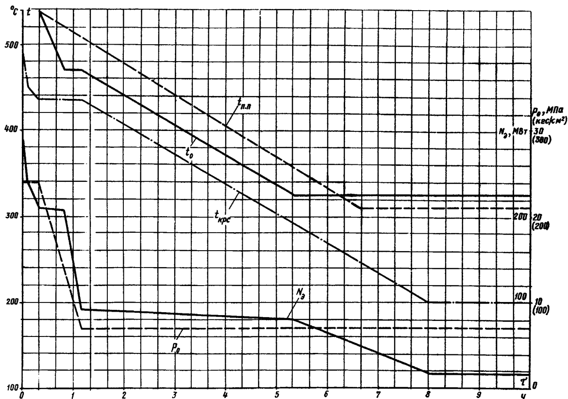
Рис.10. График-задание останова блока с расхолаживанием турбины
