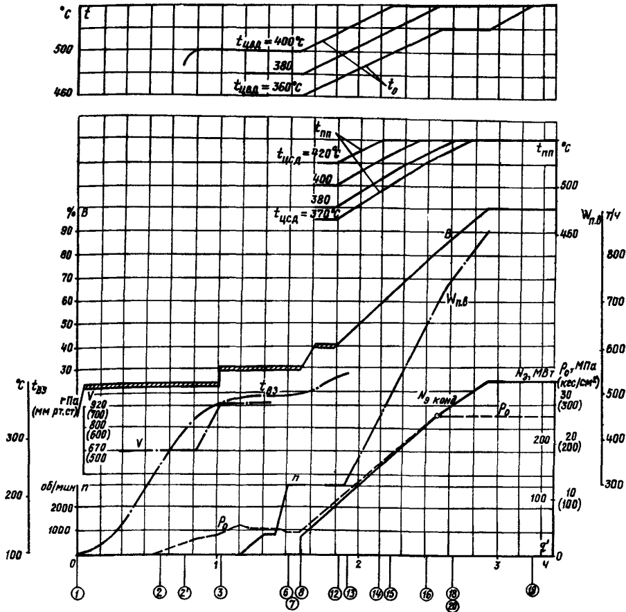
Рис.7. График-задание пуска блока из неостывшего состояния (температура паровпуска ЦВД 400-360°C, температура паровпуска ЦСД 420-370°C, продолжительность простоя 10-19 ч)
