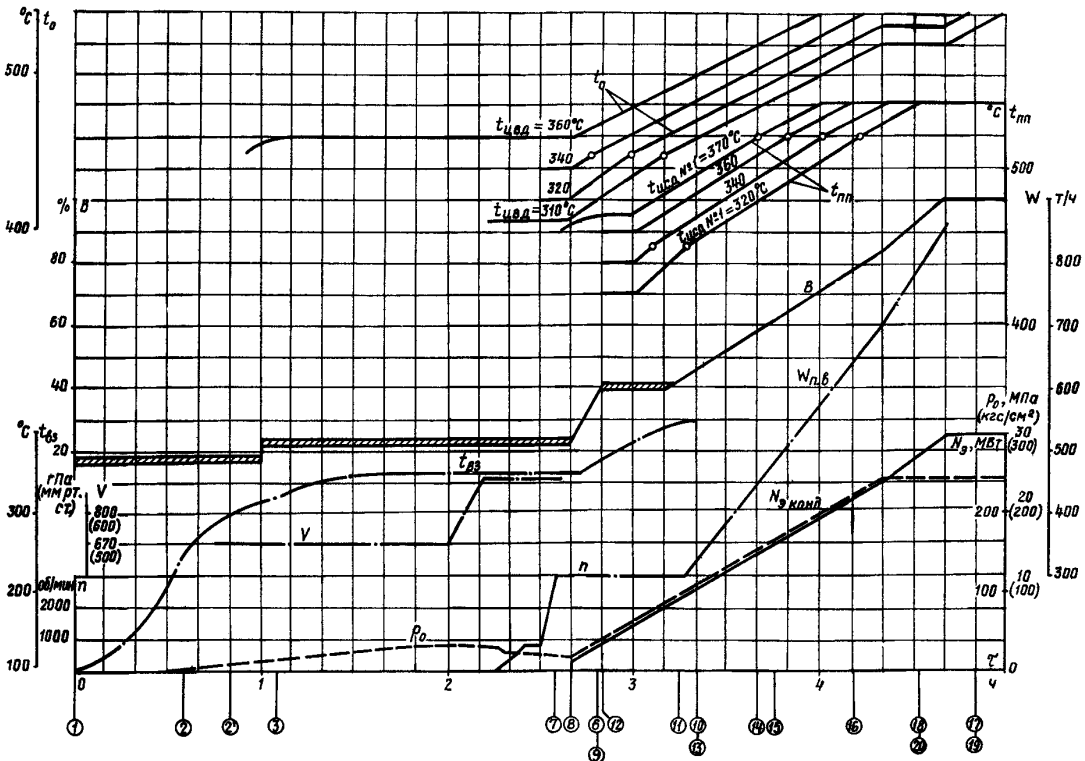
Рис. 6. График-задание пуска блока из неостывшего состояния (температура паровпуска ЦВД 360–310°C, температура паровпуска ЦСД 370–320°C, продолжительность простоя 19–30 ч)
