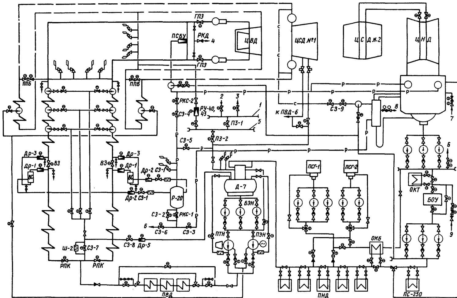
Рис. 1. Типовая пусковая схема моноблока 250 МВт с турбиной Т-250/300-240: 1 - общестанционная магистраль; 2 - от пусковой котельной; 3 - к блокам; 4 - в конденсатор; 5 - коллектор собственных нужд блока; 6 - в циркуляционный водовод; 7 - нормальная подпитка блока; 8 - аварийная подпитка блока; 9 - от насосов БЗК
