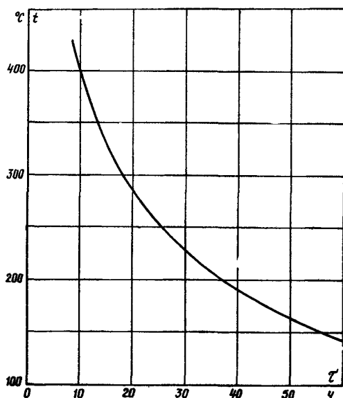
Рис. 2. Допустимые характеристики естественного остывания передусных труб высокого давления
