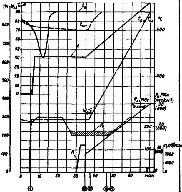
Рис.9. График-здание пуска блока из состояния горячего резерва
