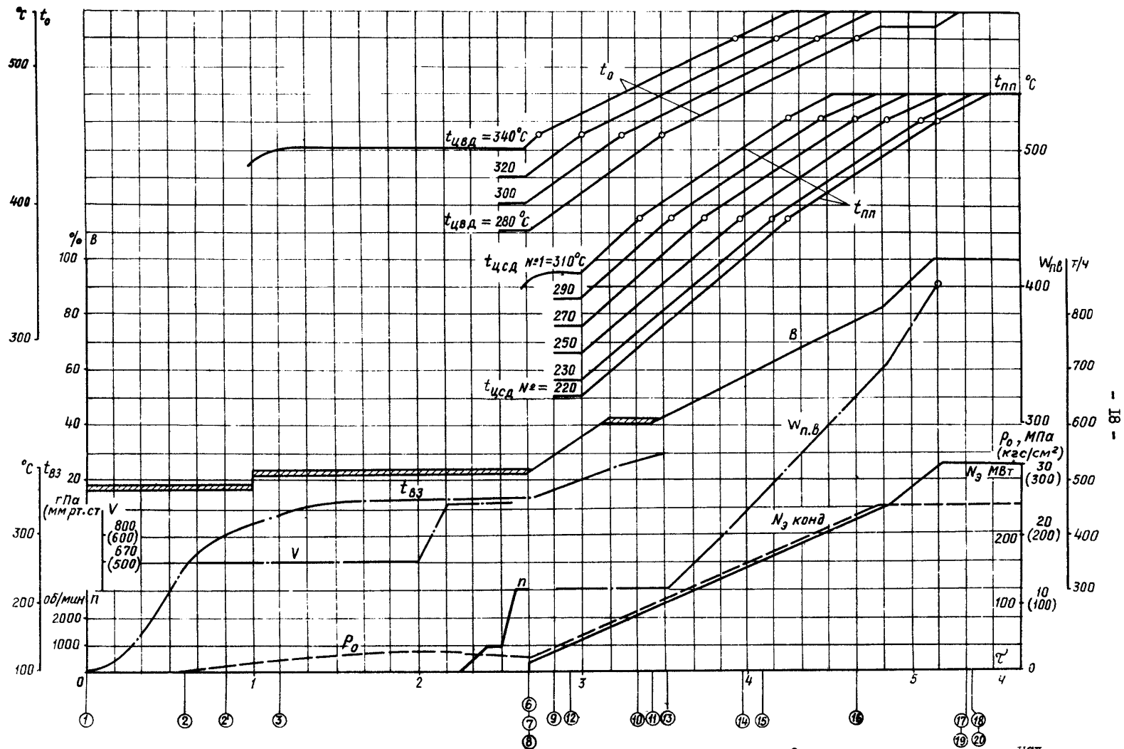
Рис. 5. График-задание пуска блока из неустойчивого состояния (температура паровпуска ЦВД 340–280°C, температура паровпуска ЦСД 310–220°C, продолжительность простоя 32–55 ч)
