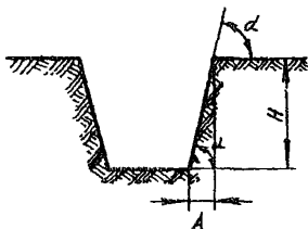
Рис.2.7. Определение крутизны откоса
