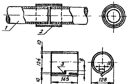
Рис.2.14. Стык асбестоцементных труб с помощью стальных манжет:
