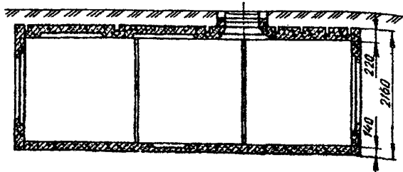
Рис.3.22. Проходной сборный железобетонный колодец специального типа ККС-2 на 37-48 каналов трубопровода
