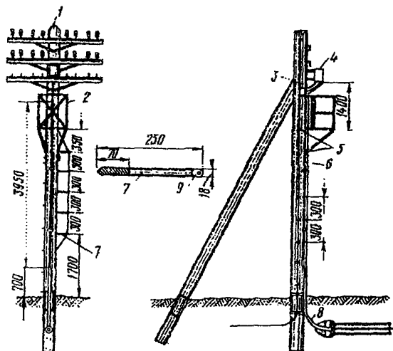
Рис. 8.25. Кабельная опора:
