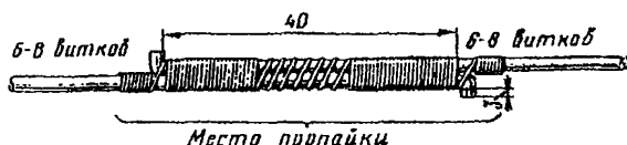
Рис. 8.37. Соединение стальных проводов наложением на сrostок бандажа из оцинкованной перевязочной проволоки
