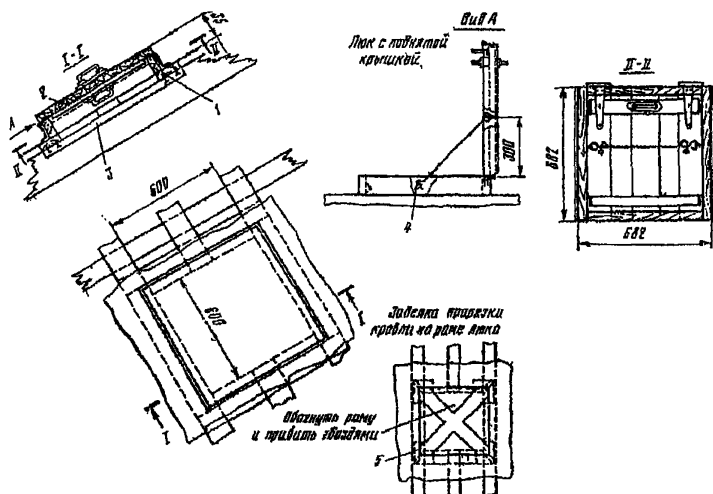
Рис. 9.15. Люк для выхода на крышу (место соприкосновения кровли с оковкой угловой рамы и все щели промазывать замазкой на сурике):
