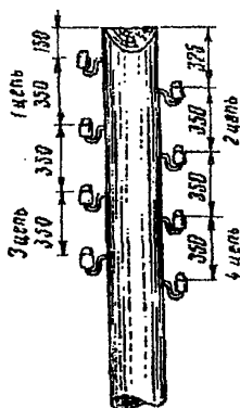
Рис. 8.9. Оснастка опоры крюками с изоляторами
