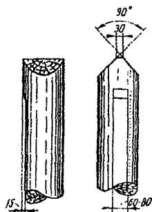
Рис. 8.5. Правильно обработанная вершина опоры
