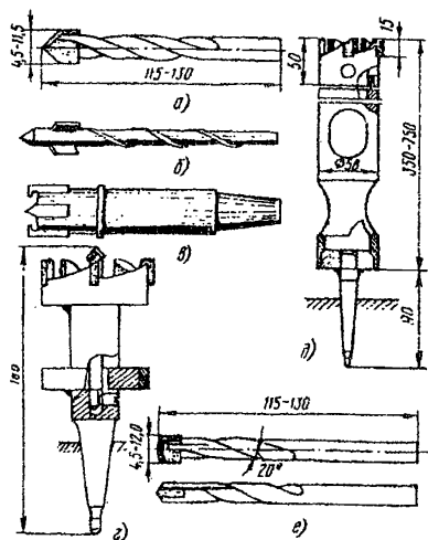
Рис. 7.19. Рабочие инструменты для пробивных работ:
