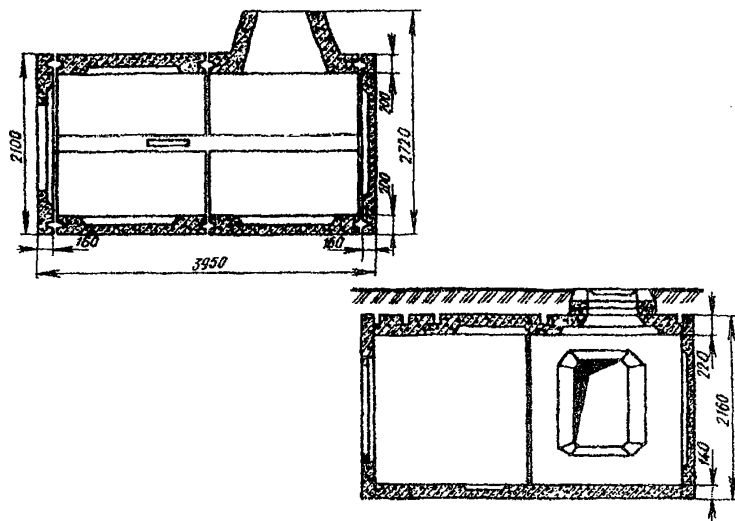
Рис.3.23. Угловой сборный железобетонный колодец специального типа KKCCy-1
