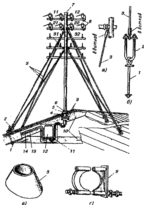
Рис. 9.7. Установка стойки 10х2 и детали ее крепления:
