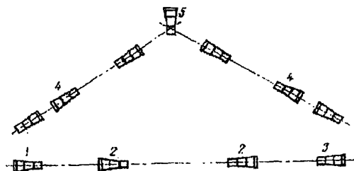
Рис. 8.17. Расположение ям для промежуточных, угловых и оконечных опор при рытье ручным способом
