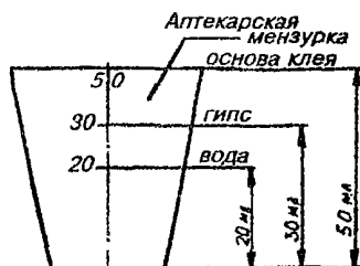
Рис.7.24. Пропорции компонентов для составления клея "Стык-10"
