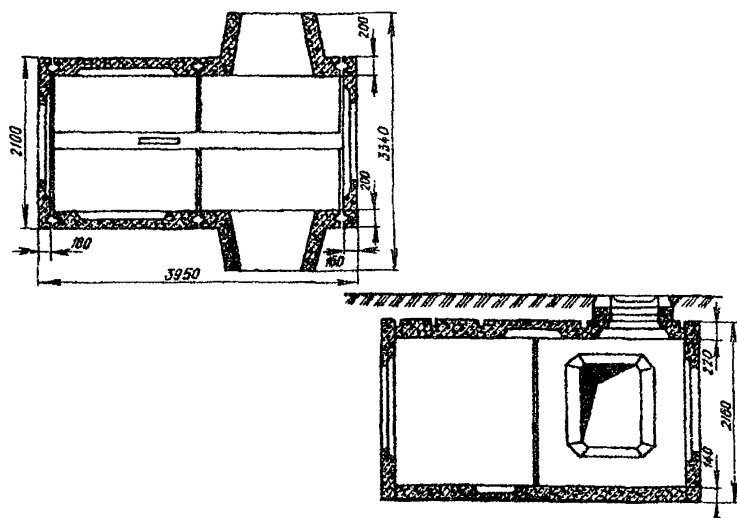
Рис.3.24. Разветвительный сборный железобетонный колодец специального типа KKCCp-1
