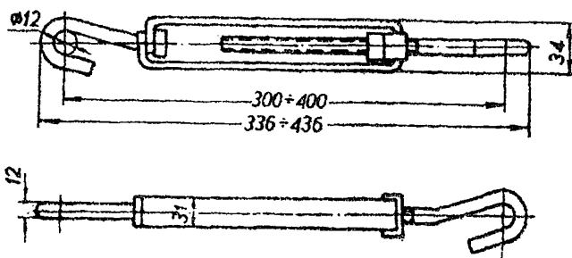
Рис. 7.11. Винтовая стяжка (тальер)
