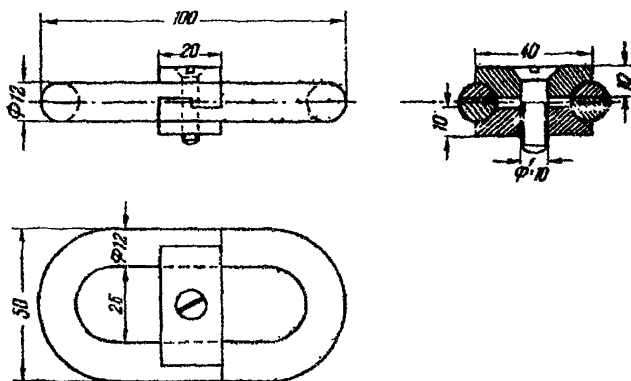
Рис. 4.4а. Карабин
