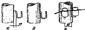
Рис. 8.8. Правила ввертывания крюков
