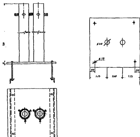
Рис 9.12. Опорная плита с двумя приваренными гильзами для установки стойки вместе с выводной трубой
