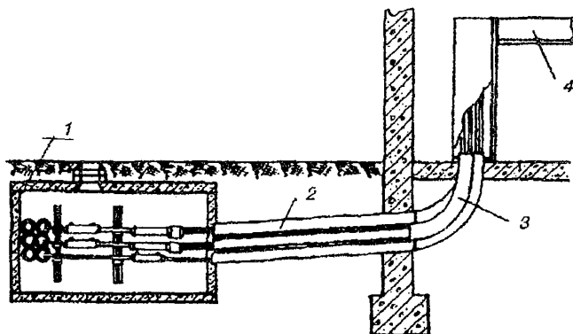
Рис.3.48. Ввод кабелей с распайкой в станционном колодце:
