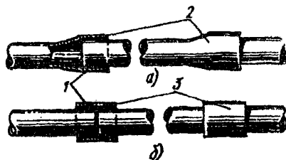
Рис.3.12. Соединение поливинилхлоридных (винилитовых) труб;
