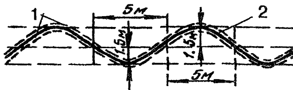
Рис.2.6. Зигзагообразная траншея при уклоне 30-45^\circ : 1 - траншея; 2 - кабель
