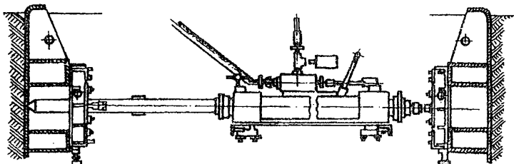
Рис.2.16. Установка гидравлического пресса в рабочем котловане
