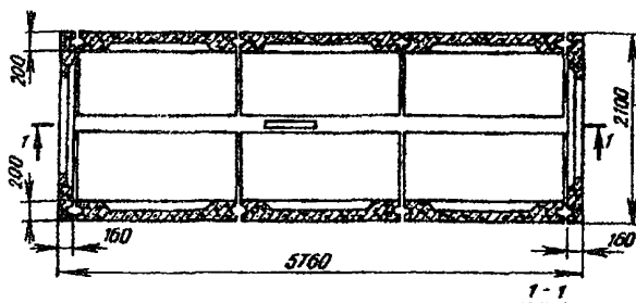
Рис.3.21. Проходной сборный железобетонный колодец специального типа ККС-1 на 25-36 каналов трубопровода
