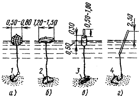
Рис.6.2. Временные буи для ориентировки створа перехода:
