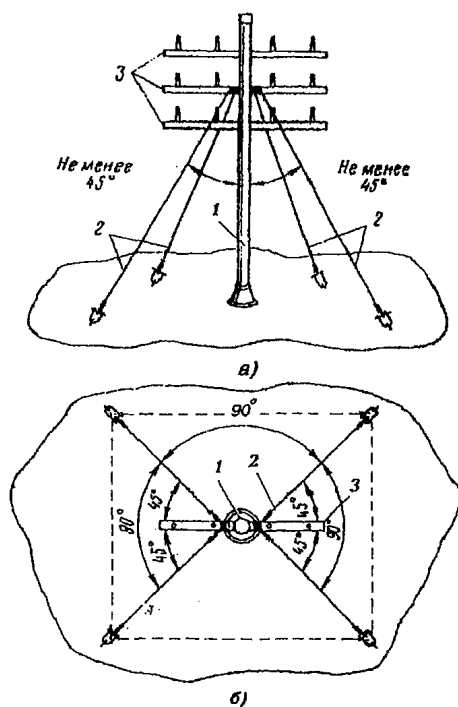
Рис.9.8. Расположение оттяжек стойки: а - вид спереди: 1 - вертикальная труба стойки; 2 - оттяжки; 3 - траверсы; б - вид сверху
