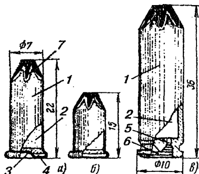
Рис.7.28. Монтажные патроны:
