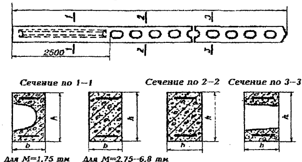
Рис.8.3. Опоры типа ПО и ПОН
