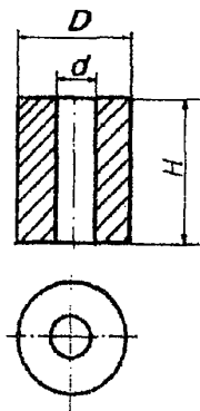
Рис. 8.33. Термитно-мufельный патрон
