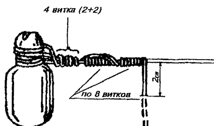
Рис. 9.21. Закрепление провода на изоляторе оконечной телефонной стойки
