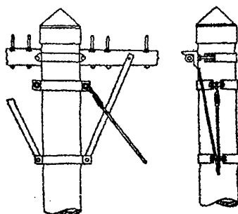
Рис 8.22. Крепление подкосов и оттяжек к железобетонной опоре
