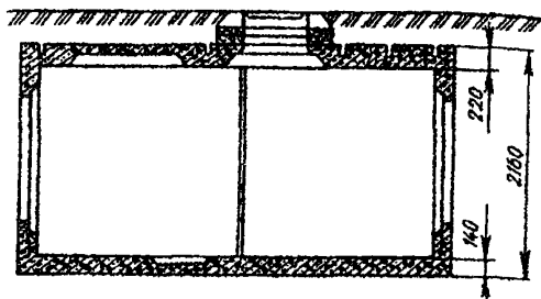
Рис.3.21. Проходной сборный железобетонный колодец специального типа ККС-1 на 25-36 каналов трубопровода
