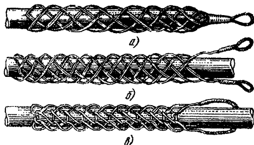
Рис.4.6. Чулки стальные кабельные:
