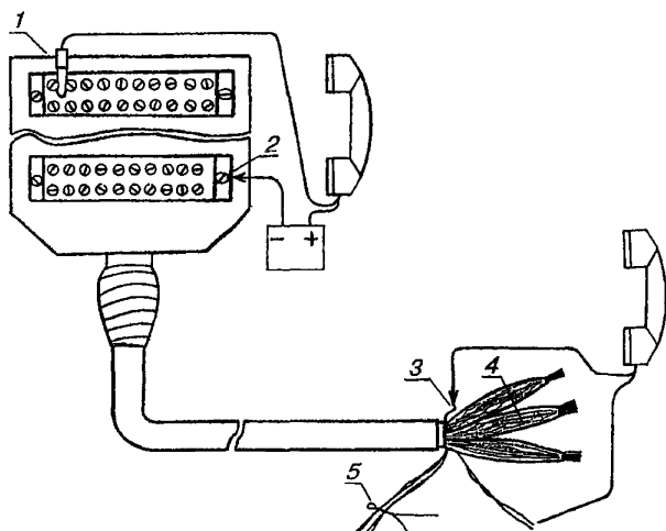
Рис.11.30. Прозвонка бокса в сборной муфте:
