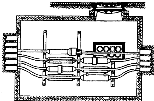
Рис.11.1. Расположение муфт в колодцах кабельной канализации и коллекторах
