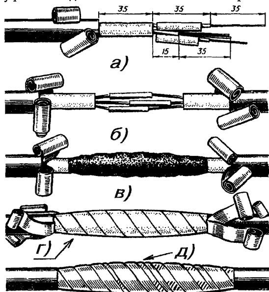
Рис.11.62. Монтаж прямой муфты на кабеле КСПП 1x4 "холодным" способом
