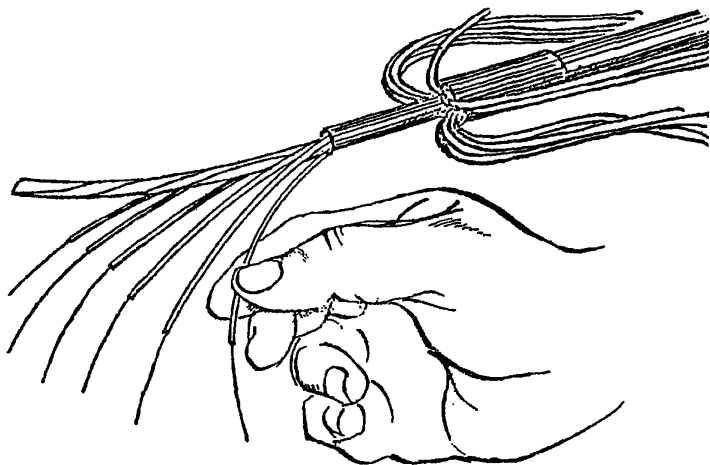
Рис.12.12. Установка полиэтиленовых трубочек под внутреннюю оболочку в пазы центрального элемента
