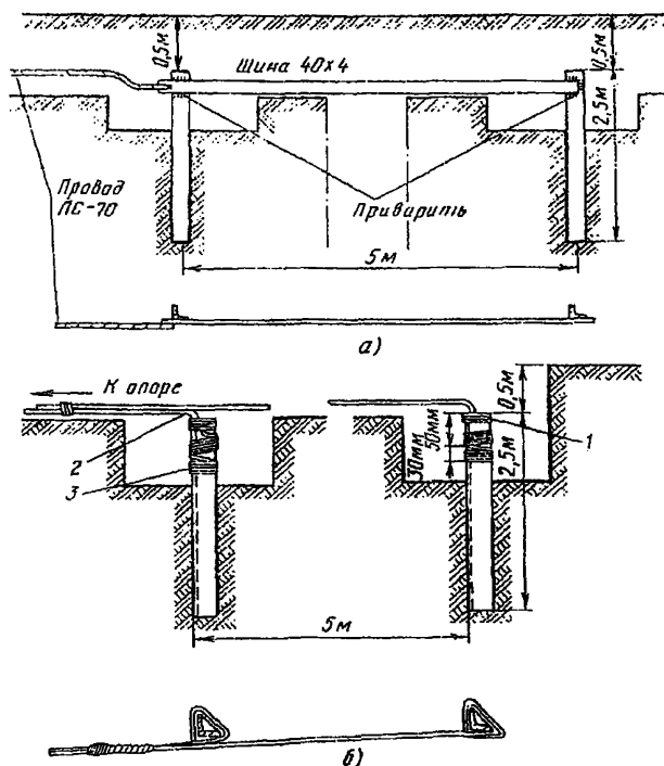
Рис.18.11. Заземления для защиты кабелей от ударов молнии:
