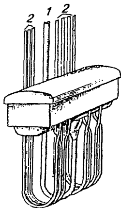
Рис.10.7. Выкладка абонентских проводов на вводе в распределительную коробку
