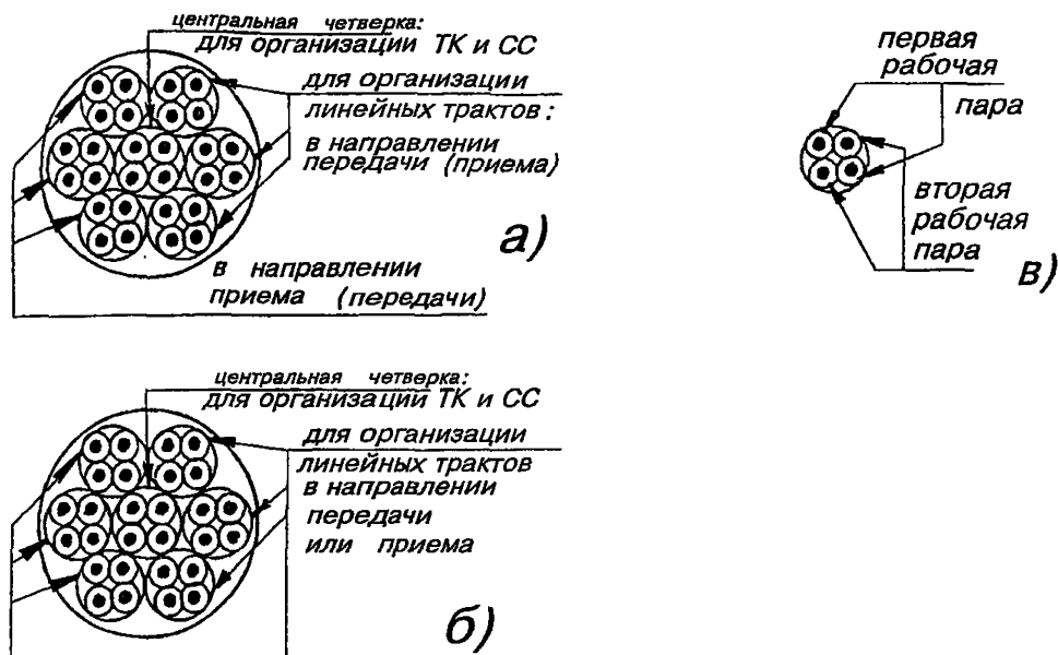
Рис.13.7. Назначение четверок в кабеле МКС 7х4х1,2:
