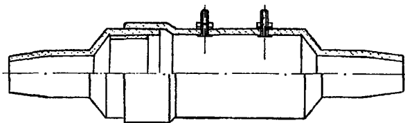
Рис. 11.33. Полиэтиленовая соединительная муфта типа МПС, используемая в качестве газонепроницаемой
