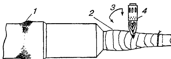
Рис.11.24. Наплавление полиэтиленовой ленты под стеклолентой:
