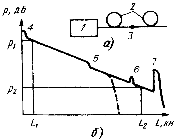
Рис.15.2. Измерение затухания методом обратного рассеяния:
