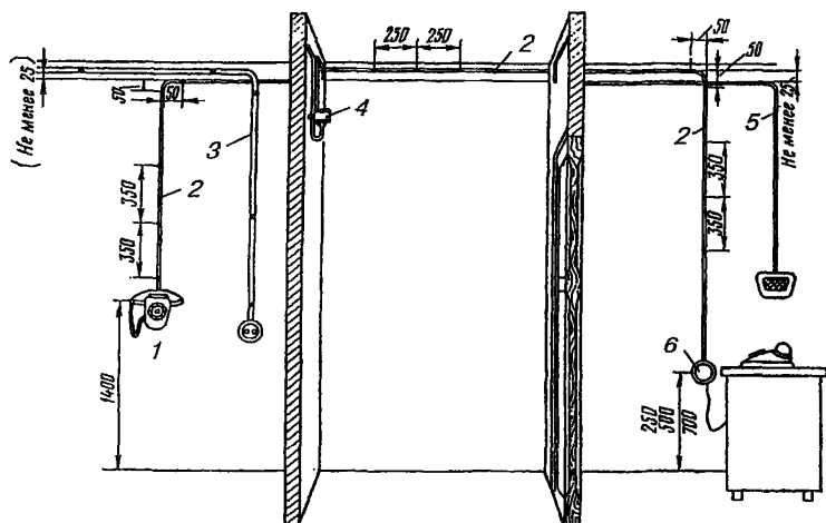
Рис.10.10. Виды абонентских проводок:
