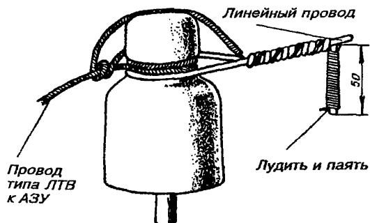
Рис.10.5. Соединение провода ЛТВ-В (ЛТР-В) с линейным проводом
