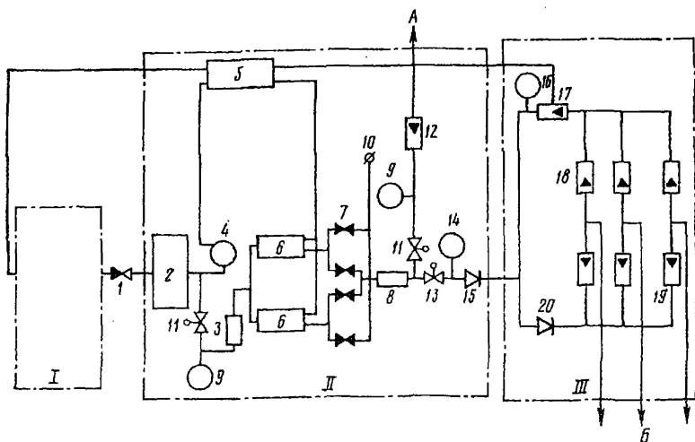
Рис.16.2. Функциональная схема КСУ-2М:
