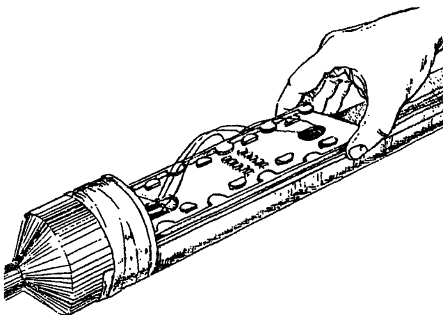
Рис.12.4. Установка кассеты на каркас
