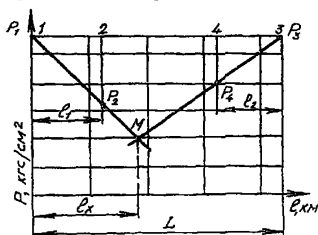
Рис. 16.4. График распределения давления в кабеле
