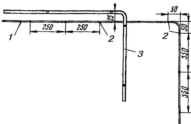
Рис.10.8. Прокладка однопарного провода абонентской проводки:
