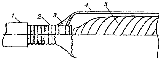
Рис.11.27. Восстановление стальных гофрированных оболочек городских телефонных кабелей:
