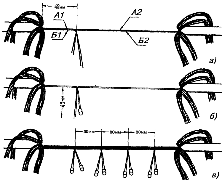
Рис.11.19. Сращивание жил при помощи одножильных соединителей
