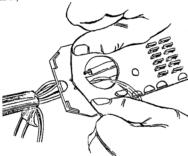
Рис.12.13. Установка кассеты и вывод волокон через окно кассеты
