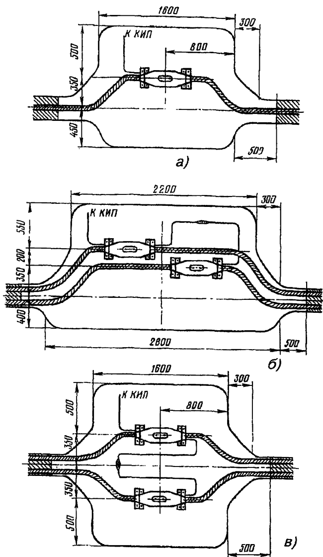
Рис.11.4. Расположение муфт в котлованах:
