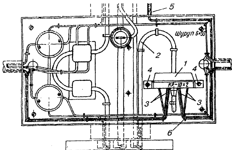
Рис.10.6. Размещение распределительных устройств: телефонных и проводного вещания в нише лестничной клетки:
