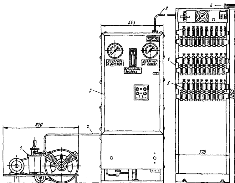
Рис.16.1. Компрессорно-сигнальная установка КСУ-2М:
