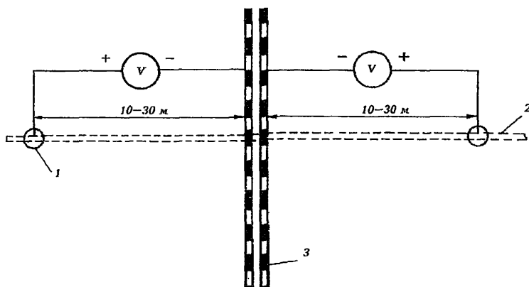
Рис.17.5. Схема измерения разности потенциалов между кабелем и рельсами на участке пересечения:
