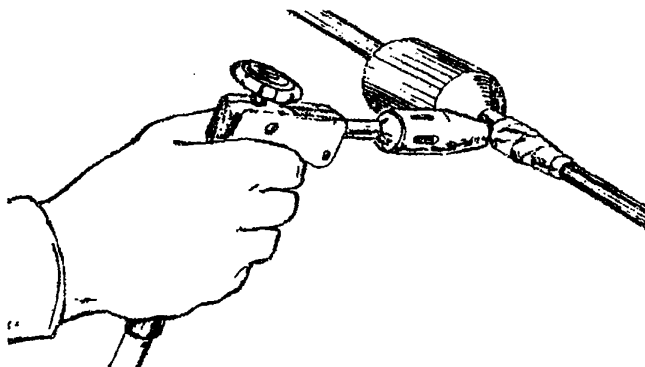
Рис.12.2. Наплавление полиэтиленовой ленты под стеклолентой на стыке конуса с оболочкой кабеля
