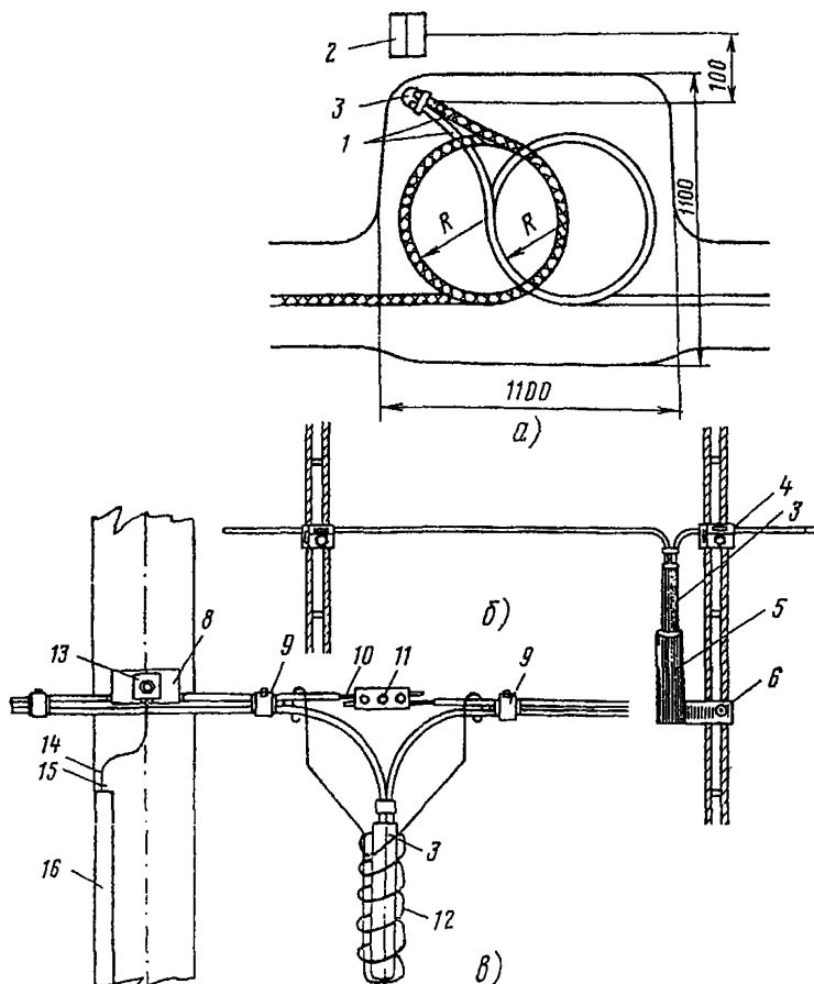
Рис.11.60. Размещение тупиковых муфт:
