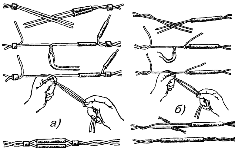
Рис.11.10. Процесс сращивания жил ручной скруткой: а) с изолированием индивидуальными гильзами; б) с изолированием общей гильзой
