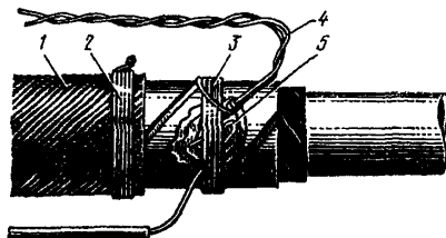
Рис.11.7. Наложение бандажей и устройство перемычек:
