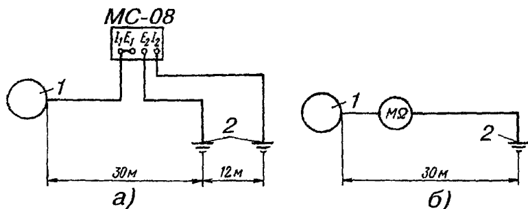
Рис. 17.7. Схема измерения сопротивления изоляции корпусов НУП:
