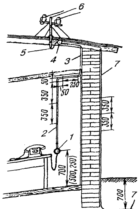
Рис.10.4. Абонентский пункт с воздушным вводом со стойки через чердачное перекрытие
