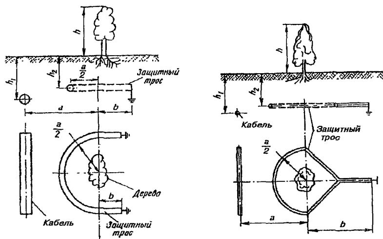
Рис.18.1. Схемы для перехвата токов молнии, попавших в дерево, с помощью защитного троса, проложенного в земле между кабелем и деревом:
