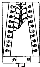
Рис.11.40. Ввод и включение кабеля в распределительную коробку типа КРО 10х2
