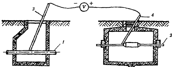
Рис. 17.6. Схема измерения разности потенциалов между кабелем и соседним подземным металлическим сооружением:
