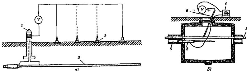
Рис. 17.4. Схема измерения разности потенциалов оболочек кабелей относительно земли по методу выноса электрода:
