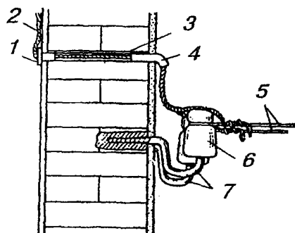
Рис.10.1. Устройство абонентского ввода с воздушной столбовой линии через кирпичную стену:
