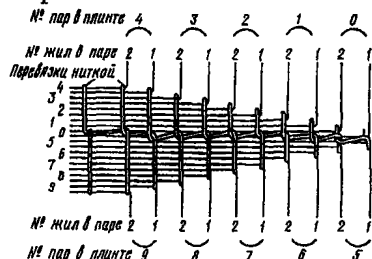
Рис.11.46. Схема расшивки жил на плинт бокса
