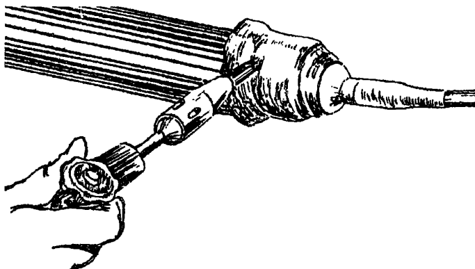
Рис.12.9. Усадка пояска ТУТ 100/50 на стыке цилиндрической части муфты с конусом
