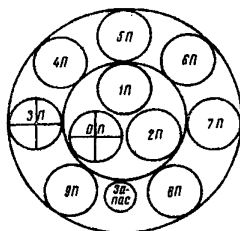
Рис.11.42. Распределение жил по плитам боксов: а) при нумерации по схеме 10.72; б) при нумерации по схеме 10.73
