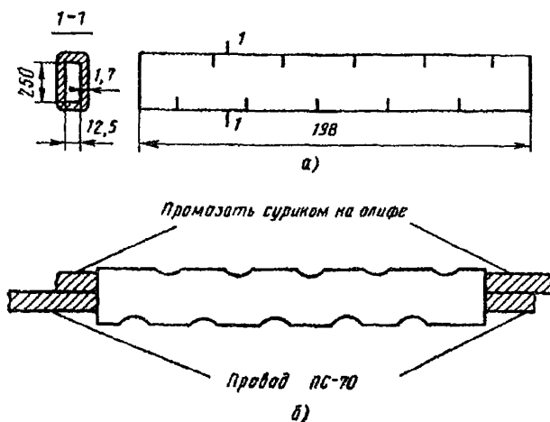
Рис.18.2. Сращивание защитных проводов ПС-70 с помощью овальных соединителей:
