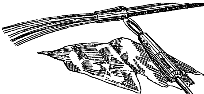
Рис.12.11. Продольная герметизация кабеля термоусаживаемой трубкой
