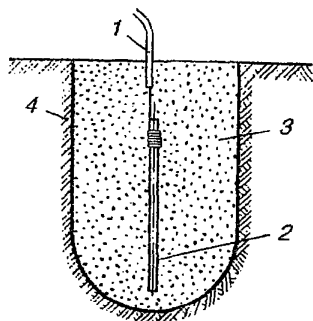
Рис.18.14. Устройство заземлителя в грунте с высоким удельным сопротивлением
