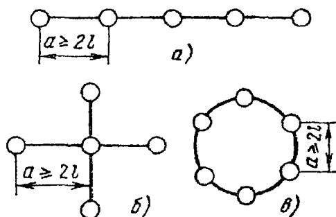
Рис.18.9. Расположение электродов заземления:
