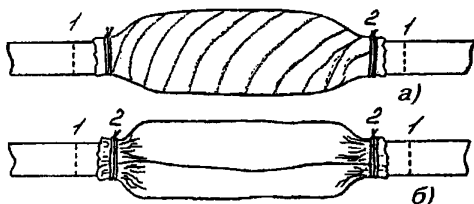
Рис.11.20. Восстановление поясной изоляции на кабелях типа Т: а) миткалевой лентой; б) кабельной бумагой
