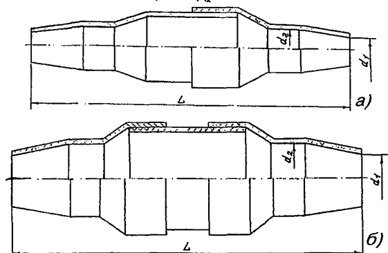
Рис. 11.36. Муфты газонепроницаемые малогабаритные МГНМс:
