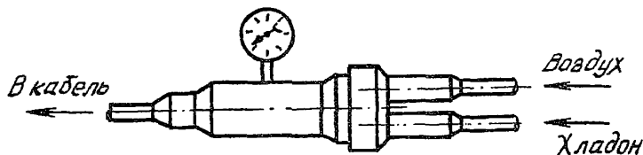
Рис. 16.5. Камера для смешивания хладона с воздухом (свинцовая разветвительная муфта)
