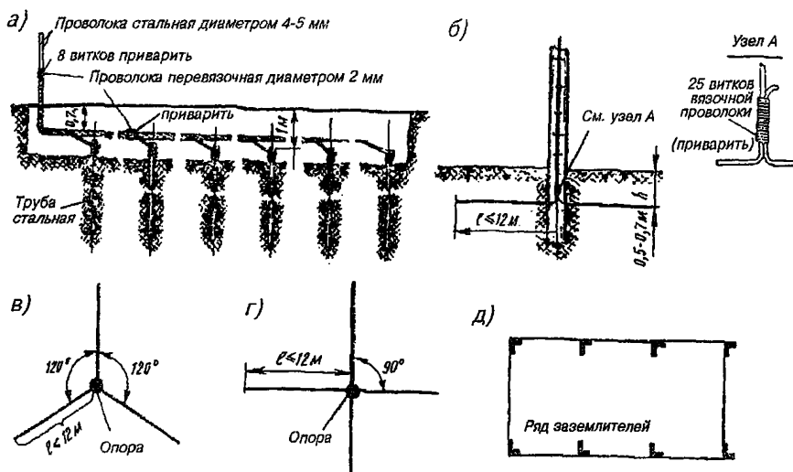
Рис.18.10. Многоэлектродные заземлители:
