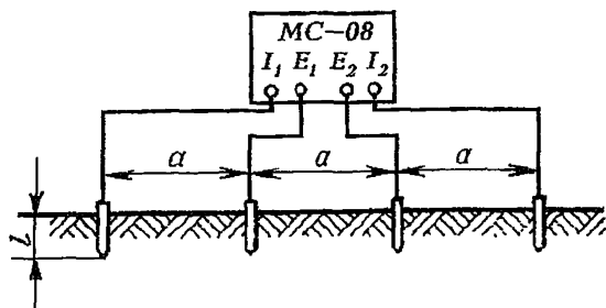
Рис. 17.1. Схема измерения удельного сопротивления земли прибором МС-08: a — расстояние между электродами, l — глубина забивки стержней
