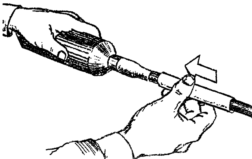
Рис.12.3. Установка пояска ТУТ 30/15 на стык конуса с оболочкой кабеля
