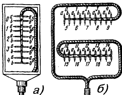
Рис.11.47. Расшивка кабеля и порядок включения жил на плиты кабельных ящиков:
