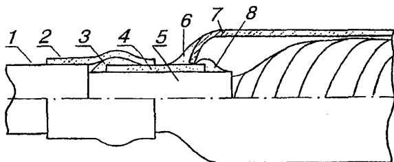
Рис.11.28. Восстановление алюминиевой оболочки кабеля ГТС:
