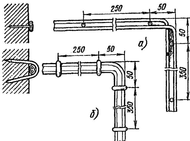
Рис.10.9. Способы крепления провода ТРП (ТРВ):
