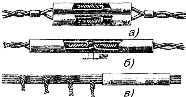
Рис.11.11. Способы изолирования скруток жил:
