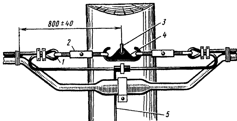
Рис.11.38. Размещение муфты подвешенного кабеля с встроенным стальным канатом:
