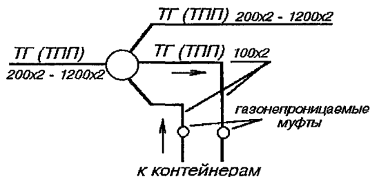
Рис.13.3. Схема выпайки кабелей 100 \times 2 из кабеля большей емкости
