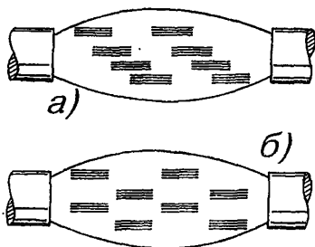
Рис.11.12. Размещение скруток жил по длине муфты:
