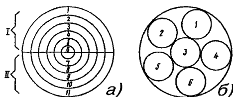
Рис.11.8. Очередность монтажа групп жил сердечника:
