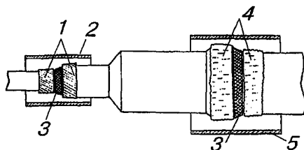
Рис.11.25. Расположение поясков сэвильеновой ленты и слоев клея-расплава на полиэтиленовой муфте:
