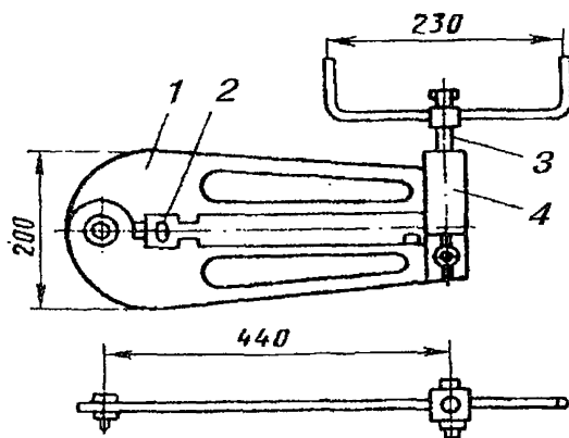
Рис.18.3. Клещи типа МИ-31 для обжатия овальных соединителей:
