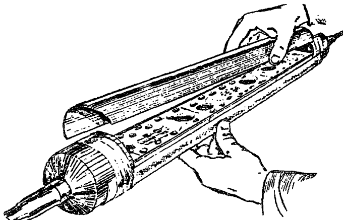
Рис.12.8. Установка второй половины каркаса
