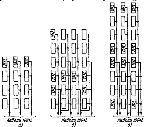
Рис.11.48.Расшивка кабелей 100х2 на защитные полосы 25х2:
