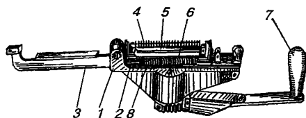
Рис.11.14. Ручная пресс-техника ПСМЖ-200:
