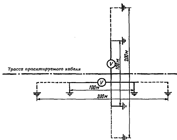
Рис. 17.2. Схема определения блуждающих токов в земле
