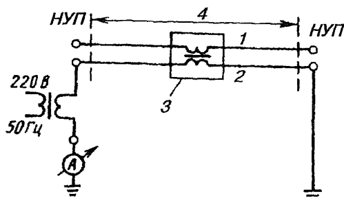
Рис.18.5. Схема измерения тока после монтажа РТ:
