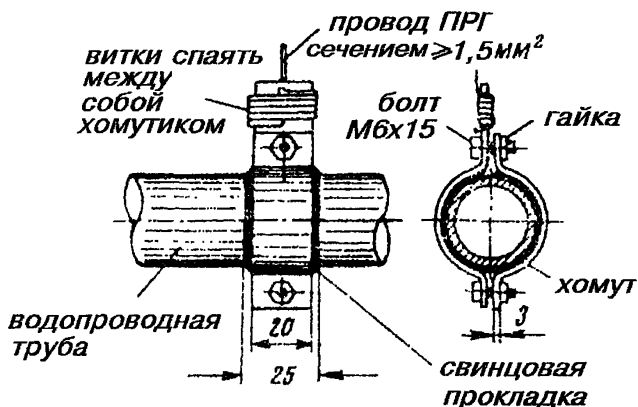
Рис.18.12. Устройство заземления с использованием в качестве заземлителя водопроводной трубы
