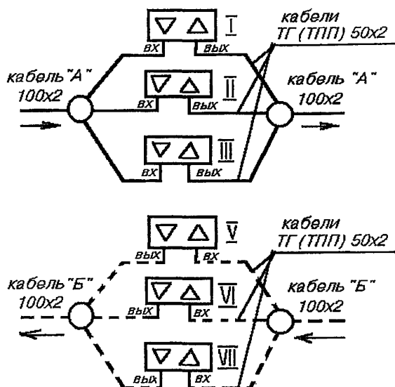
Рис.13.2. Схема распаики кабелей при двухкабельном двухконтейнерном варианте
