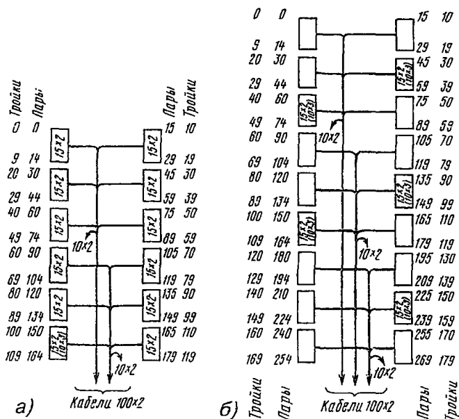
Рис.11.51. Расшивка кабелей 100x2 на рамки 15x2 (10x3):
