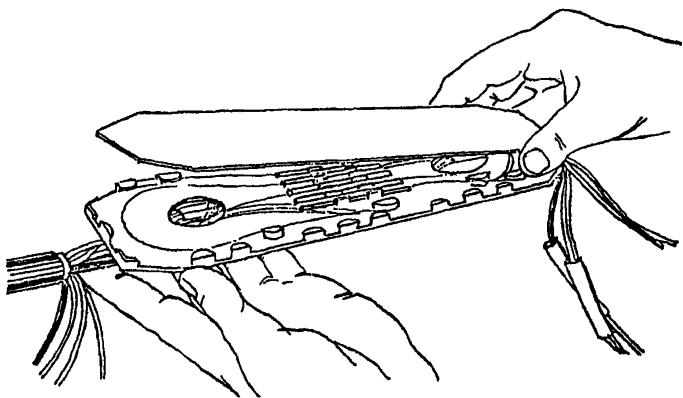
Рис.12.14. Установка крышки на кассету
