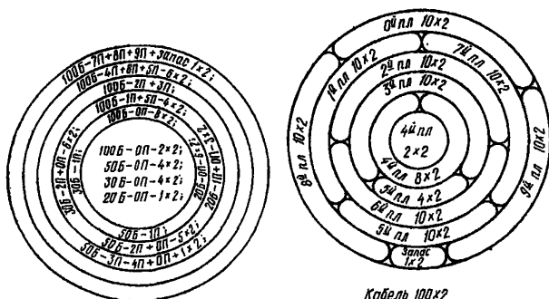
Рис.11.42. Распределение жил по плитам боксов: а) при нумерации по схеме 10.72; б) при нумерации по схеме 10.73
