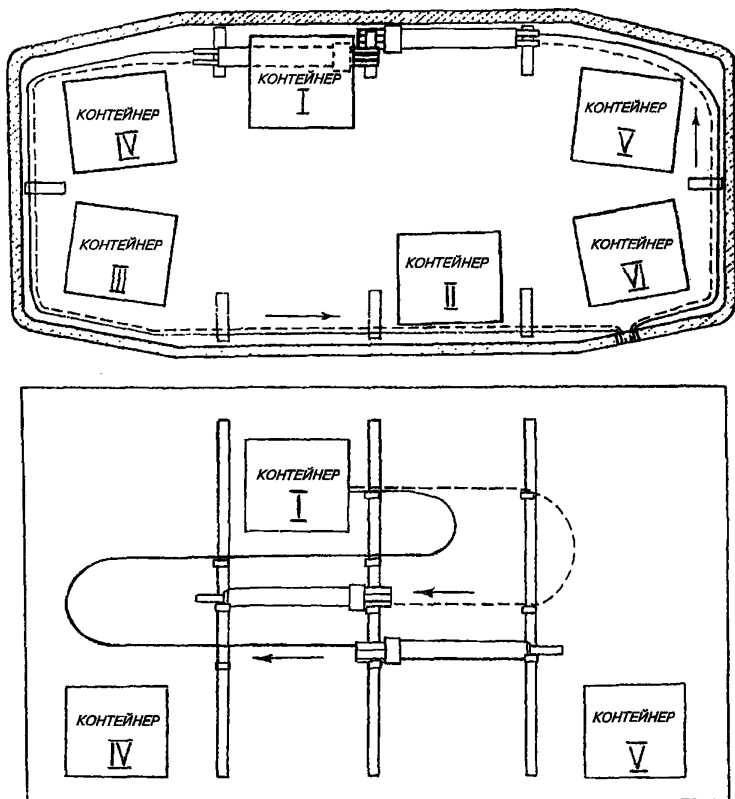
Рис.13.1. Схема расположения кабеля и муфт в колодце ККС-5
