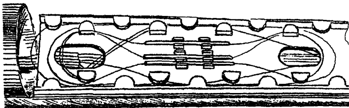
Рис.12.7. Укладка трех соединенных оптических волокон и защитных гильз КДЗС в кассете
