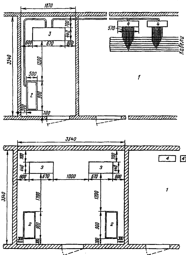
Рис.16.3. Размещение КСУ-2М:
