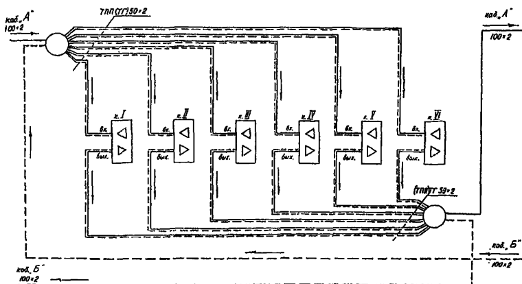
Рис.13.4. Схема распайки кабелей при двухкабельном одноконтейнерном варианте
