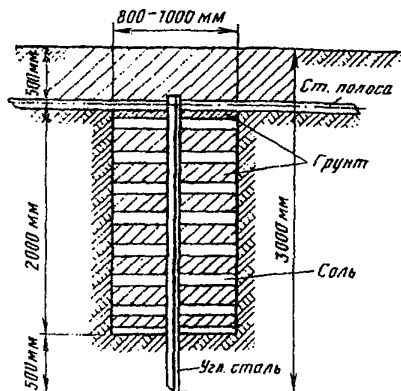
Рис.18.13. Конструкция котлована при обработке грунта солью для установки заземлителя из угловой стали
