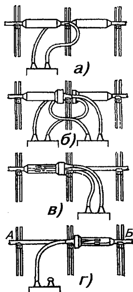
Рис.11.53. Соединение пупиновских ящиков с линейными кабелями:
