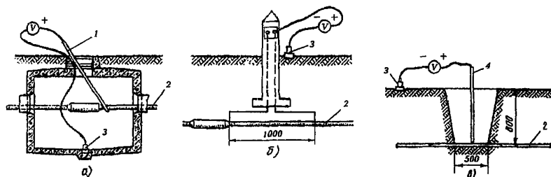
Рис. 17.3. Схема измерения разности потенциалов оболочек кабеля относительно земли:
