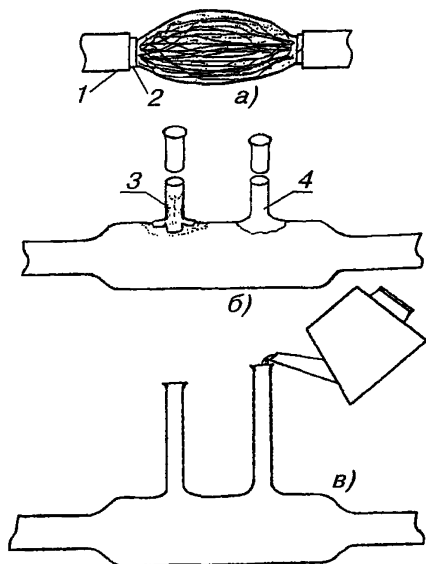
Рис.11.34. Монтаж ГНМ на кабеле типа Т:
