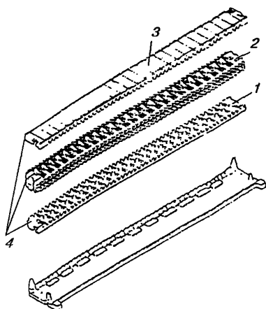
Рис. 11.16. Конструкция модуля MS:
