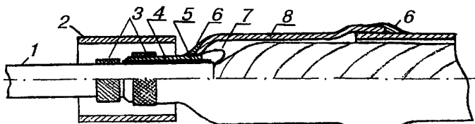
Рис.11.26. Монтаж переходной манжеты и свинцовой муфты на стыке кабелей в свинцовой и полиэтиленовой оболочках:
