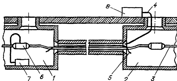
Рис.16.6. Определение места негерметичности оболочки кабеля в пролете канализации с помощью киперной ленты:
