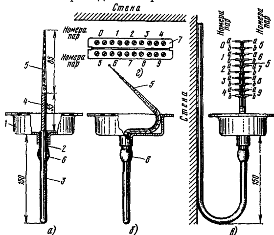
Рис.11.41. Примерные размеры разделки кабеля и порядок включения жил в распределительную коробку 10х2 КРТ, КРТП:
