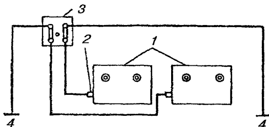
Рис. 18.4. Схема включения протектора для защиты корпуса РТ от коррозии:
