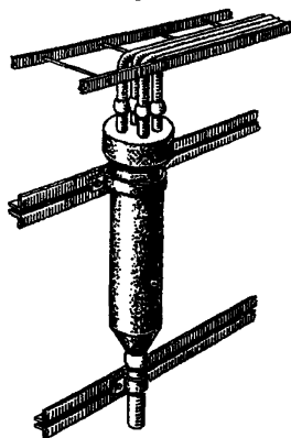
Рис.11.2. Крепление вертикальных станционных разветвительных муфт к каркасу
