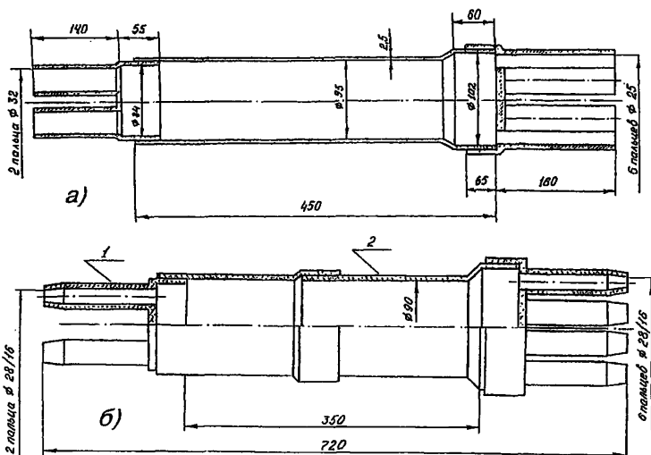
Рис.13.5. Разветвительные муфты:
