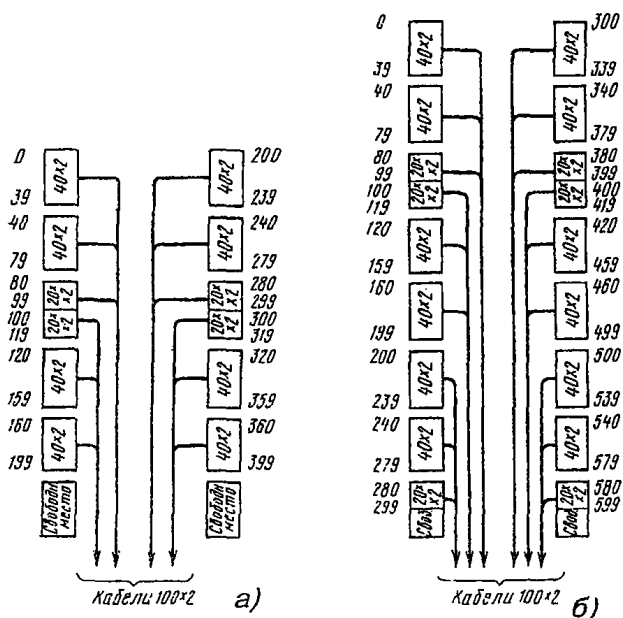
Рис.11.50. Расшивка кабелей 100x2 на рамки 40x2:
