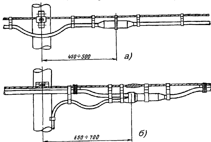
Рис. 11.3. Размещение муфт на подвесных кабелях: а) соединительных; б) разветвительных
