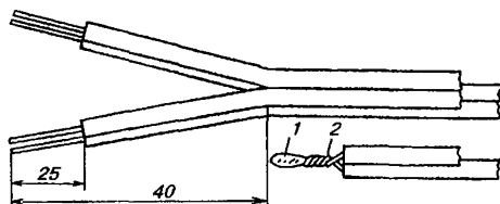
Рис.11.61. Разделка и соединение жил кабеля ПРППМ (ПРВПМ):
