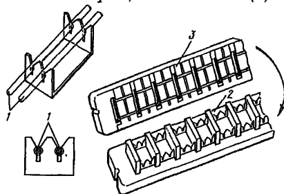
Рис.11.13. Соединитель СМЖ-10:
