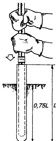
Рис.11.59. Установка муфты и погружение сrostка в нее
