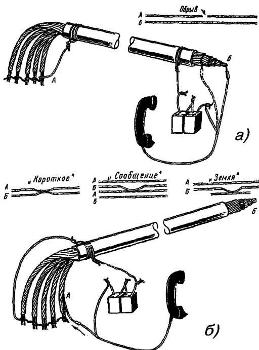
Рис.11.5. Проверка жил кабеля: а) на "обрыв"; б) на "сообщение"
