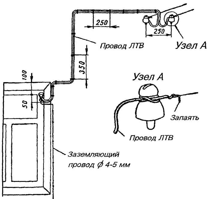
Рис.10.2. Устройство абонентского ввода с воздушной столбовой линии через окно
