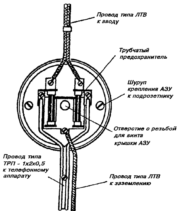
Рис.10.3. Монтаж АЗУ
