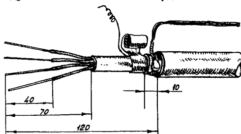
Рис.11.54. Разделка концов кабеля КСПБ
