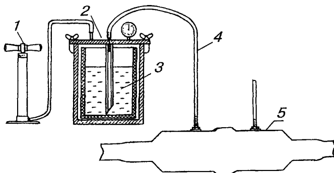
Рис.11.35. Заливка ГМ на кабеле типа ТП:
