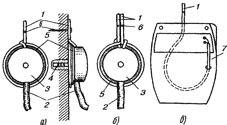
Рис.10.11. Способы включения однопарного провода в розетки телефонных аппаратов:
