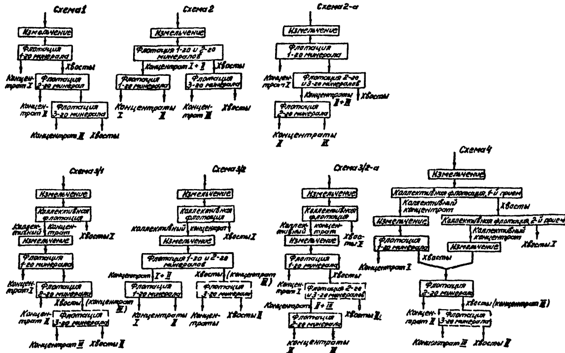
Рис. 7 Принципиальные схемы флотации полиметаллических руд содержащих при плавных компонентах
