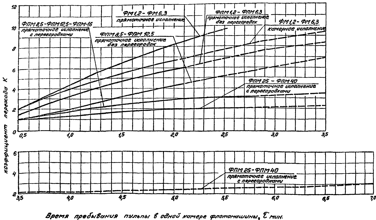
Рис. 8 Зависимость K от T для флотационных машин различных типов
