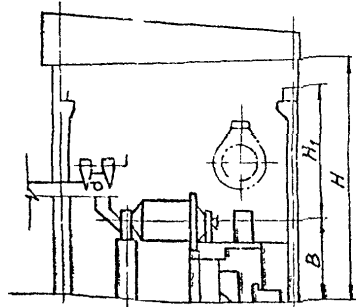
Разрез 1-1
