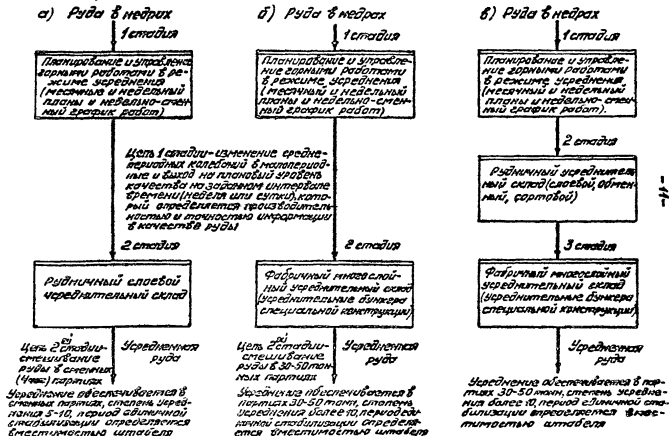
Рис. 2 Принципиальные схемы усреднения руды для дальнейшего усреднения
