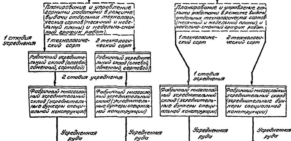
Рис. 1 Принципиальные схемы ускорения руды для внутрисортowego усреднения
