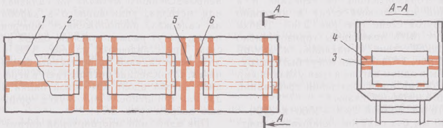
Рис. 3.71: 1—салазки; 2—листовой металл в пачках; 3—прокладка; 4—упорный брусок; 5—продольный упорный брусок; 6—соединительная планка
