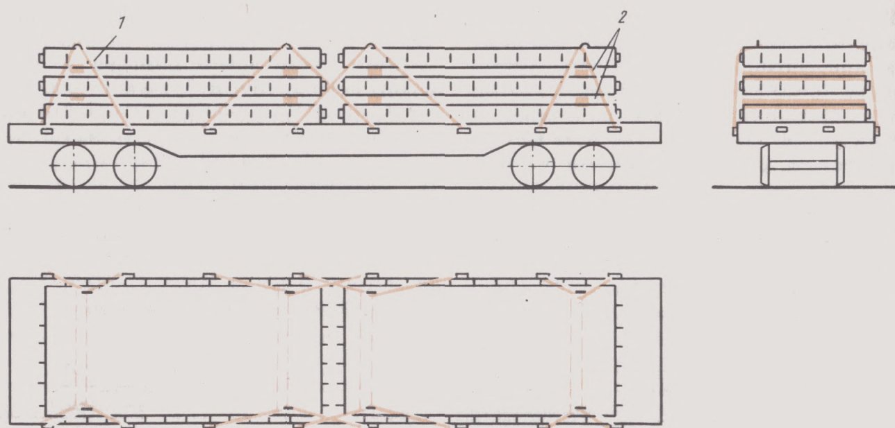
Рис. 4.10: 1—растяжка; 2—прокладка
