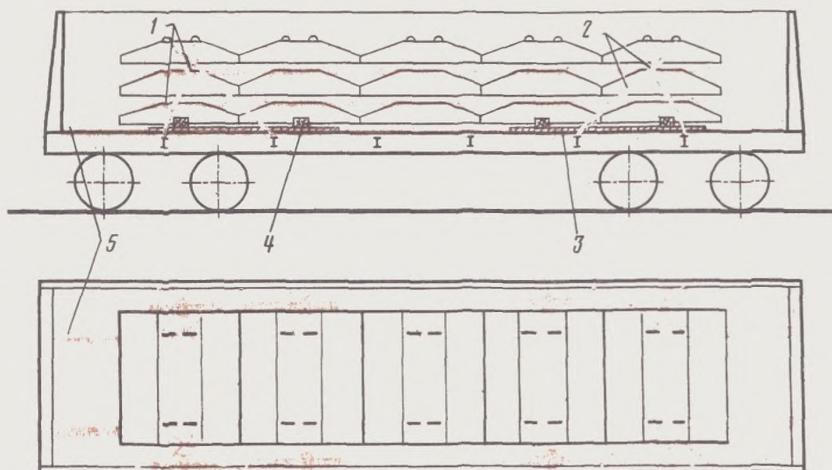
Рис. 4.42: 1—прокладки; 2—растяжки; 3—специальная подкладка упорных брусков; 4—поперечный упорный брусок; 5—подкладки
