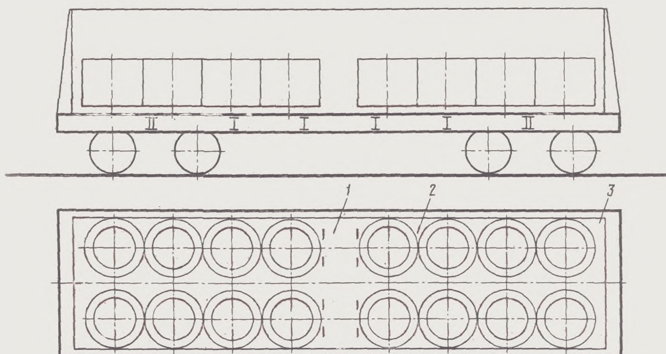
Рис. 3.132: 1—распорные бруски; 2—подкладки; 3—поперечные упорные бруски
