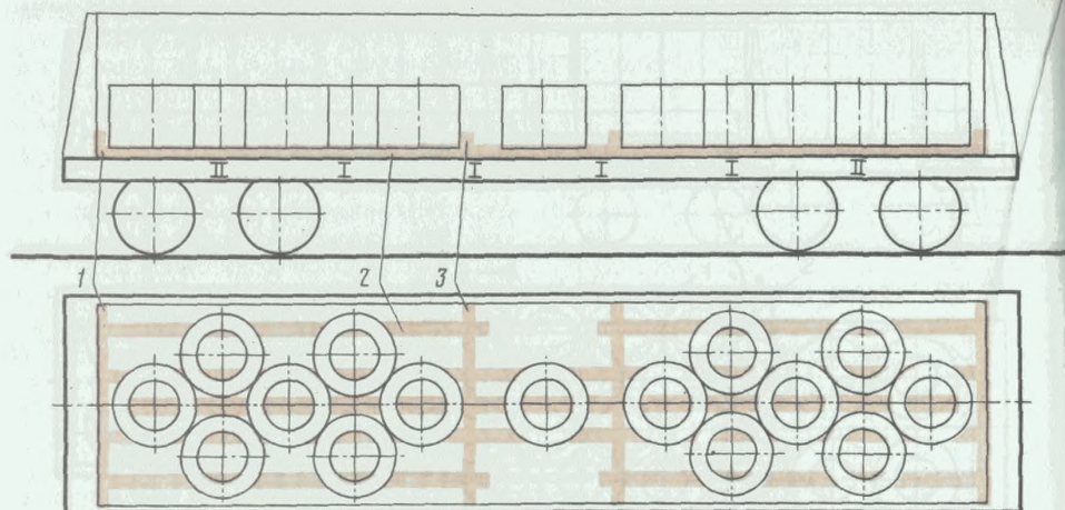
Рис. 3. 133: 1—упорный брус; 2—подкладки; 3—скрепляющая планка
