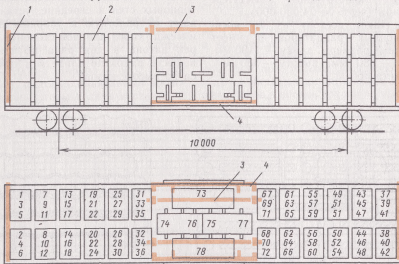
Рис. 39 (III): 1—рама упорная; 2—транспортный пакет из 13 радиаторов; 3—распорка; 4—рама-упор
