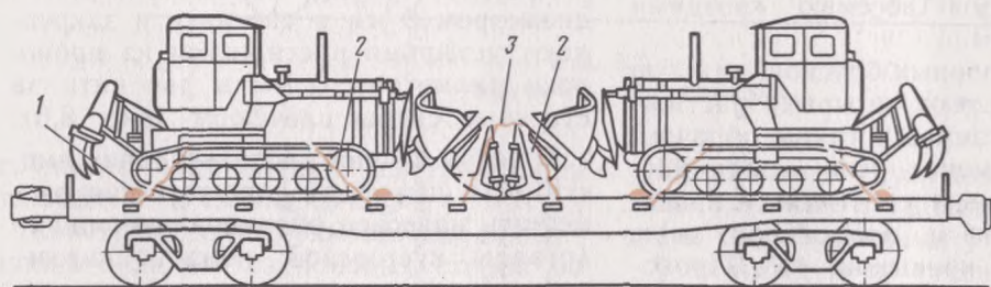
Рис. 8.6: 1—упорные бруски; 2—растяжки; 3—увязки
