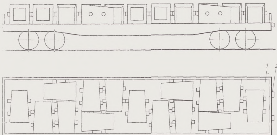
Рис. 3.120: 1—упорный брус; 2—распорный брус
