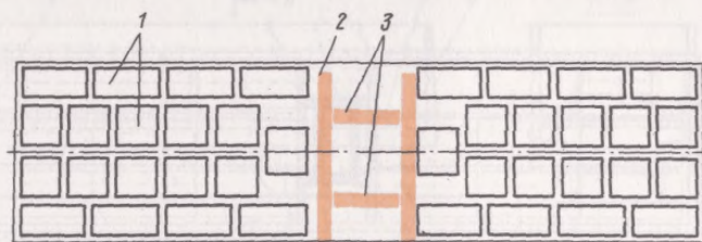
Рис. 3.50: 1—пачки листового металла; 2—упорные бруски; 3—распорные бруски
