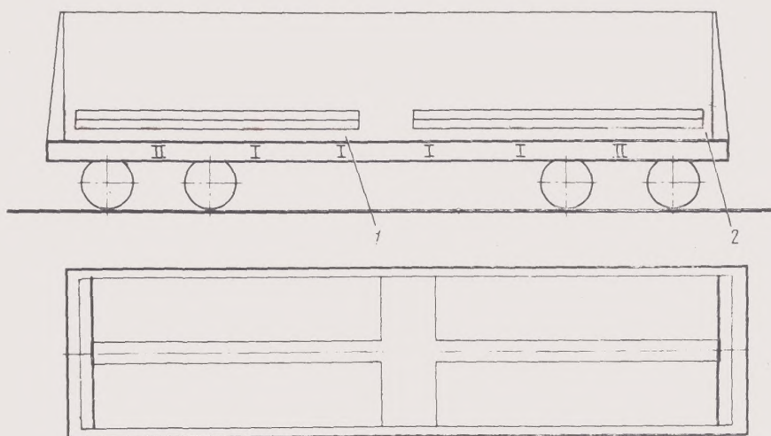
Рис. 3.103: 1—подкладки; 2—торцовый щит
