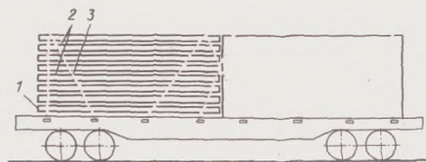
Рис. 4.7: 1—подкладка; 2—прокладка; 3—растяжка
