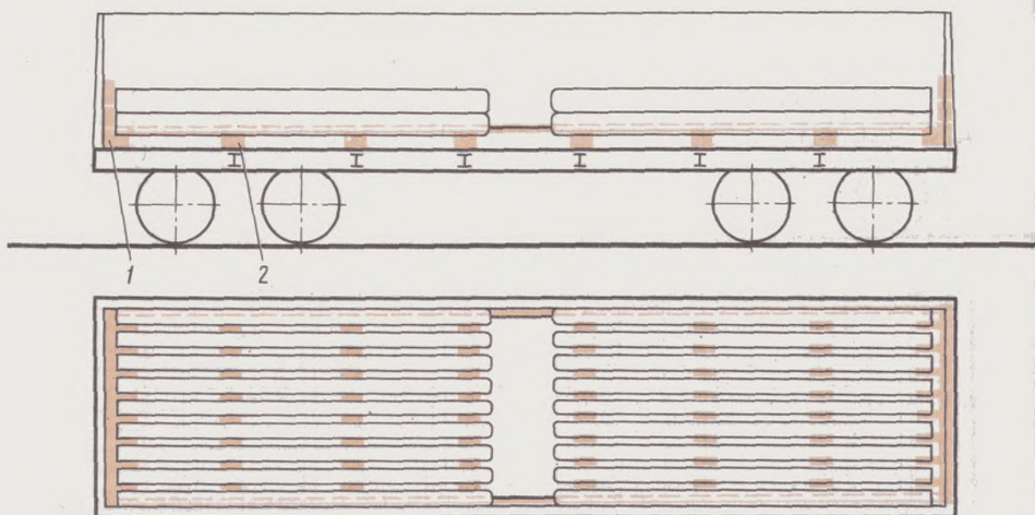
Рис. 3.115: 1—доски торцового ограждения; 2—подкладки
