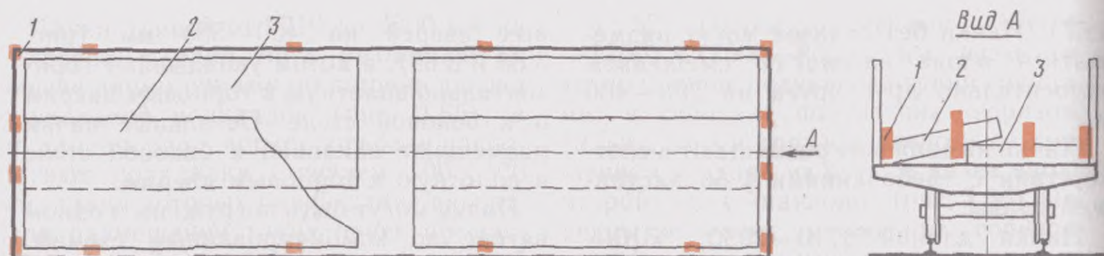
Рис. 3.70: 1—вертикальные бруски; 2, 3—пачки листового металла, уложенного соответственно наклонно и горизонтально
