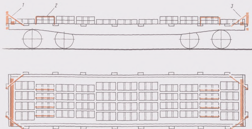
Рис. 3.41: 1—растяжка; 2—обвязка пачек; 3—торцовые стойки
