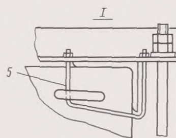
Рис. 4.22: 1—опорно-крепежное устройство (исполнение 1); 2—подкладка; 3—прокладка; 4—проволочная скрутка; 5—хомут
