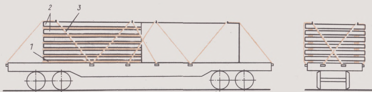
Рис. 4.11: 1—подкладка; 2—прокладка; 3—растяжка
