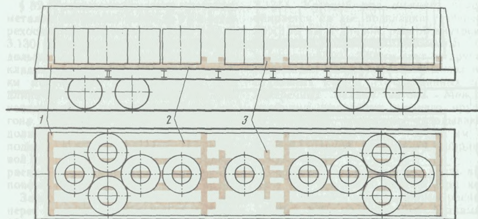
Рис. 3.134: 1—упорный брус; 2—подкладки; 3—скрепляющие планки
