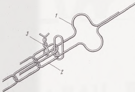
Рис. 2.34: 1—замок с переменным зевом; 2—цепной замок; 3—проволочная закрутка
