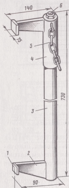
Рис. 38 (III): 1—пята; 2—косынка; 3— опорный стакан; 4—ста- кан; 5—цепная петля; 6—болт
