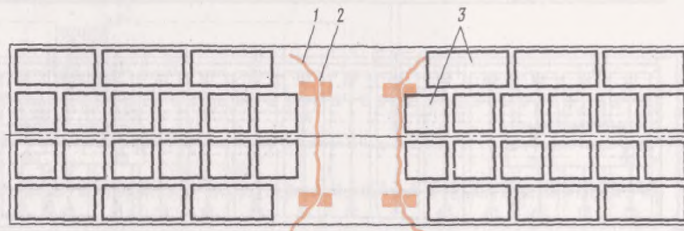
Рис. 3.51: 1—проволочная увязка; 2—брусок; 3—пачки листового металла
