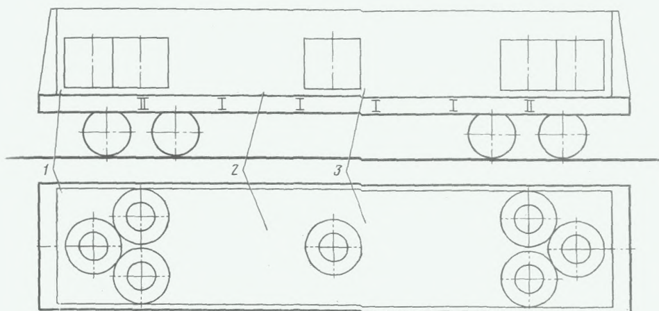
Рис. 3.135; 1—упорный брус; 2—подкладки; 3—скрепляющие планки
