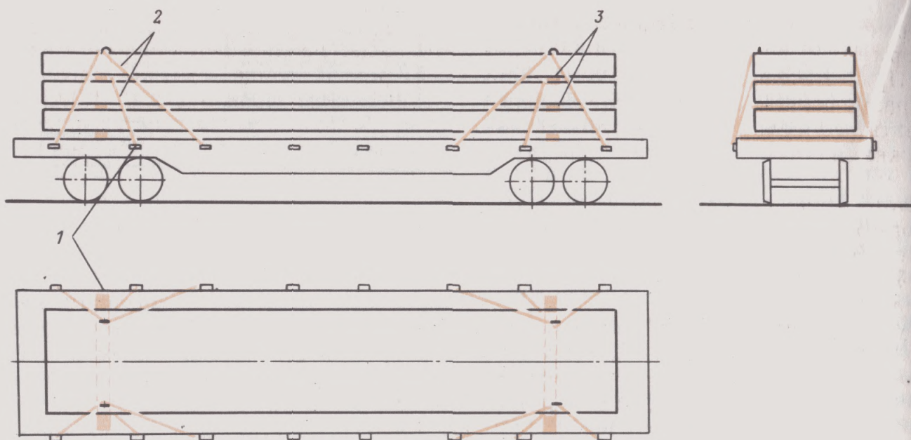
Рис. 4.9: 1—подкладка; 2—растяжка; 3—прокладка
