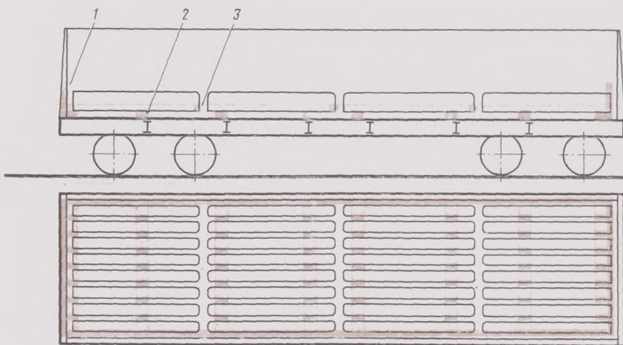
Рис. 3.118: 1—доски торцового ограждения; 2, 3—подкладки
