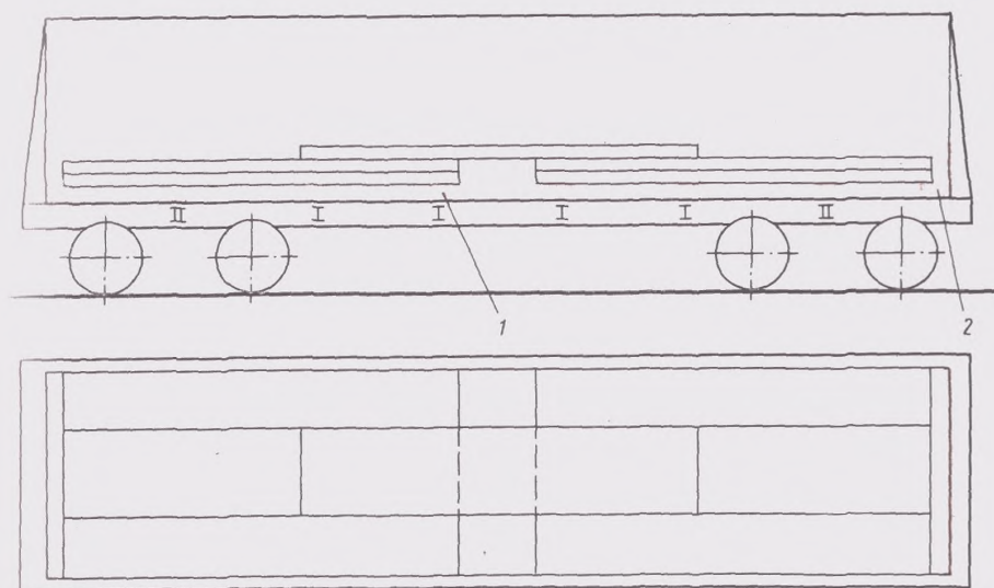
Рис. 3.105: 1—подкладки; 2—торцовый щит
