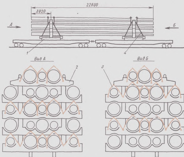
Рис. 10.28: 1—турникет; 2—бандаж; 3—обвязка; 4—растяжка
