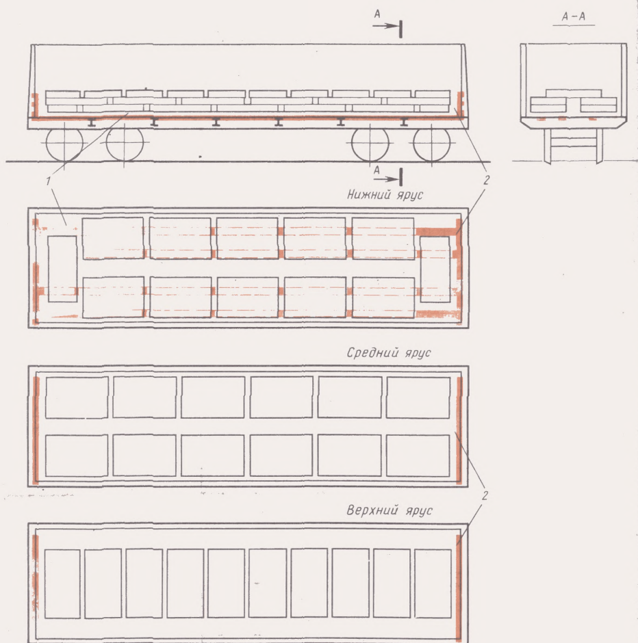
Рис. 3.92: 1—подкладки; 2—щит
