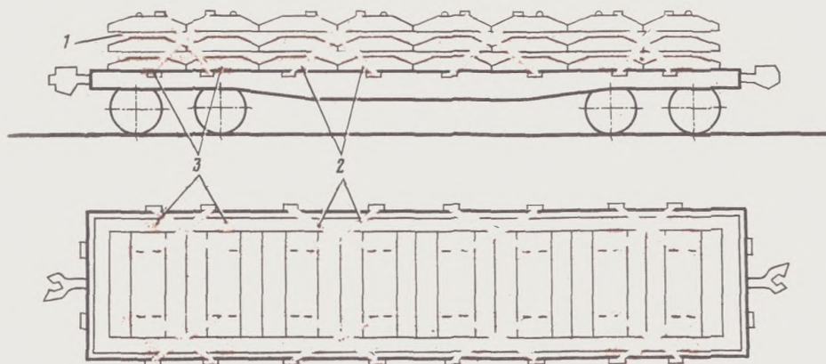
Рис. 4.41: 1—прокладка; 2—растяжка; 3—поперечные упорные бруски
