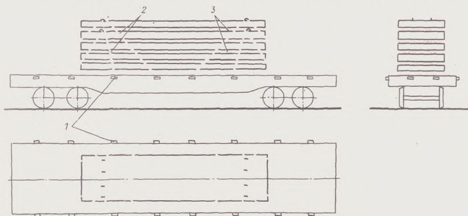
Рис. 4.8: 1—подкладка; 2—растяжка; 3—прокладка
