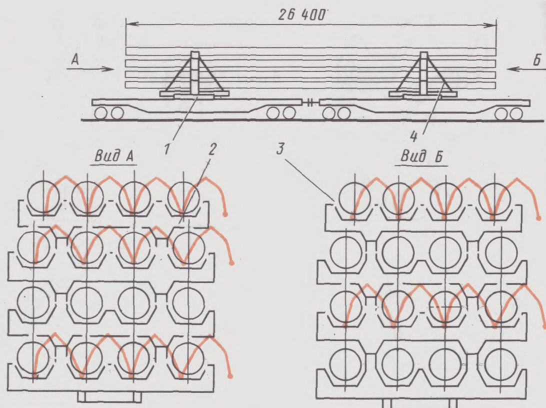
Рис. 10.25: 1—турникет; 2—бандаж; 3—обвязка; 4—растяжка
