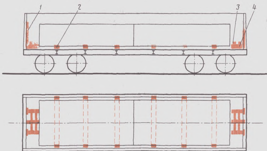
Рис. 3.90: 1—вертикальные бруски; 2—подкладки; 3—соединительные планки; 4—распорные бруски
