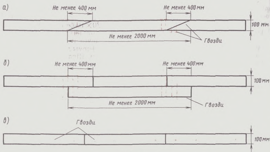
Рис. 4.1: а, б—составные продольные подкладки в полувагоне; в—на платформе
