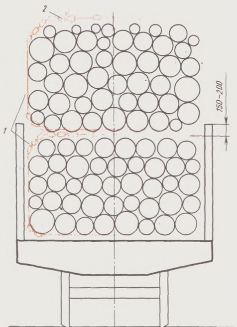
Рис. 2.65: 1—стропы ПС-05; 2—проволочная закрутка
