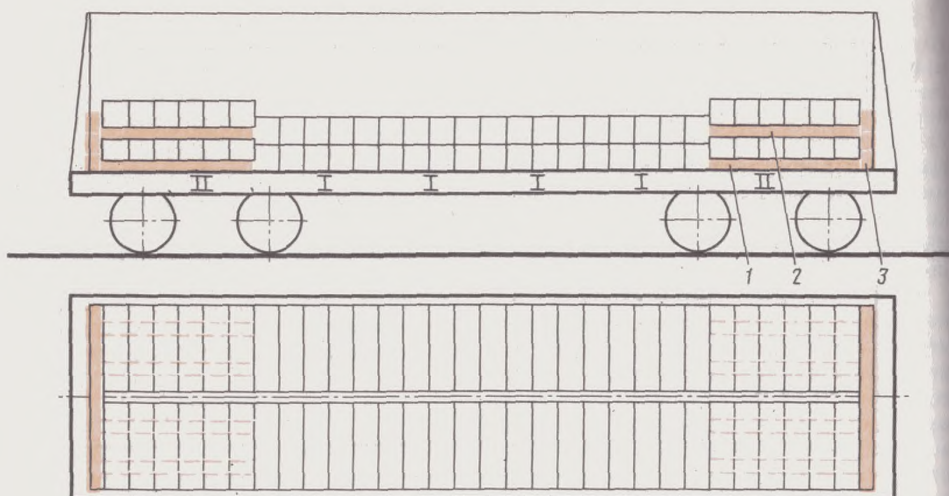
Рис. 3.114: 1—подкладки; 2—прокладки; 3—торцовые ограждения
