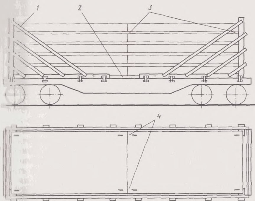
Рис. 4.21: 1—опорно-крепежное устройство (исполнение 1); 2—подкладка; 3—прокладка; 4—проволочная скрутка
