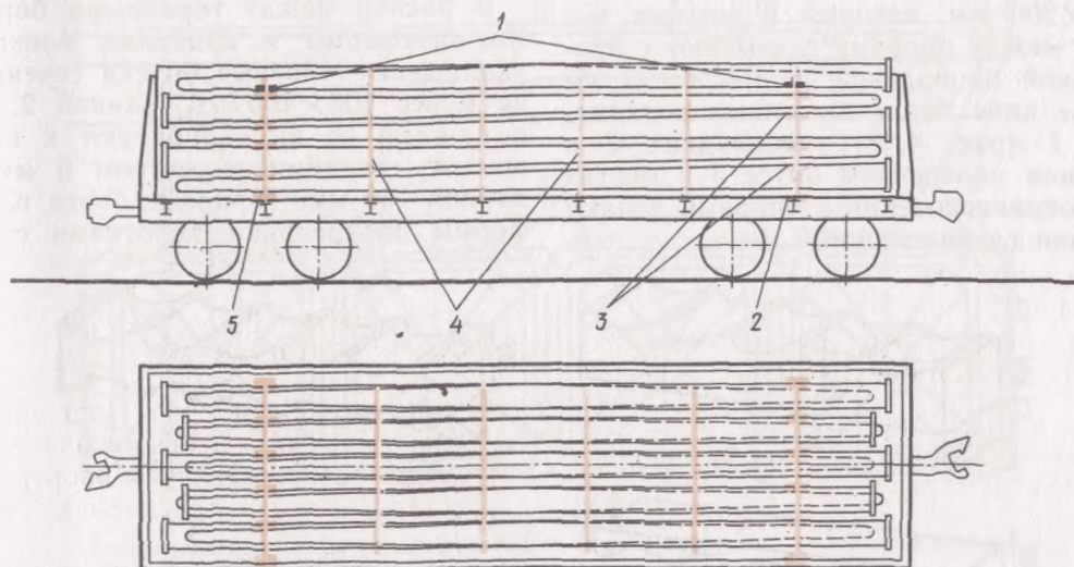
Рис. 4.46: 1—клинья; 2—подкладка; 3—прокладка; 4—обвязка; 5—утолщенная подкладка
