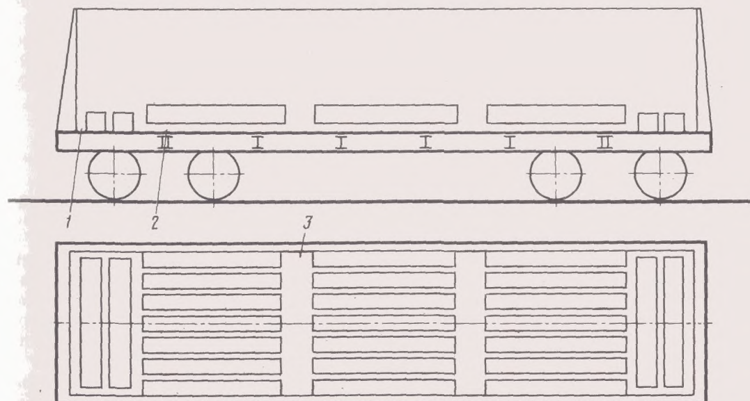
Рис. 3.117: 1—доски торцового ограждения; 2, 3—подкладки
