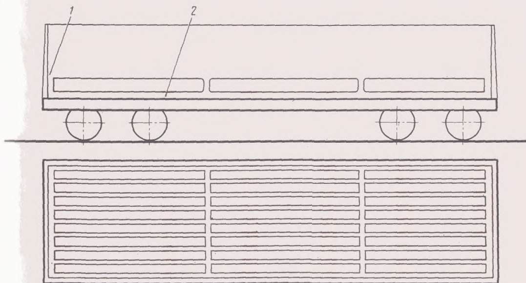
Рис. 3.116: 1—доски торцового ограждения; 2—подкладки
