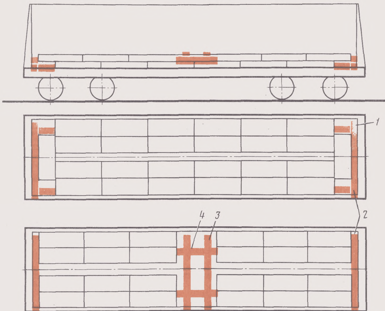
Рис. 3.100: 1—продольные упорные бруски; 2—поперечные бруски сечением 100×150 мм; 3—соединительные планки; 4—распорные бруски
