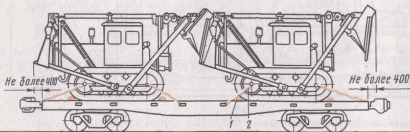
Рис. 8.8: 1—упорные бруски; 2—растяжки
