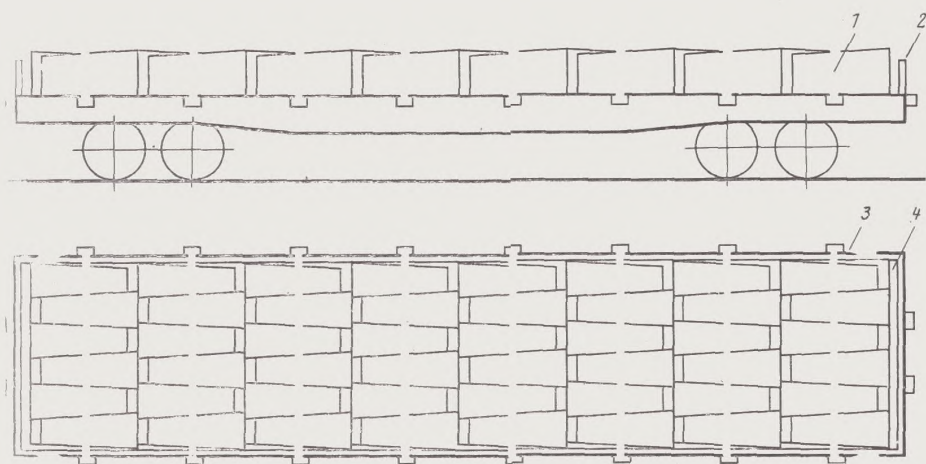
Рис. 3.119: 1—обвязка из проволоки; 2—торцовая стойка; 3—увязка; 4—упорный брус
