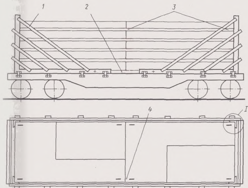
Рис. 4.22: 1—опорно-крепежное устройство (исполнение 1); 2—подкладка; 3—прокладка; 4—проволочная скрутка; 5—хомут
