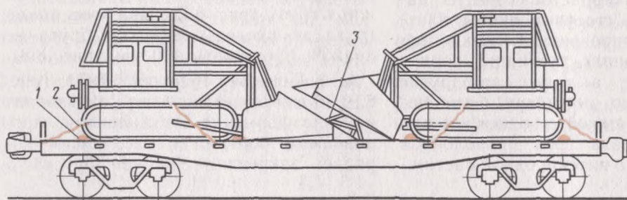
Рис. 8.7: 1—упорные бруски; 2—растяжки; 3—специальные подставки
