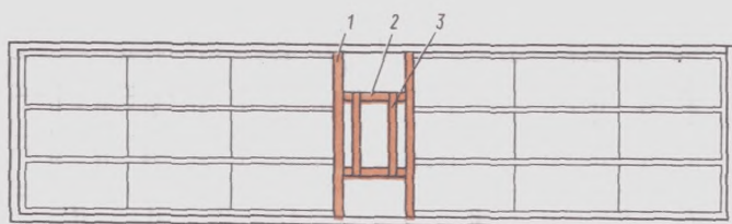
Рис. 3.52: 1—упорные бруски; 2—распорные бруски; 3—соединительные планки
