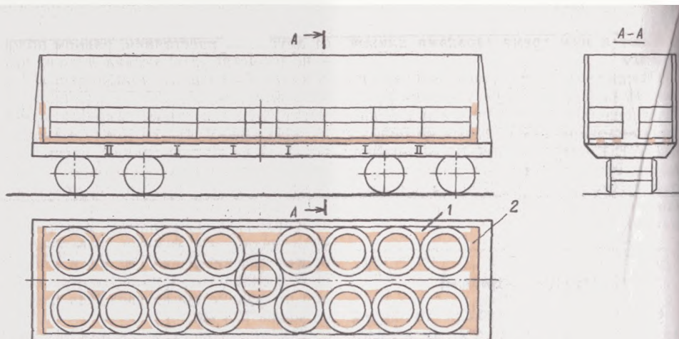
Рис. 3.130: 1—подкладки; 2—поперечные упорные бруски
