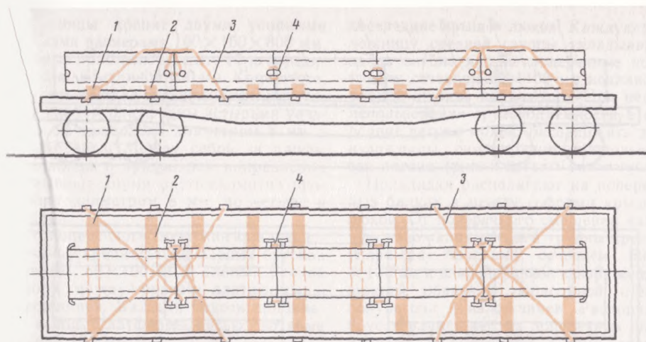
Рис. 3.123: 1—подкладки; 2—поперечные упорные бруски; 3—растяжки; 4—увязка изложниц
