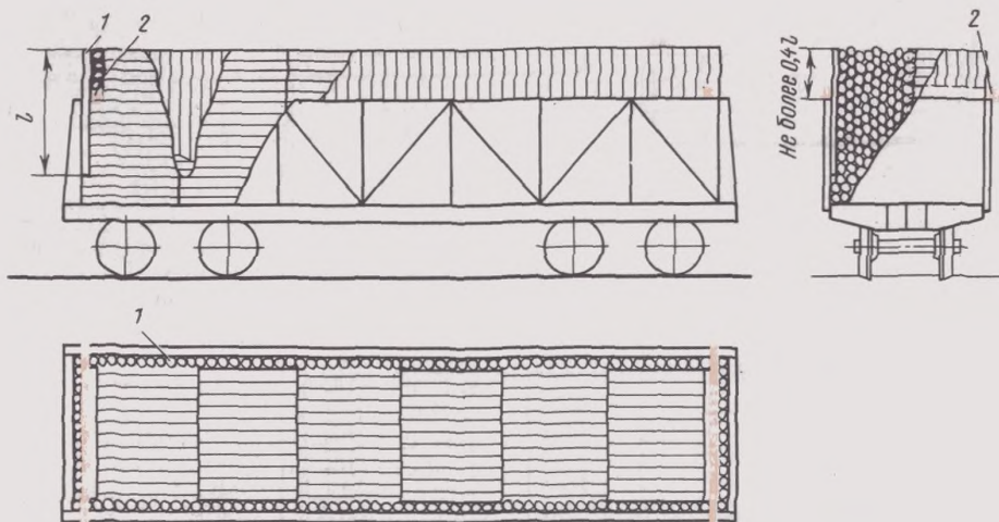
Рис. 2.24: 1—оторцовка; 2—доски, скрепляющие оторцовку
