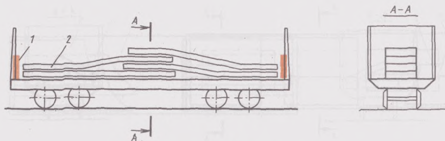
Рис. 3.72: 1—вертикальные бруски; 2—листовой металл в пачках
