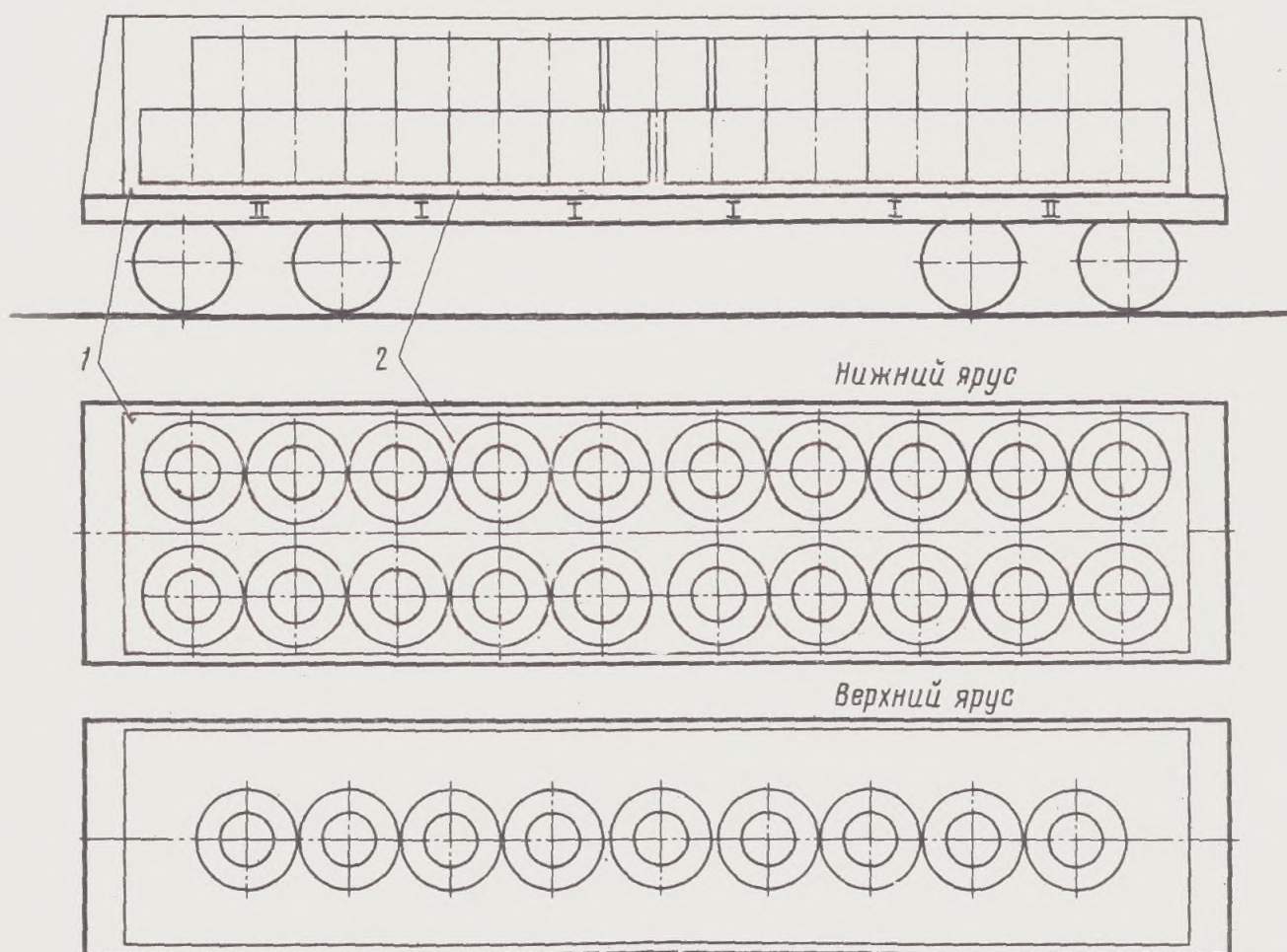
Рис. 3.131: 1—упорный брус; 2—подкладки
