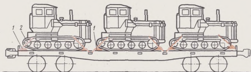
Рис. 8.2: 1—упорные бруски; 2—растяжки
