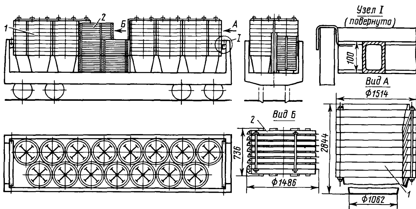
Рис 9 18 1—пакет контейнеров, 2—пакет крышек
