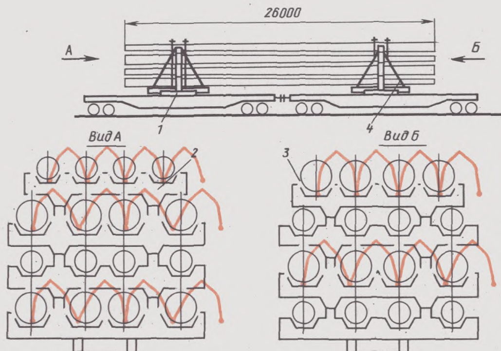
Рис. 10.26: 1—турникет; 2—бандаж; 3—обвязка; 4—растяжка
