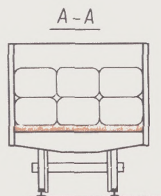
Рис. 3.13: 1—торцовое ограждение; 2—подкладки; 3—поперечная обвязка
