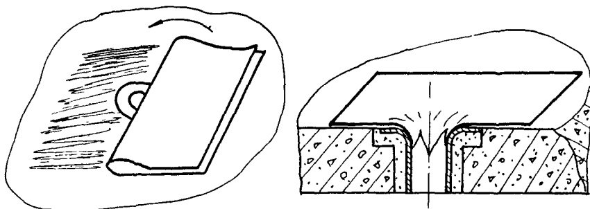
Рис. 3. Оклейка водоприемной воронки дополнительным слоем полимерного материала:
