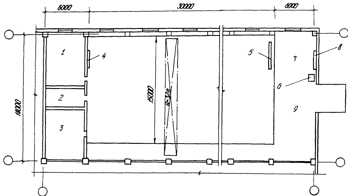
Рис. I. План цеха для склейки ковров кровли:
