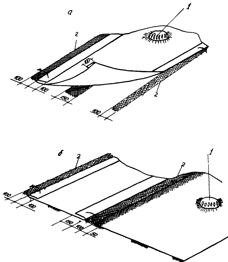
Рис. 6. Полосовая наклейка полотнищ основного гидроизоляционного ковра: 1 - водоприемная воронка; 2 - мастичный слой; а - наклейка первого рулона; б - наклейка второго и последующих рулонов
