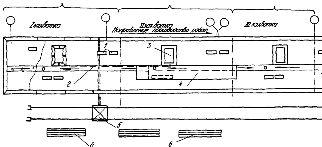
Рис. 6. Схема организации работ на кровле:
