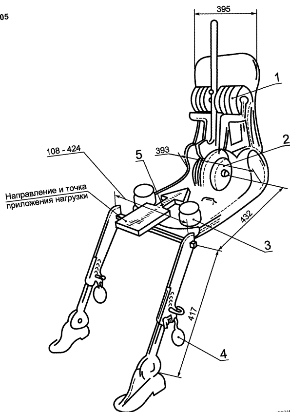
1 — спинные грузы; 2 — сидалищные грузы; 3 — набедренные грузы; 4 — ножные грузы Рисунок С.2 — Размеры элементов механизма 3-D Н и распределение грузов
