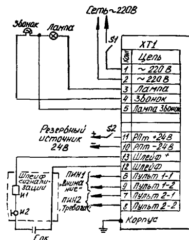
Схема электрическая соединений прибора И1, И2 - извещатели, С ок - оконечный конденсатор
