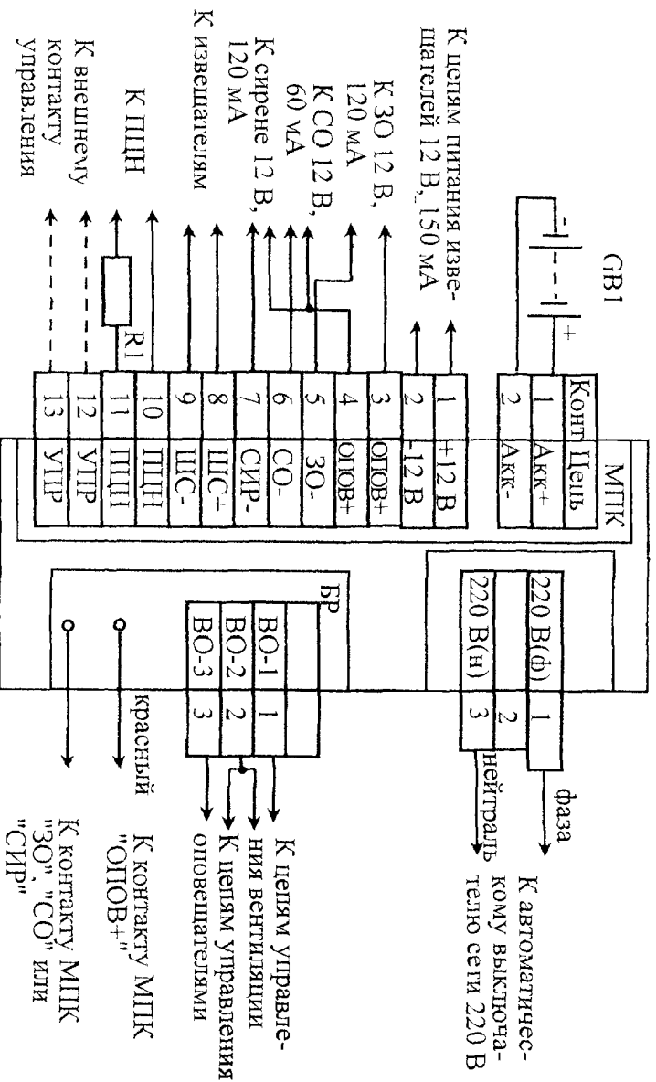
СХЕМА ВНЕШНИХ ПОДКЛЮЧЕНИИ ППКП «НОТА» (ВАРИАНТ 2.00 И 2.01)
