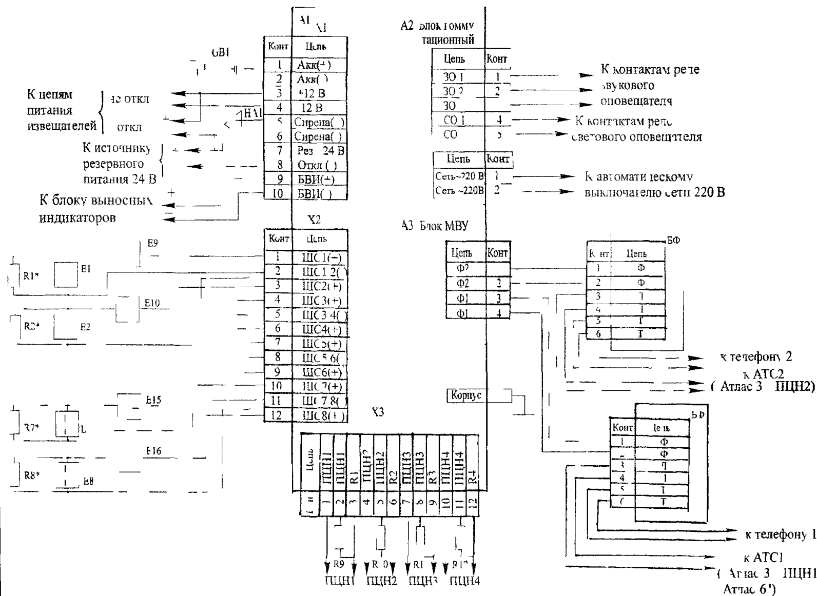
СХЕМА ВНЕШНИХ ПОДКЛЮЧЕНИЙ ПКОП АККОРД (ВАРИАНТ С РАСШИРЕНИЕМ)
