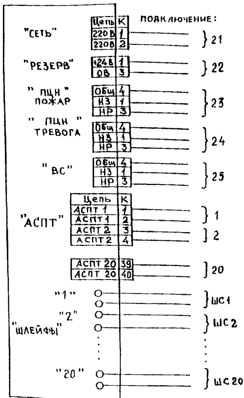
Рис. 52 Схема включения прибора 1, 2 20—на системы пожаротушения и дымоудаления, 21—частота 50 Гц, 220 В, 22—резервное питание 24 В, 23—на ПЦН извещение Пожар, 24—на ПЦН извещение Тревога, 25—на выносную сигнализацию
