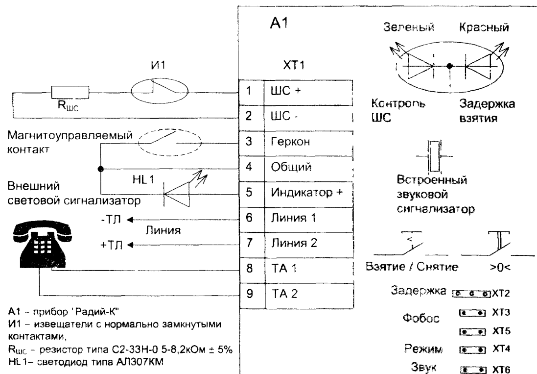
Схема электрическая подключения устройства «Радий-К» при эксплуатации
