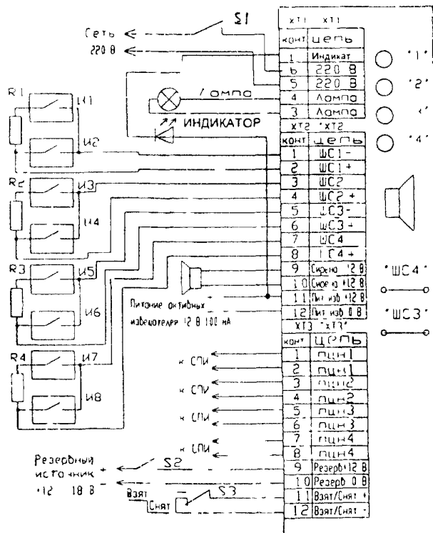
Схема электрическая соединений прибора А1
