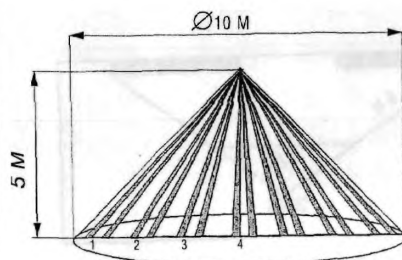
Схема зоны обнаружения в вертикальной плоскости (ИК-канал)
