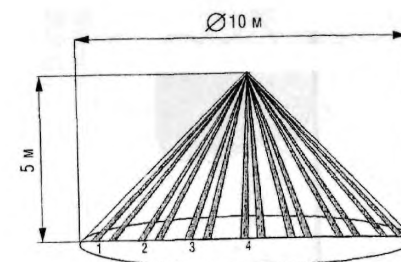
Схема обнаружения в вертикальной плоскости
