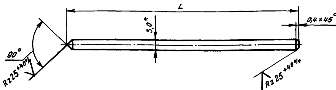
Размеры, мм
