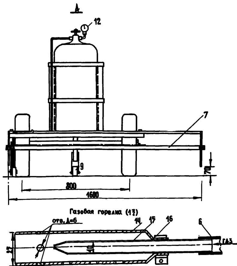
Рис.12. Схема установки для соединения полотен синтетических материалов:
