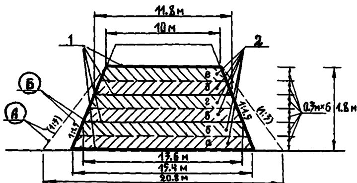
Рис.9. Поперечный профиль насыпи, отсыпаемой из переувлажненных грунтов: А-вариант без оттиба синтетического материала на откос; Б-вариант с оттибом; I-синтетический материал; 2-грунт,отсыпaeмый слоями 0,3м; а-е - слои грунта в порядке их отсыпки
