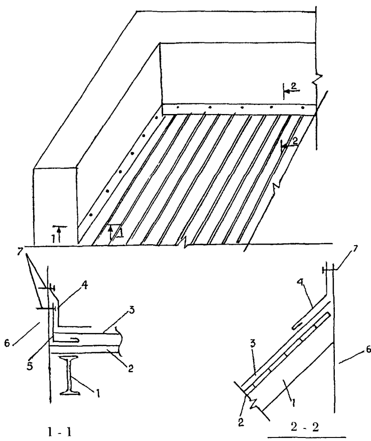
Рис. 12. Места примыкания к стенам и парапетам по уклону и горизонтали: 1 - стропила; 2 - обрешетка; 3 - водонепроницаемый ковер; 4 - фартук; 5 - дополнительный слой; 6 - стена; 7 - дюбель)
