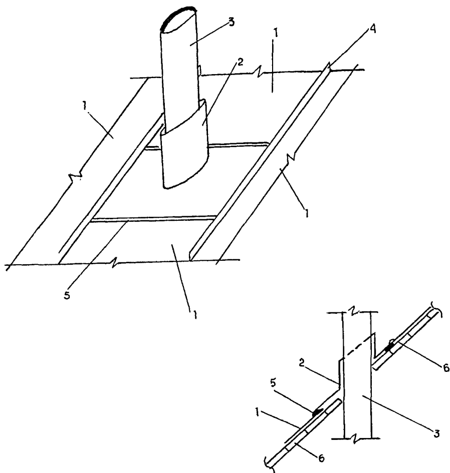
Рис. 15. Место примыкания водонизоляционного ковра к технологическим трубопроводам: 1 - водонизоляционный ковер; 2 - фасонная деталь из металла; 3 - технологический трубопровод; 4 - стоячий фальц; 5 - лежачий фальц; 6 - обрешетка
