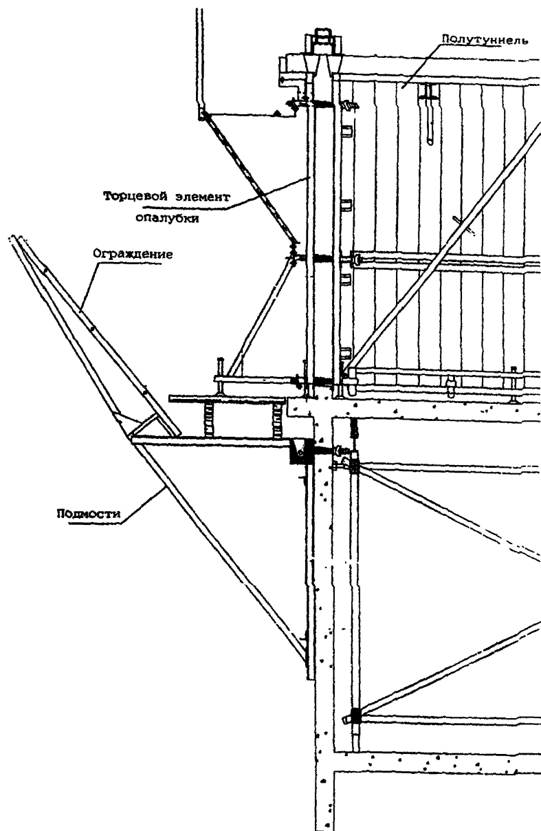
Разрез 2-2
