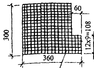
Сетка С1
