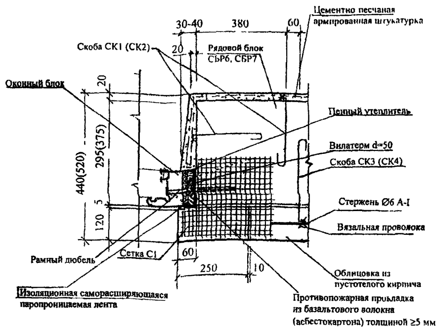
Сетка С1
