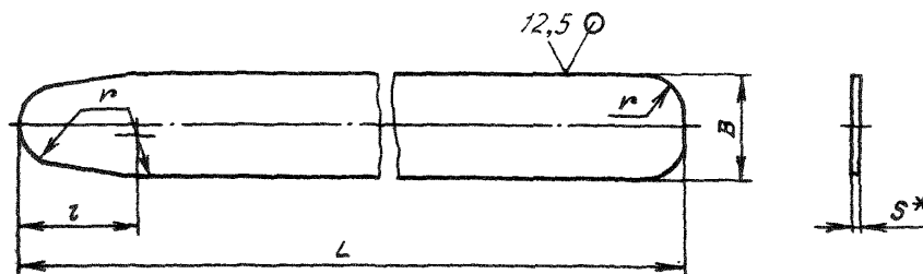
Размеры, мм
