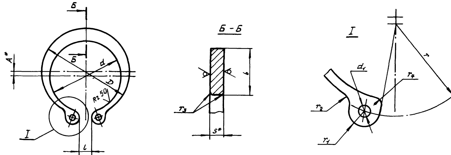
Размеры, мм
