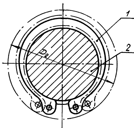
Черт. 2
