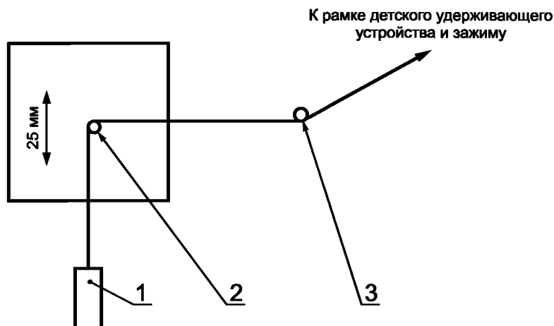
1 — груз; 2 — промежуточный ролик; 3 — направляющий ролик
