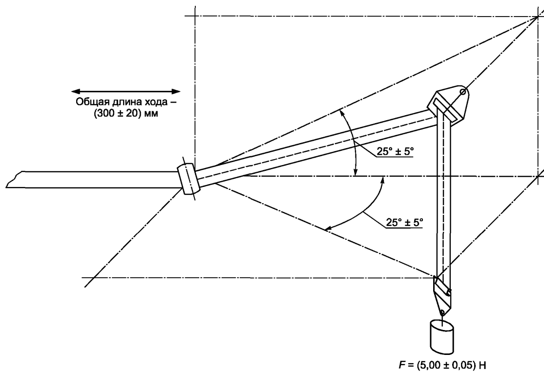
Рисунок Д.4 — Испытание с направляющим устройством
