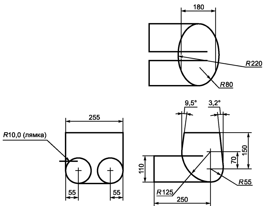
Рисунок Ш.1 — Манекен Р10 в разрезе
