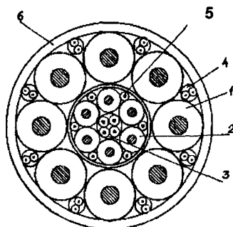
Рис 2 Схема коаксиального кабеля комбинированной конструкции 1 - коаксиальная пара 2,6/9,4, 2 - коаксиальная пара 1,2/4,6, 3 - симметричная четверка, 4 - симметричная пара, 5 - одиночная жила, 6 - оболочка
