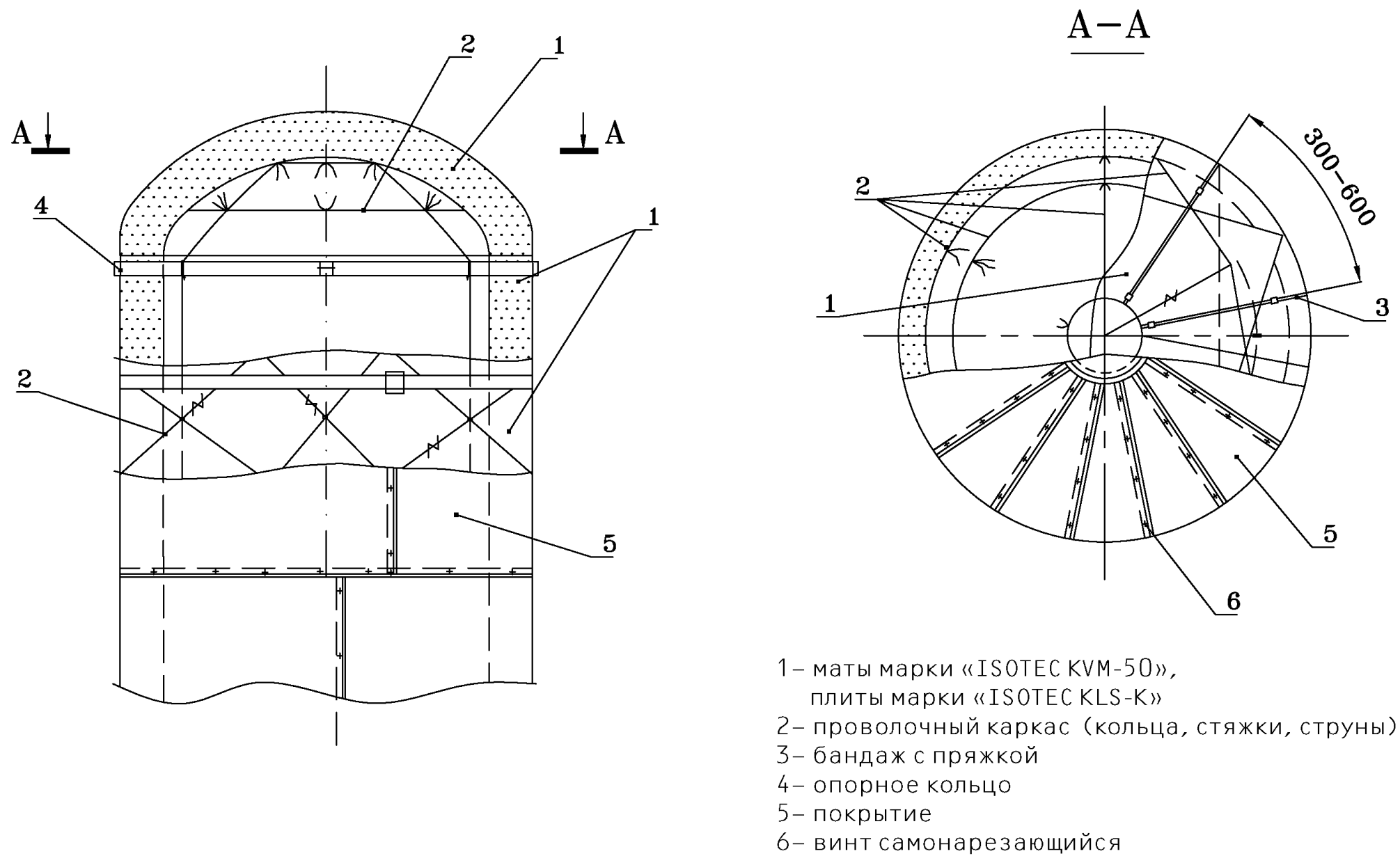
Рис. 16. Изоляция вертикальных аппаратов матами марки «ISOTEC KVM-50» или плитами марки «KLS-K» с креплением бандажами и стяжками с металлическим покрытием
