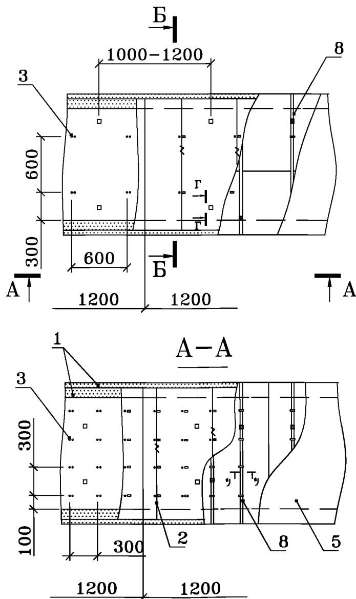
Рис. 25. Конструкция тепловой изоляции на основе плит марки "ISOTEC KLS-K" для горизонтальных газоходов прямоугольного сечения с положительными температурами
