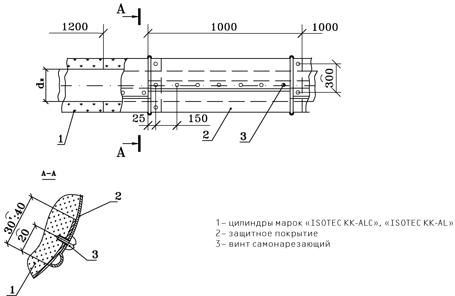
Рис. 3. Конструкция тепловой изоляции трубопроводов цилиндрами марок «ISOTEC KK-ALC», «ISOTEC KK-AL» с креплением защитного покрытия винтами
