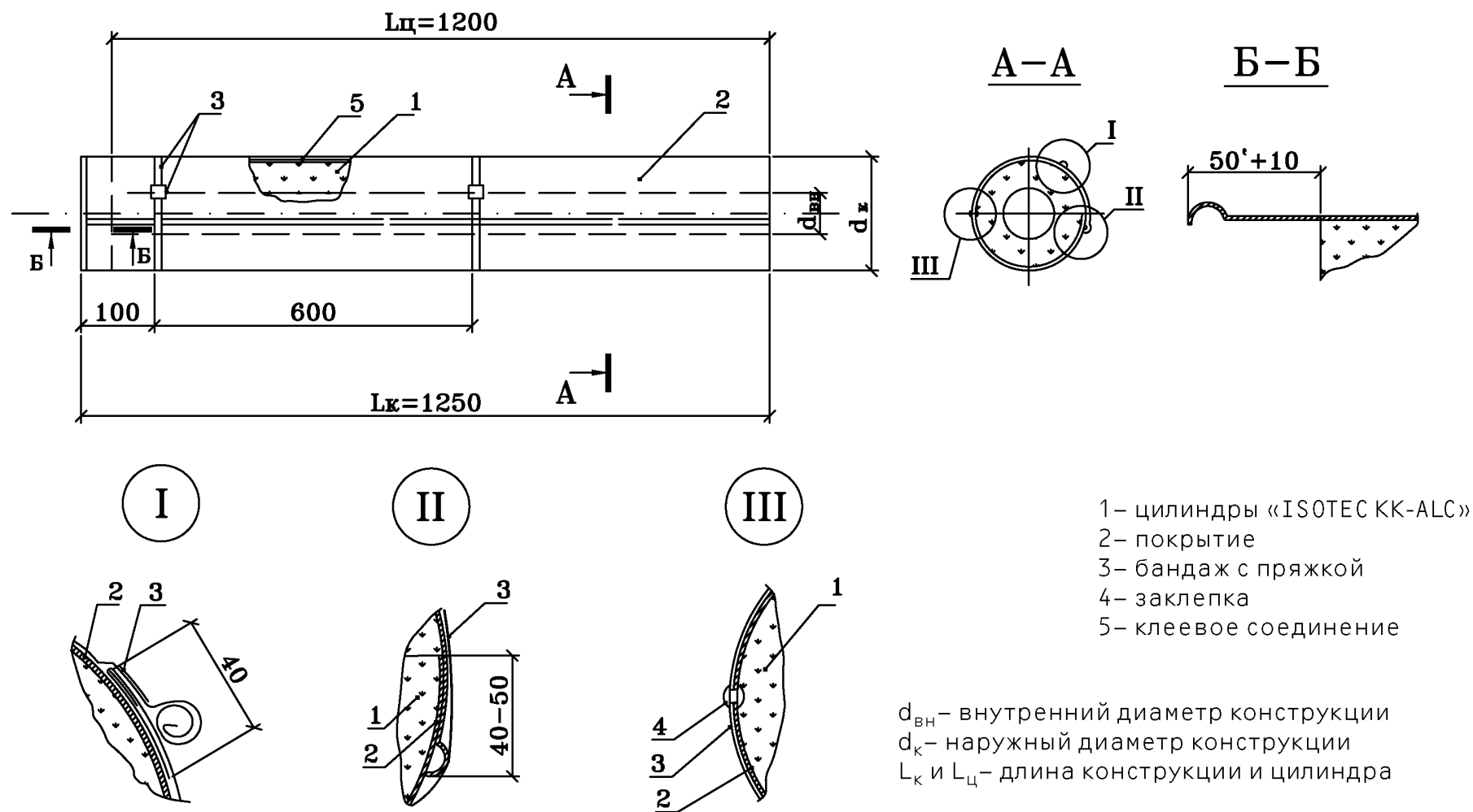
Рис. 8. Конструкция теплоизоляционная сборная на основе цилиндров марки «ISOTEC KK» с металлическим защитным покрытием и креплением бандажами
