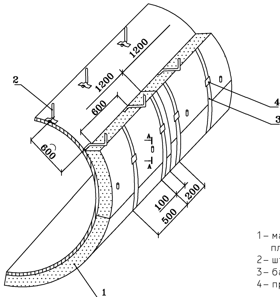
Рис. 18. Изоляция горизонтальных аппаратов матами марки «ISOTEC KVM-50» или плитами марки «KLS-K» в один слой с креплением штырями
