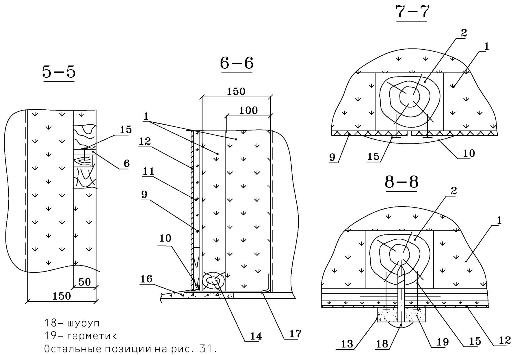
Рис. 33. Разрезы 5-5 – 8-8 к рис. 31.
