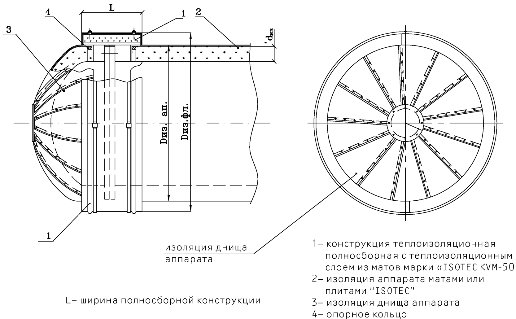
Рис. 21. Изоляция фланцевого соединения горизонтального аппарата конструкциями теплоизоляционными полносборными с теплоизоляционным слоем из матов марки «ISOTEC KVM-50»
