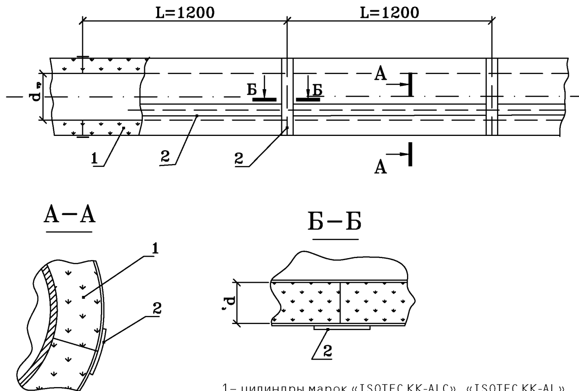
Рис. 1. Изоляция трубопроводов диаметром до 140 мм включительно цилиндрами марок «ISOTEC KK-ALC», «ISOTEC KK-AL» с облицовкой паронепроницаемой алюминиевой фольгой
