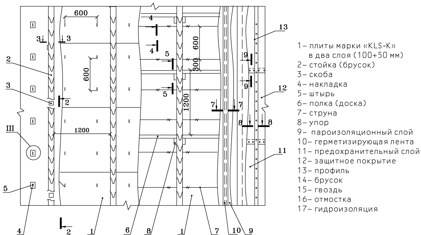
Рис. 31. Узел I к рис. 30. Конструкция изоляции на основе плит марки «ISOTEC KLS-K» для цилиндрической стенки резервуара холодной воды
