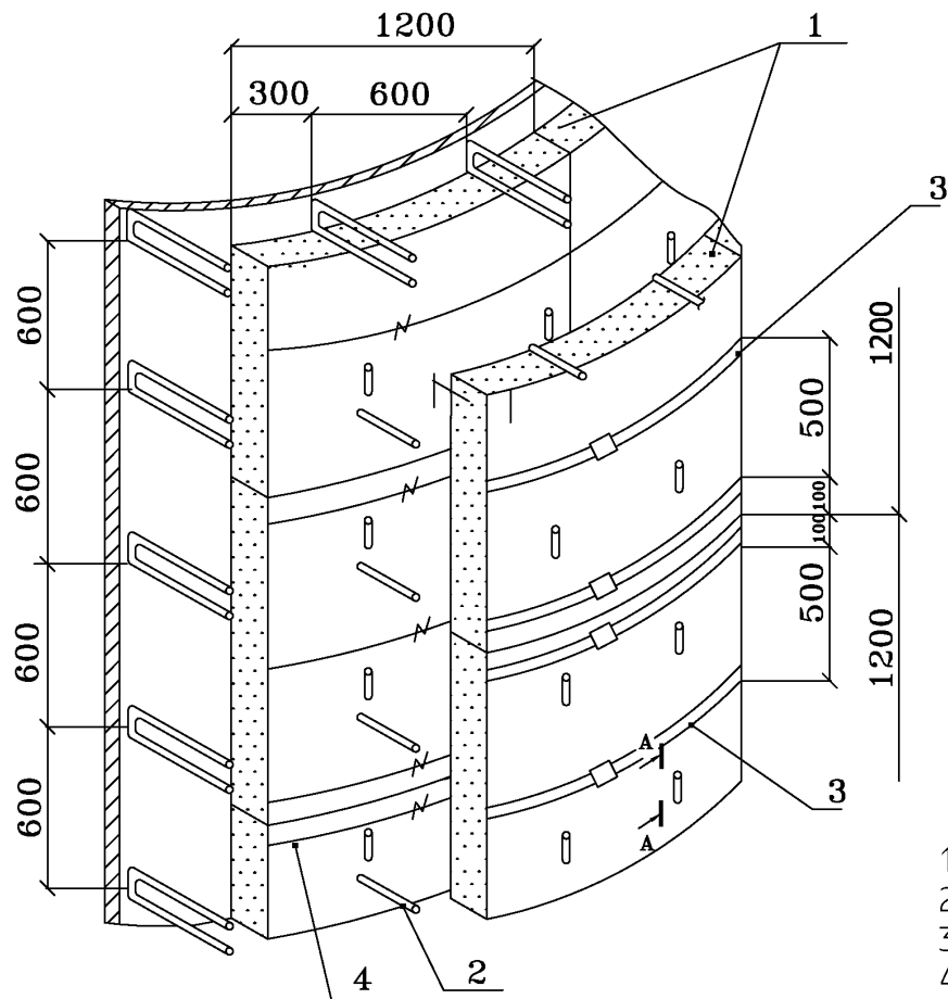
Рис. 19. Изоляция вертикальных аппаратов матами марки «ISOTEC KLS-K» в два слоя с креплением штырями
