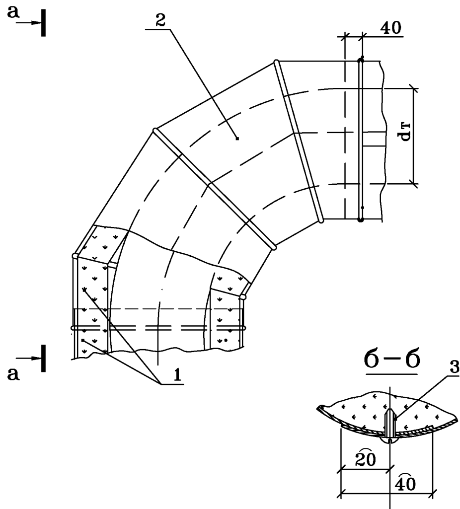
Рис. 4. Конструкция отвода трубопровода из цилиндров марок «ISOTEC KK-ALC», «ISOTEC KK-AL» с покрытием металлическим отводом
