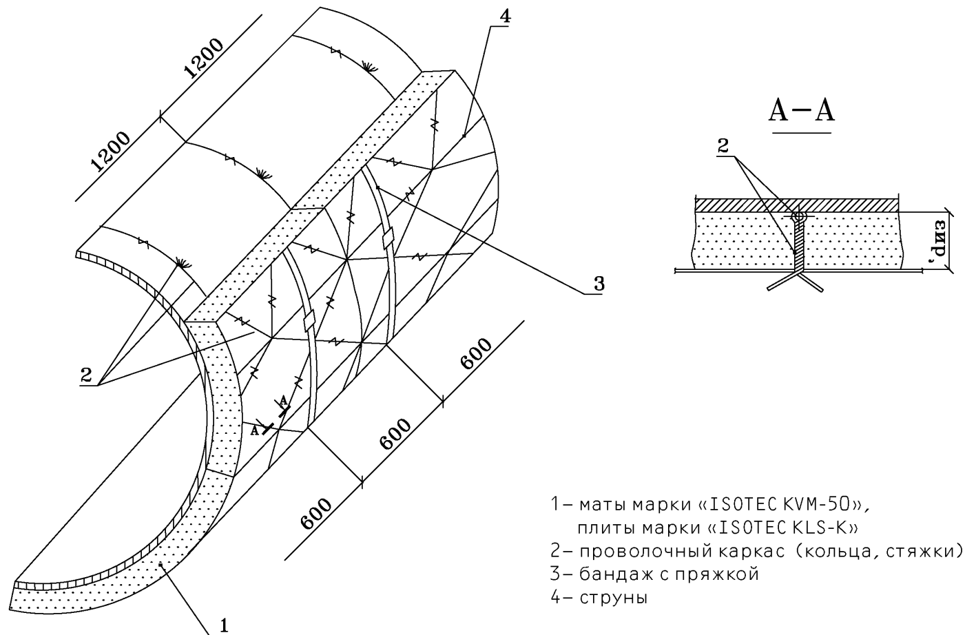
Рис. 17. Изоляция горизонтальных аппаратов матами марки «ISOTEC KVM-50» или плитами марки «KLS-K» в один слой с креплением на проволоочном каркасе
