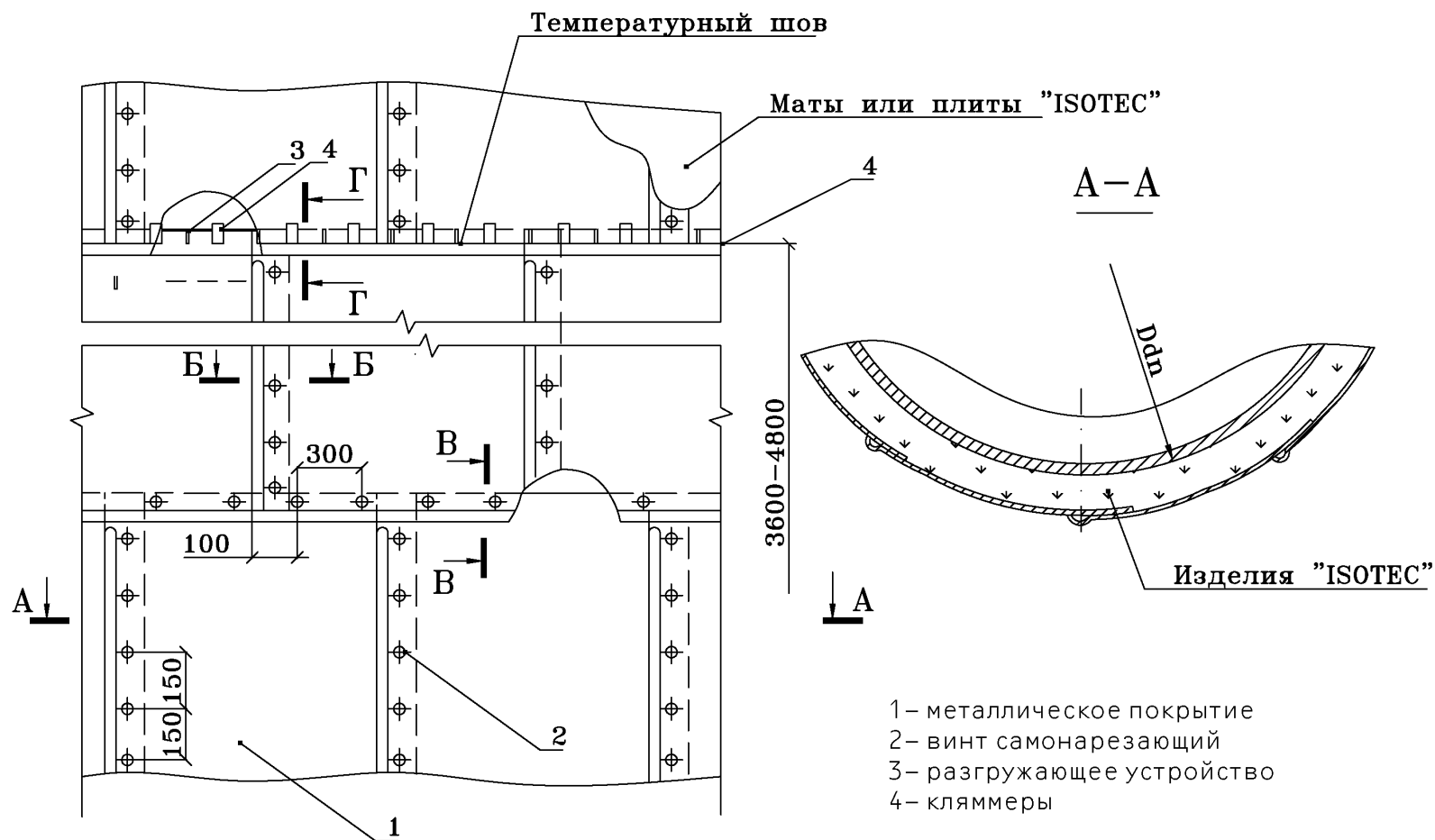
Рис. 23. Конструкция металлического покрытия тепловой изоляции для вертикальных аппаратов и резервуаров
