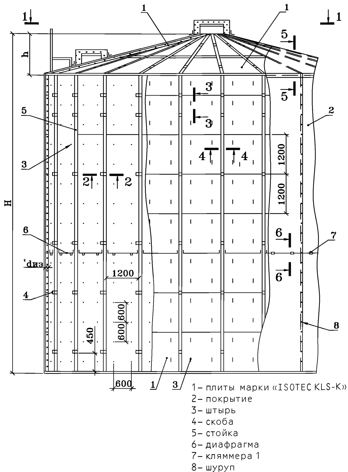
Рис. 27. Конструкция тепловой изоляции на основе плит марки «ISOTEC KLS-K» для резервуара для хранения нефти и нефтепродуктов температурой не выше 80 °С
