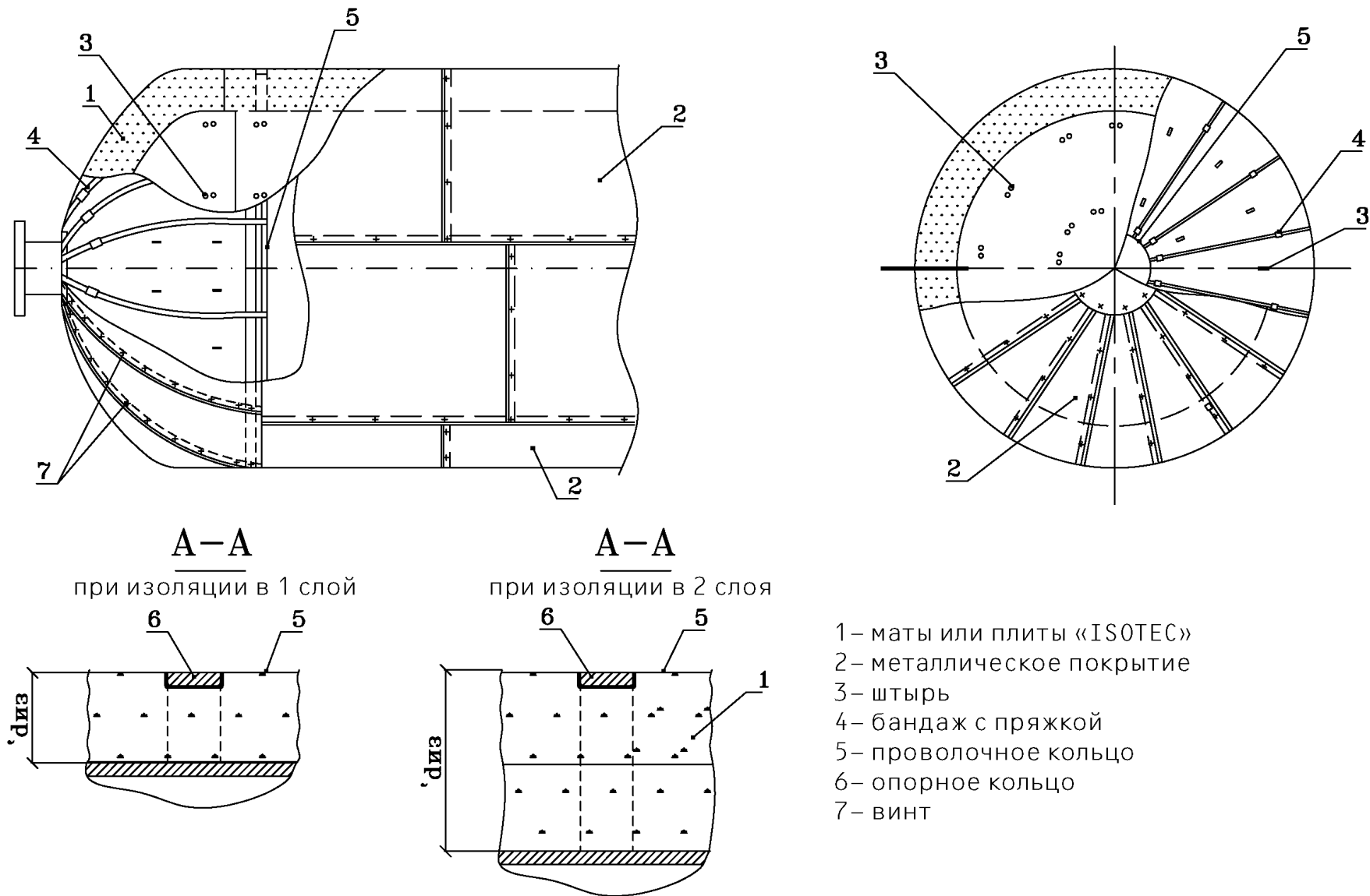
Рис. 20. Изоляция днищ горизонтальных аппаратов матами или плитами «ISOTEC» с креплением штырями и с металлическим защитным покрытием
