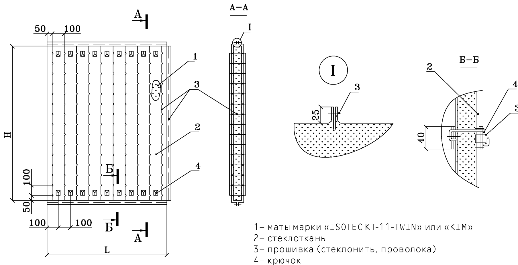
Рис. 15. Матрац с теплоизоляционным слоем из матов «ISOTEC»
