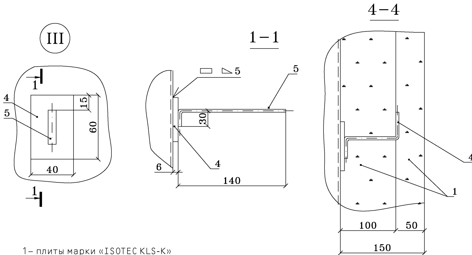
Рис. 32. Узел III и разрезы 1-1 и 4-4 к рис. 31.
