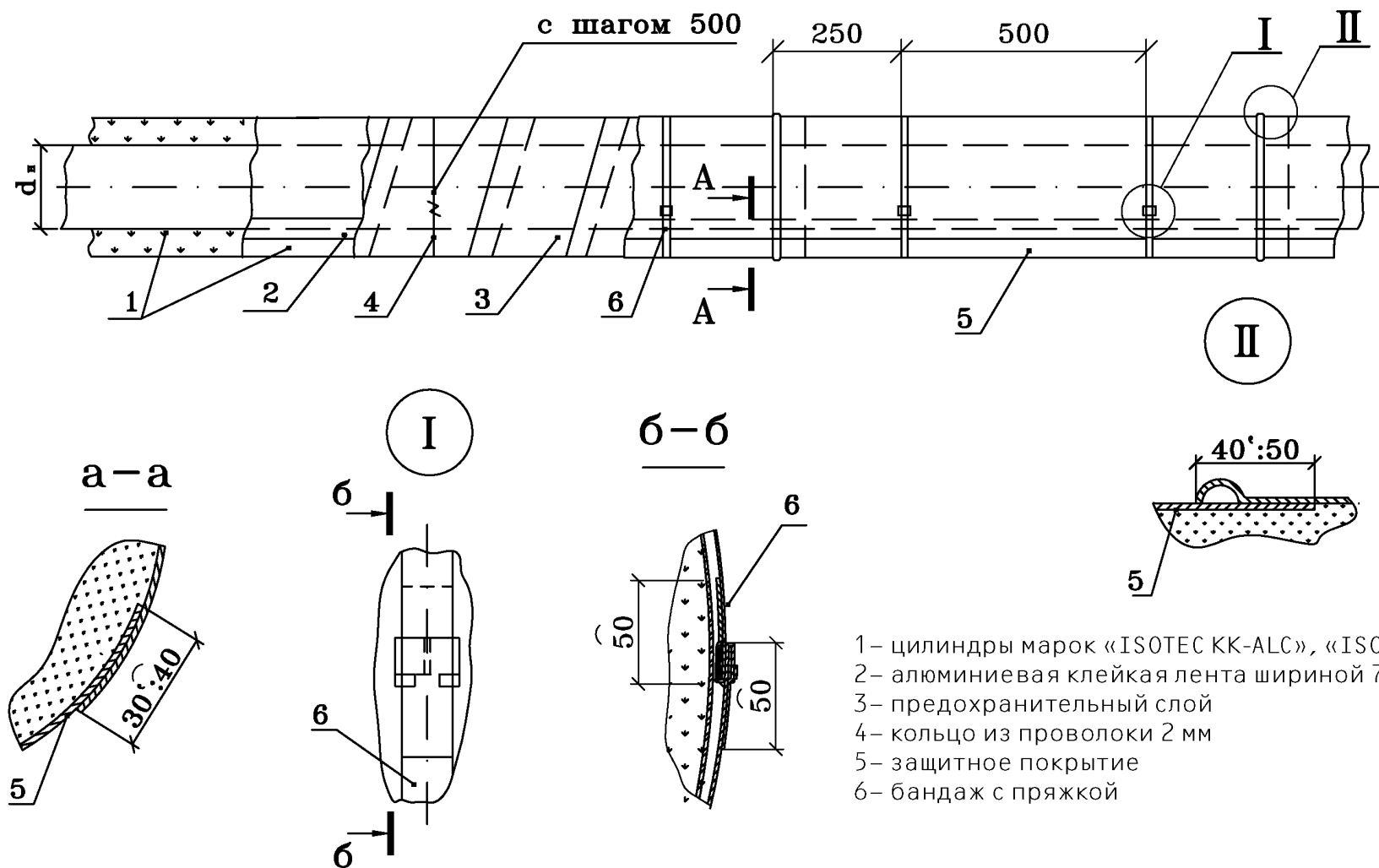
Рис. 2. Конструкция тепловой изоляции трубопроводов цилиндрами марок «ISOTEC KK-ALC», «ISOTEC KK-AL» с креплением металлического защитного покрытия бандажами
