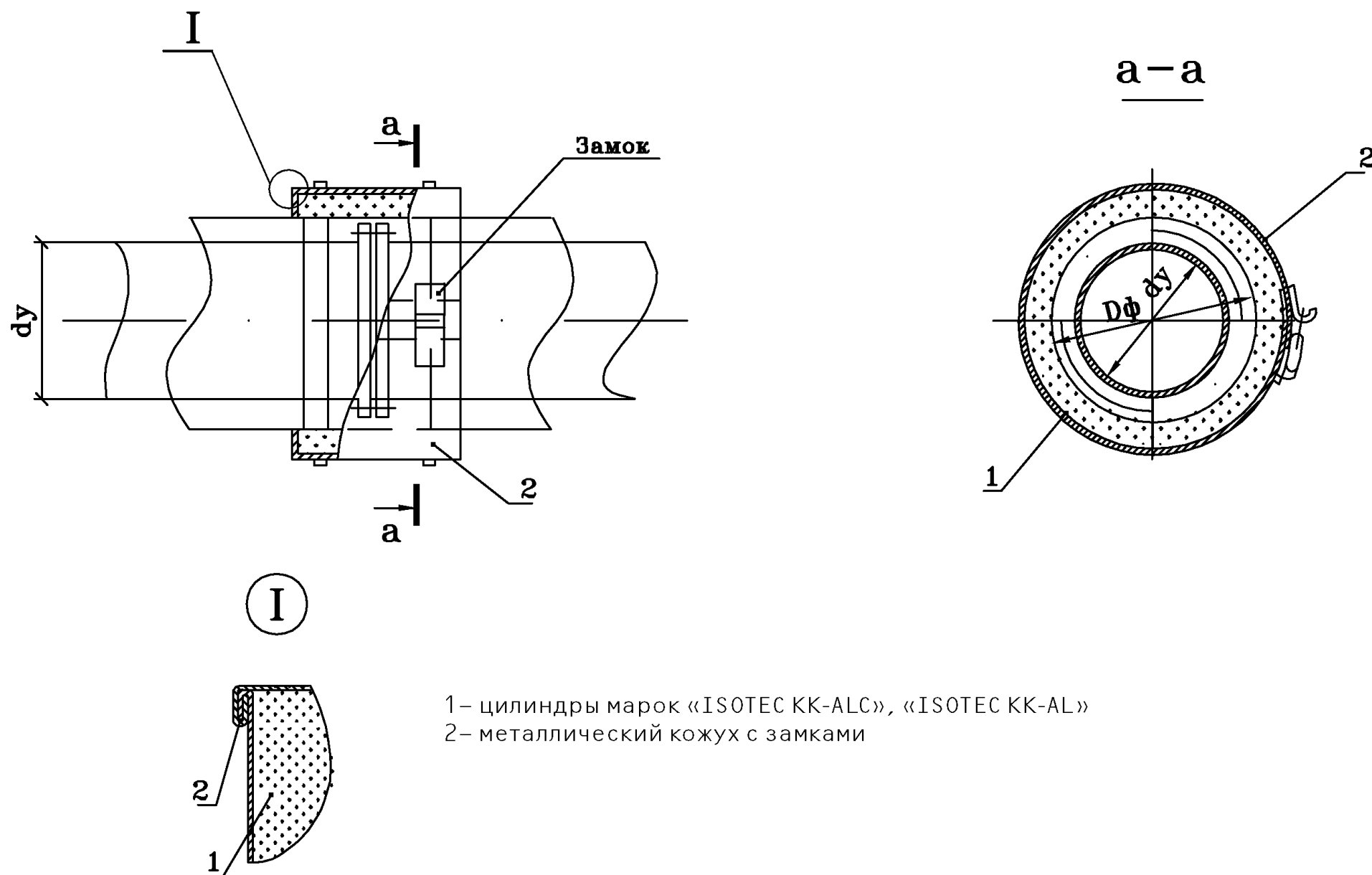
Рис. 6. Изоляция фланцевого соединения цилиндрами марок «ISOTEC KK-ALC», «ISOTEC KK-AL» со съемным металлическим кожухом с замками
