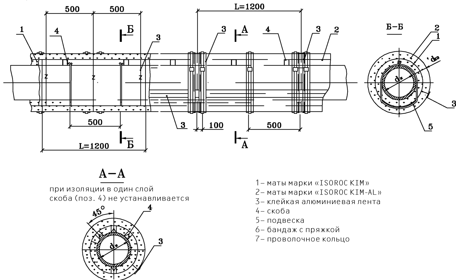
Рис. 10. Изоляция трубопроводов наружным диаметром 219 мм и более матами марок «ISOROC KIM» и «ISOROC KIM-AL»
