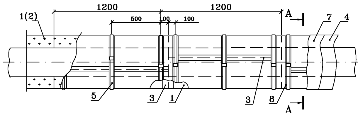
Рис. 9. Изоляция трубопроводов диаметром до 273 мм матами марки «ISOTEC KIM-AL» или трубопроводов диаметром изоляции до 140 мм скорлупами марки «ISOTEC KK-ALC»
