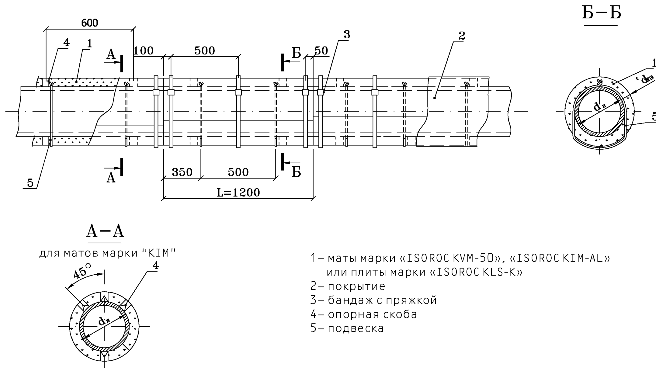
Рис. 11. Изоляция матами и плитами «ISOTEC» в один слой с креплением бандажами и подвесками
