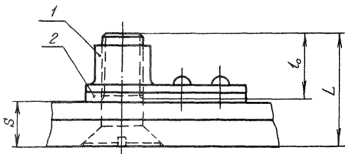
1 - гайка; 2 - шайба
