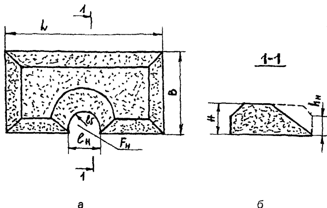
Рисунок К 5 – План бурта
