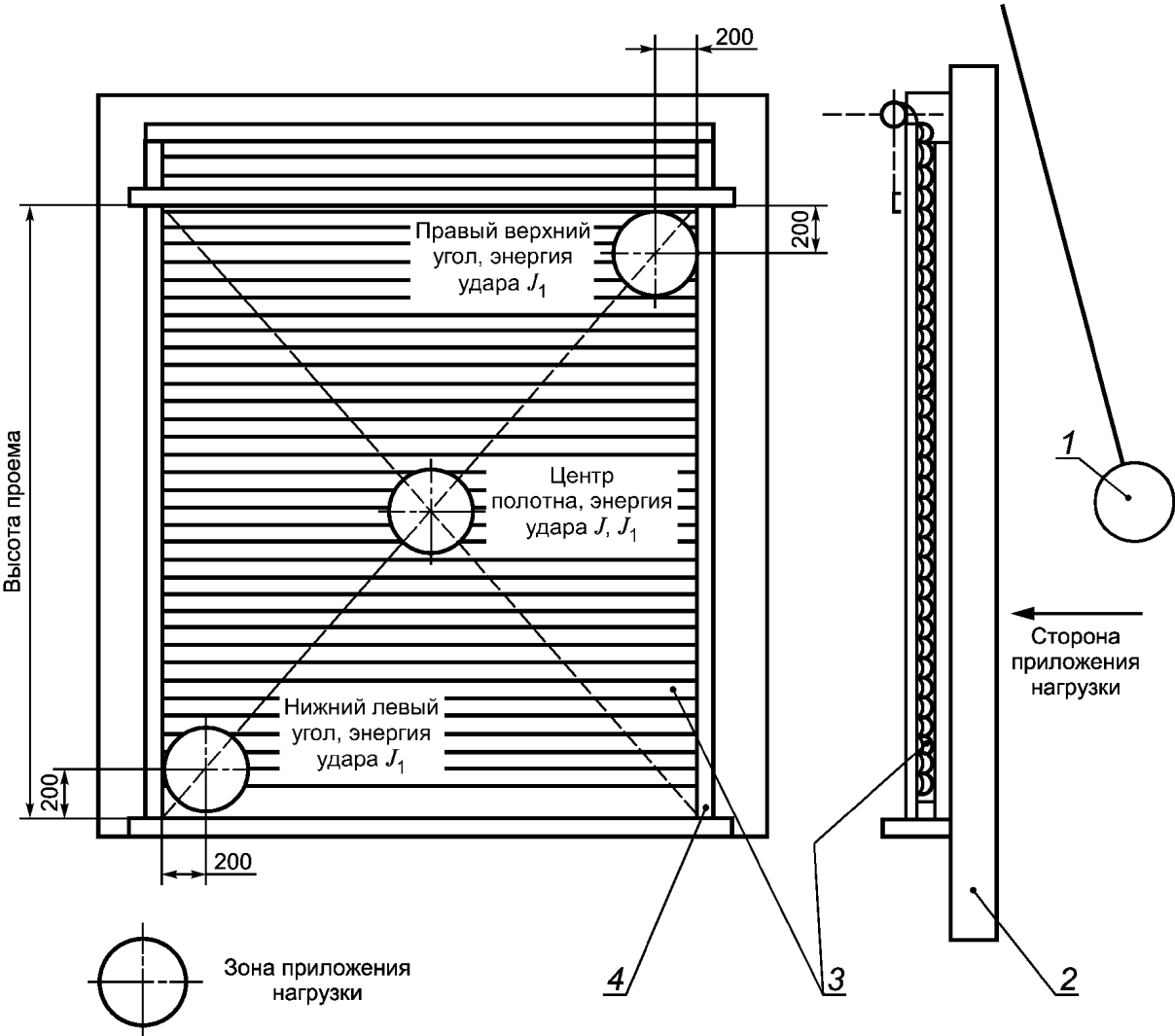
1 — ударный груз; 2 — испытательный стенд; 3 — жалюзи-роллета; 4 — направляющая шина
