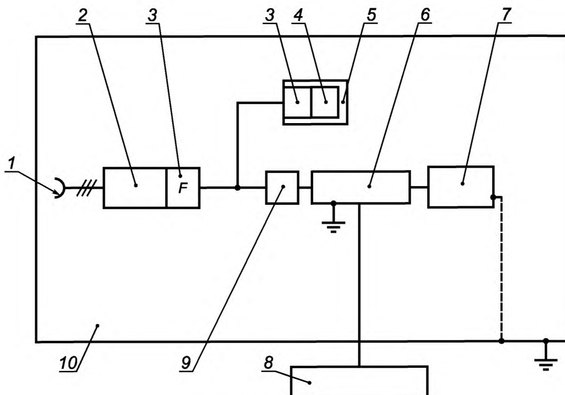
1 — сеть электропитания переменного тока 220 В, 50 Гц; 2 — блок питания; 3 — фильтр; 4 — передатчик/приемник; 5 — блок связи; 6 — устройство связи/развязки; 7 — испытуемое устройство; 8 — генератор сигналов высокой частоты и усилитель; 9 — аттенюатор; 10 — пластина заземления
