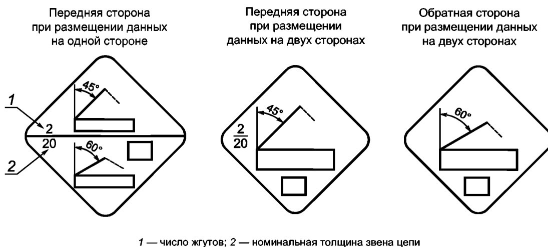
Рисунок D.2 — Ярлыки для маркировки стропальных цепей из нескольких жгутов
