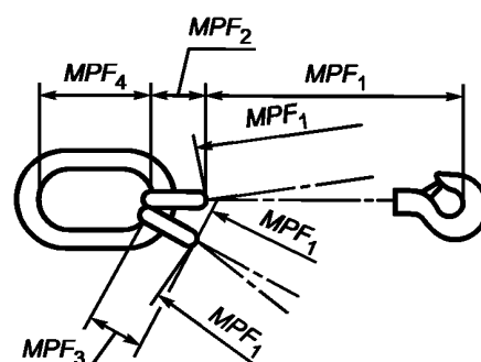
г) Стропальная цепь из четырех жгутов
