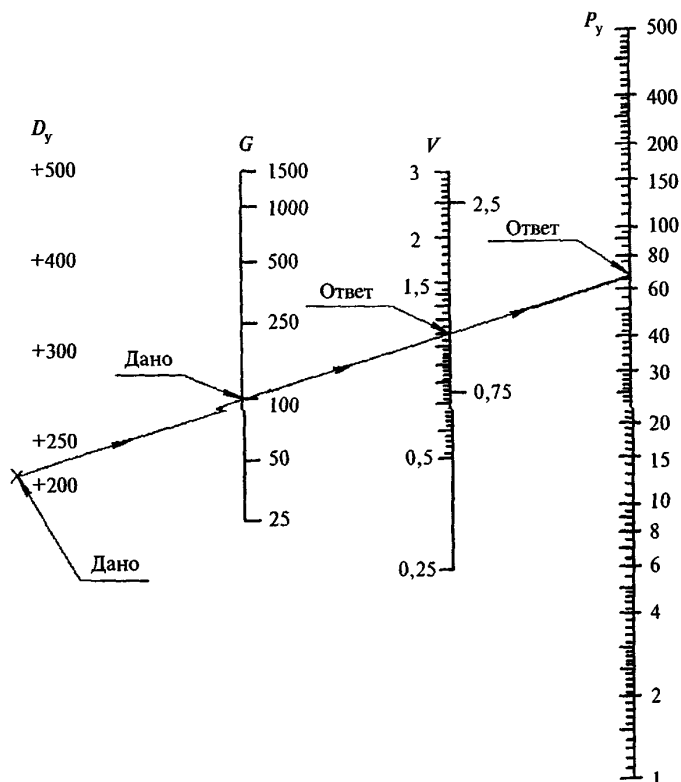
Рисунок 5 — Номограмма для гидравлического расчета трубопроводов из асбестоцементных труб
