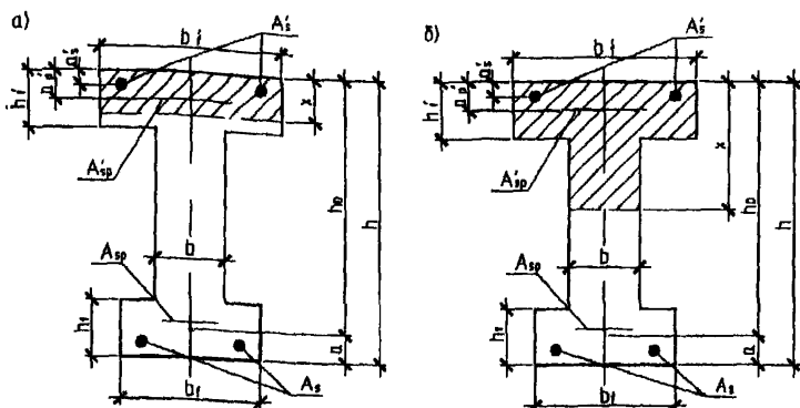
Черт.3.2. Форма сжатой зоны в двутавровом сечении железобетонного элемента
