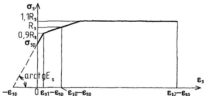
Черт.3.13.Трехлинейная диаграмма состояния арматуры с условным пределом текучести при учете предварительного напряжения (здесь \varepsilon_s - деформация арматуры от внешней нагрузки)
