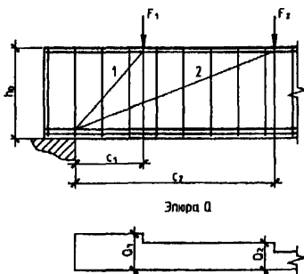
Черт.3.16. Расположение расчетных наклонных сечений при сосредоточенных силах 1 - наклонное сечение, проверяемое на действие поперечной силы Q_i ; 2 - то же, силы Q_2
