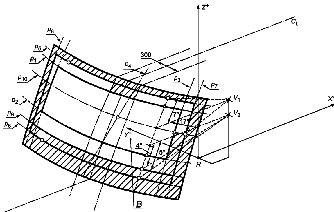
Рисунок 2a — Испытательная зона B, площадь которой сокращена (на примере ТС, предназначенного для левостороннего движения) — верхняя светонепроницаемая поверхность соответствует определению, приведенному в 2.4.2.2
