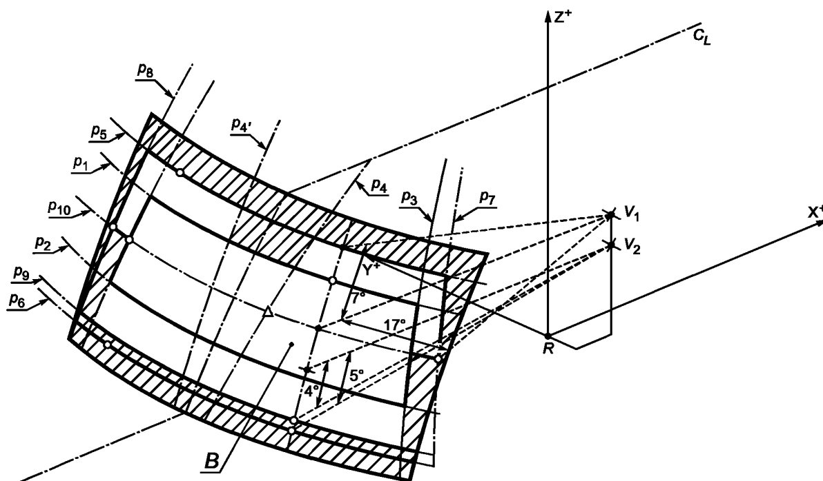
Рисунок 2a — Испытательная зона B, площадь которой сокращена (на примере ТС, предназначенного для левостороннего движения) — верхняя светонепроницаемая поверхность соответствует определению, приведенному в 2.4.2.2
