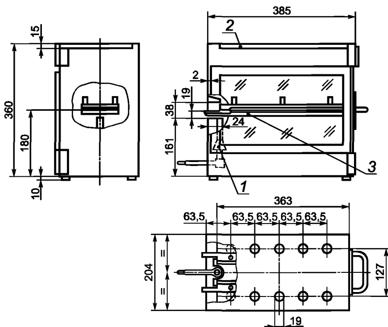
1 — газовая горелка; 2 — вентиляционная щель; 3 — образец для испытаний
