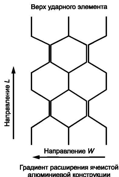
Рисунок 3 — Ориентация ячеистой алюминиевой конструкции
