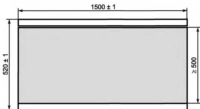
Рисунок 5 — Схема задней панели (вид спереди)
