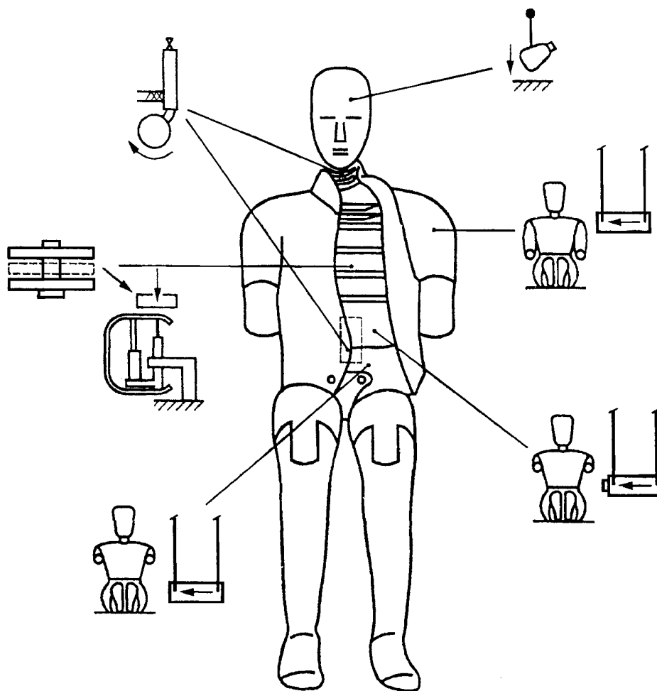
Рисунок 3 — Схема испытаний манекена на боковой удар
