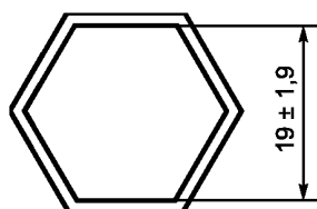
Рисунок 4 — Размер ячеек алюминиевой ячеистой конструкции
