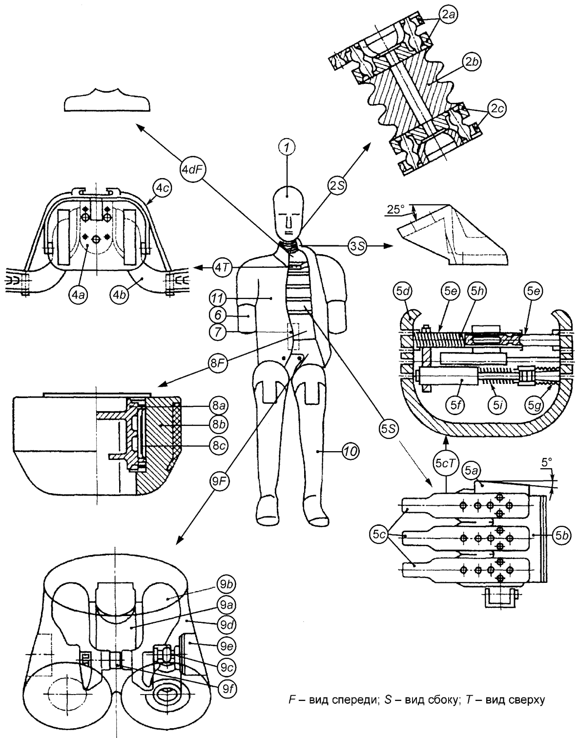
Рисунок 1 — Конструкция манекена для испытания на боковой удар
