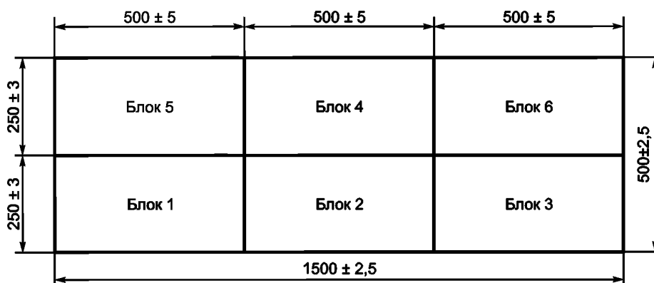
Рисунок 1 — Схема ударного элемента 1)
