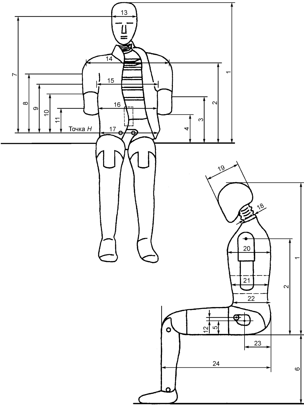
Рисунок 2 — Основные размеры манекена (см. таблицу 5.3)
