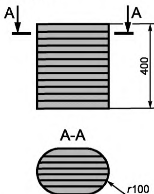
Рисунок 3 — Ударный элемент, моделирующий туловище
