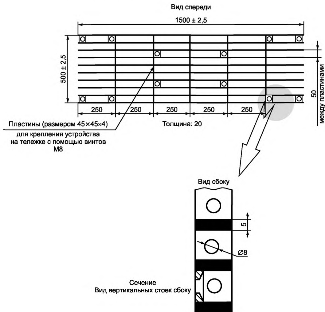
Рисунок 9 — Вентиляционная решетка
