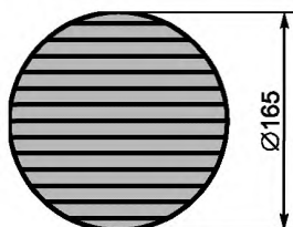
Рисунок 2 — Ударный элемент, моделирующий голову
