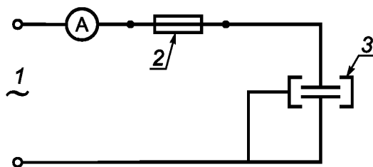
1 — источник переменного напряжения; 2 — плавкий предохранитель; 3 — конденсатор
