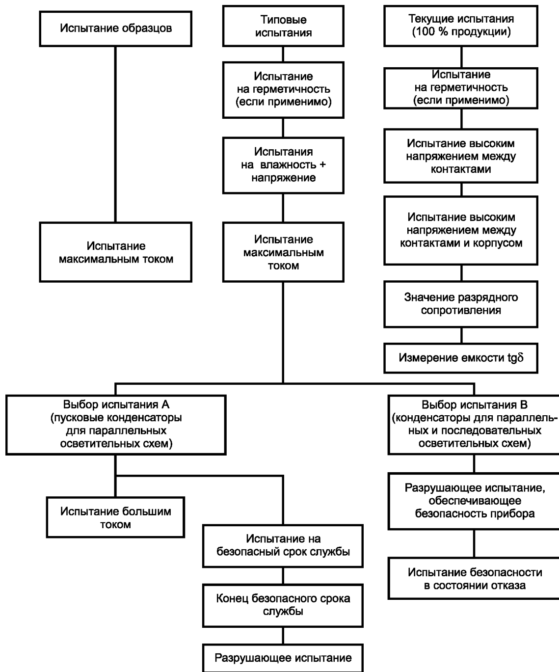
Рисунок 4— Схема процедуры испытаний
