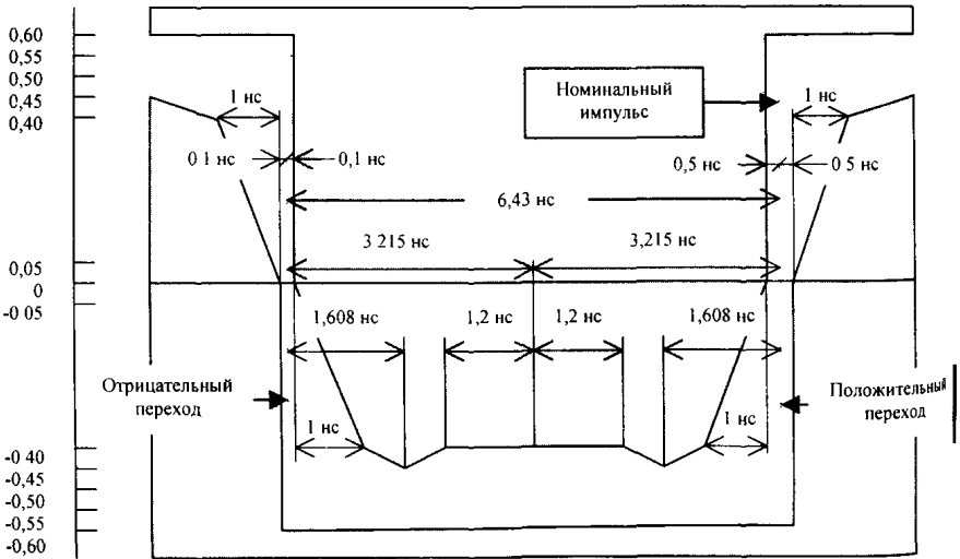
Рис.8. Маска импульса, соответствующая 1, на стыке 155,520 Мбит/с.
