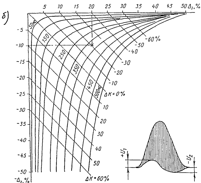
Рисунок 9 – кривые для определения P_{25} , когда сигнал яркости опережает сигнал цветности: а – для малых \Delta_1 и \Delta_2 ; б – для больших \Delta_1 и \Delta_2
