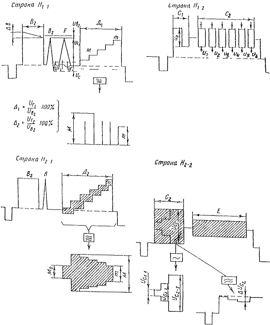
Рисунок 7 – измерения, проводимые с помощью сигналов испытательных строк
