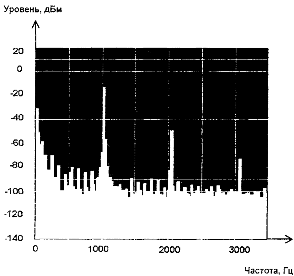
Рисунок 10 - Спектральная характеристика сигнала частотой 1020 Гц при при наличии нелинейных искажений
