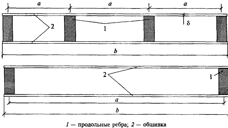
Рисунок 3 — Поперечное сечение клееных плит из фанеры и древесины
