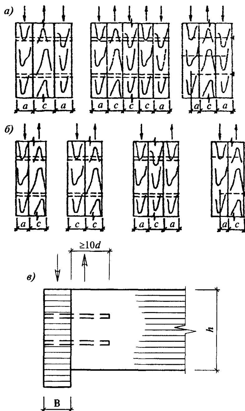
Рисунок 8 — Нагельные соединения
