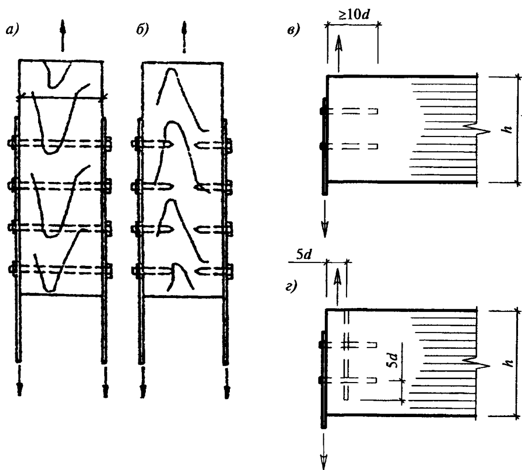
a — на болтах; б — на глухих цилиндрических нагелях; в — на глухих цилиндрических нагелях, установленных в торец клееного элемента; г — то же, с усилением поперечным армированием
