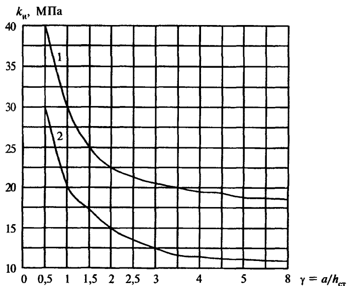
Рисунок Д.2 — Графики для определения коэффициента k_n при расположении волокон в наружных слоях фанеры вдоль пролета
