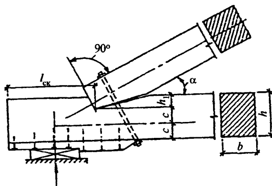
Рисунок 7 — Лобовая врубка с одним зубом
