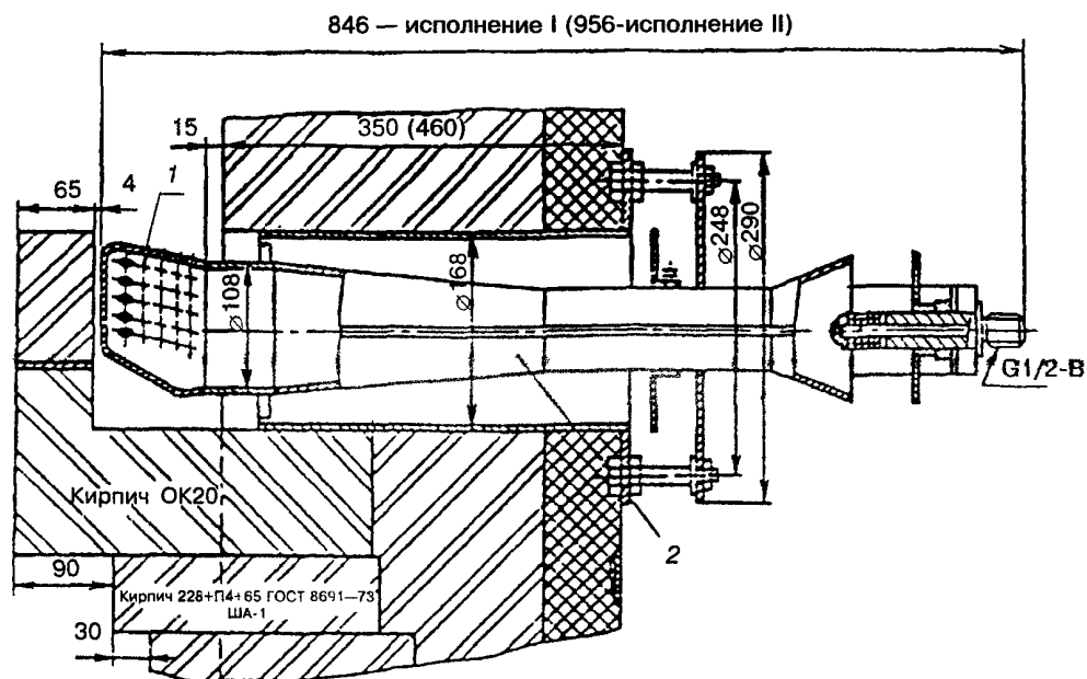
Горелка ГВН-0,35
